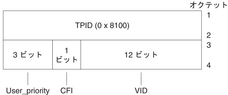
図 2-1 Ethernet タグヘッダーの形式
