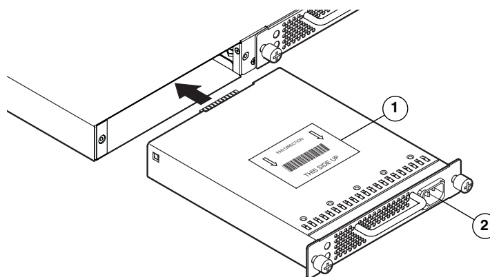
1. 部品番号ラベル
