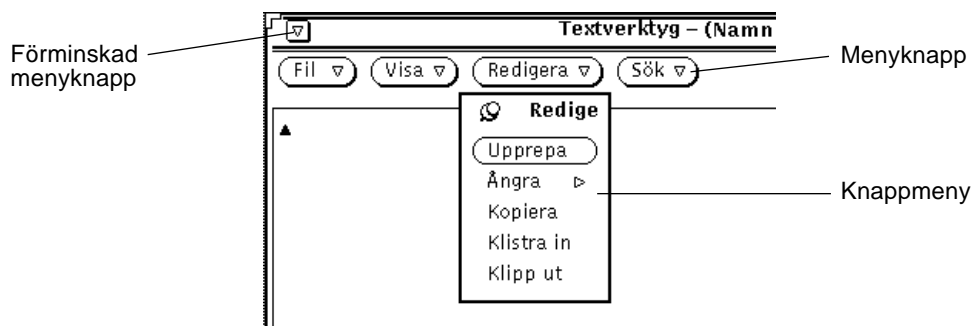
Figur 1-19 Textverktygets menyknappar
