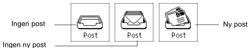
Figur 4-1 Postverktygets ikoner
