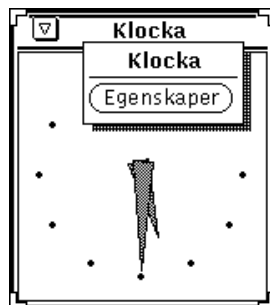
Figur 7-3 Snabbmenyn Klocka
