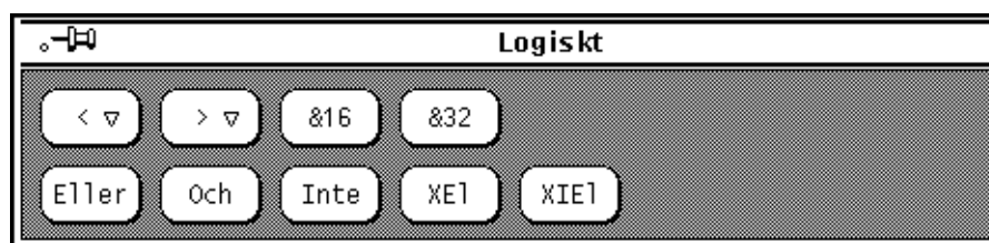
Figur 8-12 Logiska funktioner
