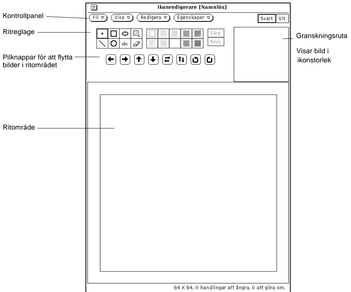
Figur 15-2 Ikonredigerarens grundfönster
