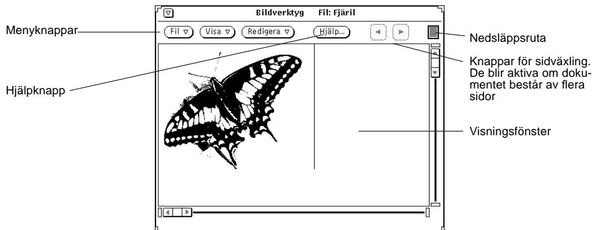
Figur 13-2 Bildverktygets grundfönster
