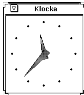
Figur 7-2 Klockans fönster
