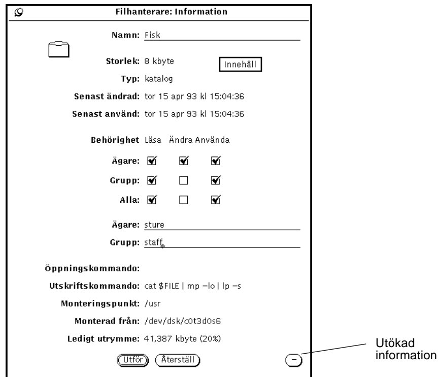
Figur 2-32 Fönstret Information
