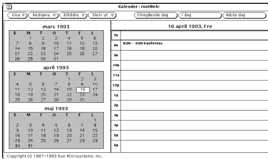
Figur 5-4 Dagskalender
