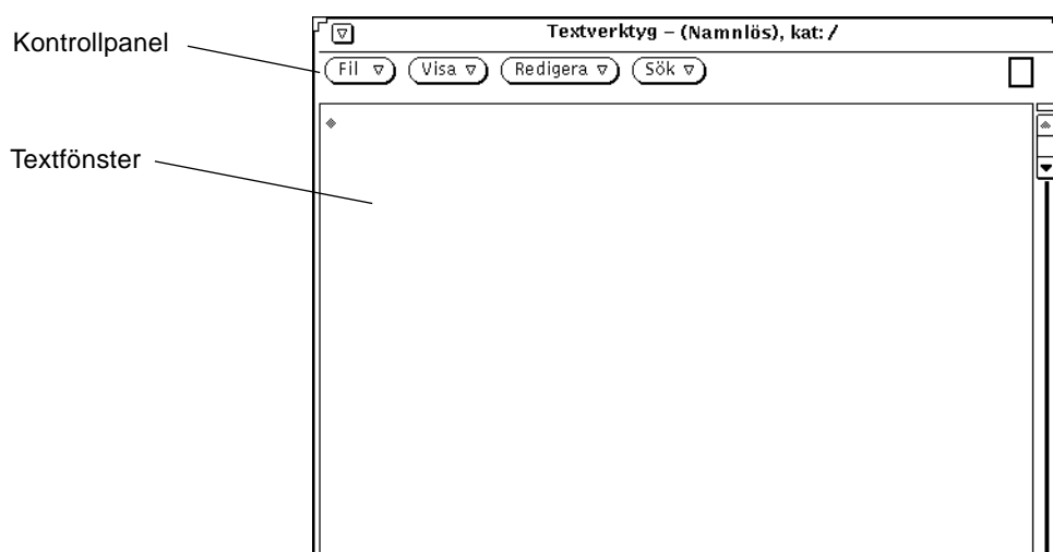
Figur 3-2 Textverktygets grundfönster
