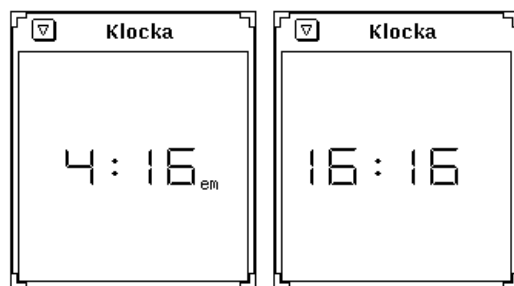
Figur 7-7 12- och 24-timmarsklocka
