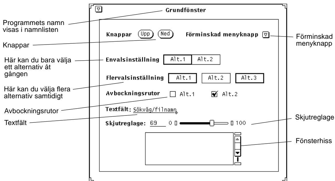
Figur 1-17 Fönsterreglage
