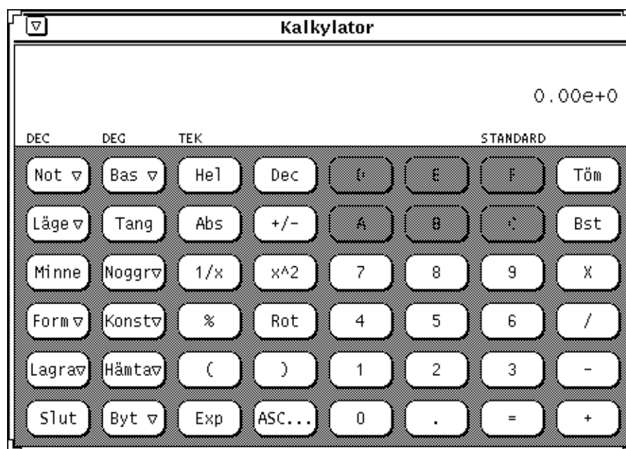
Figur 8-15 Högerhänt kalkylator
