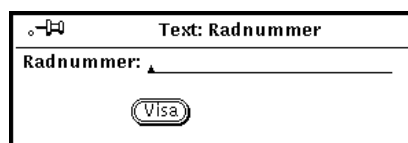
Figur 3-3 Snabbfönstret Radnummer
