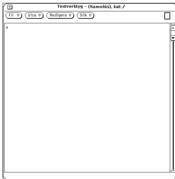
Figur 1-33 Textverktøgets fönster
