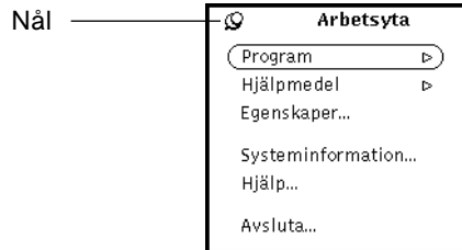
Figur 1-12 Menyn Arbetsyta
