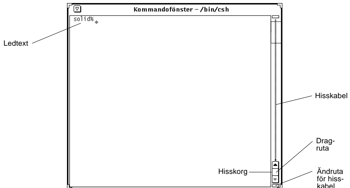
Figur 1-18 Kommandofönstrets fönsterhiss
