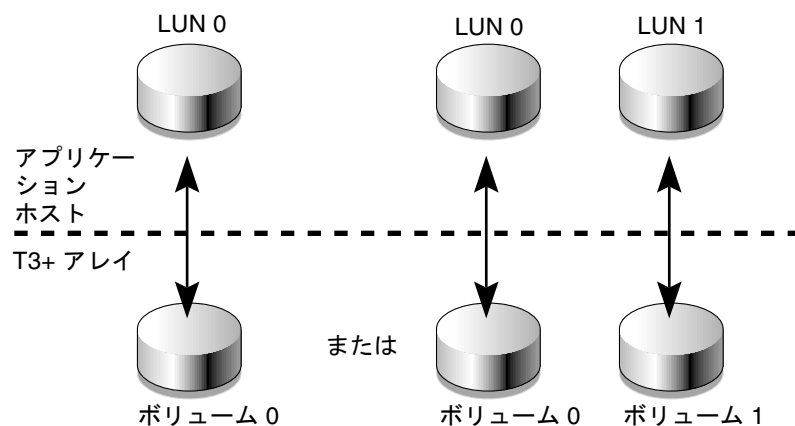
図 2-1 コントローラファームウェアバージョン 2.0.1 が搭載されている単一の T3+ アレイで構成できる 2 種類のマッピング
