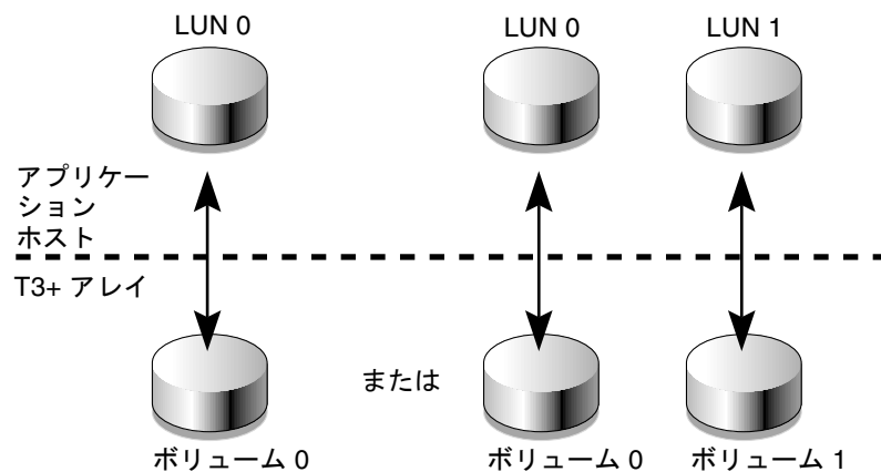
図 2-2 コントローラファームウェアバージョン 2.1 が搭載されている単一の T3+ アレイで構成できる 2 種類のマッピング
