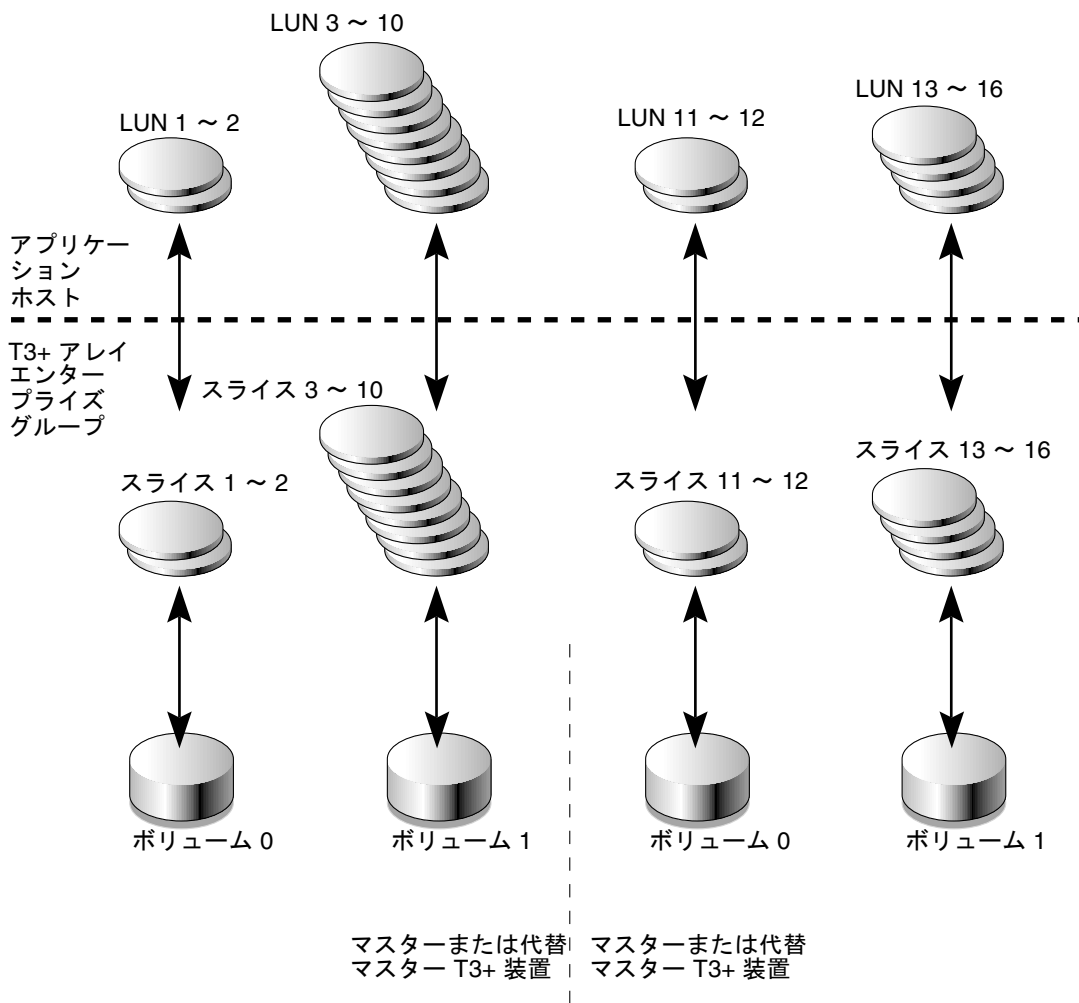
図 2-4 2つのボリュームを持ちコントローラファームウェアバージョン 2.1が搭載されてボリュームのスライシングが可能になっている T3+ アレイエンタープライズグループのスライシングの例
