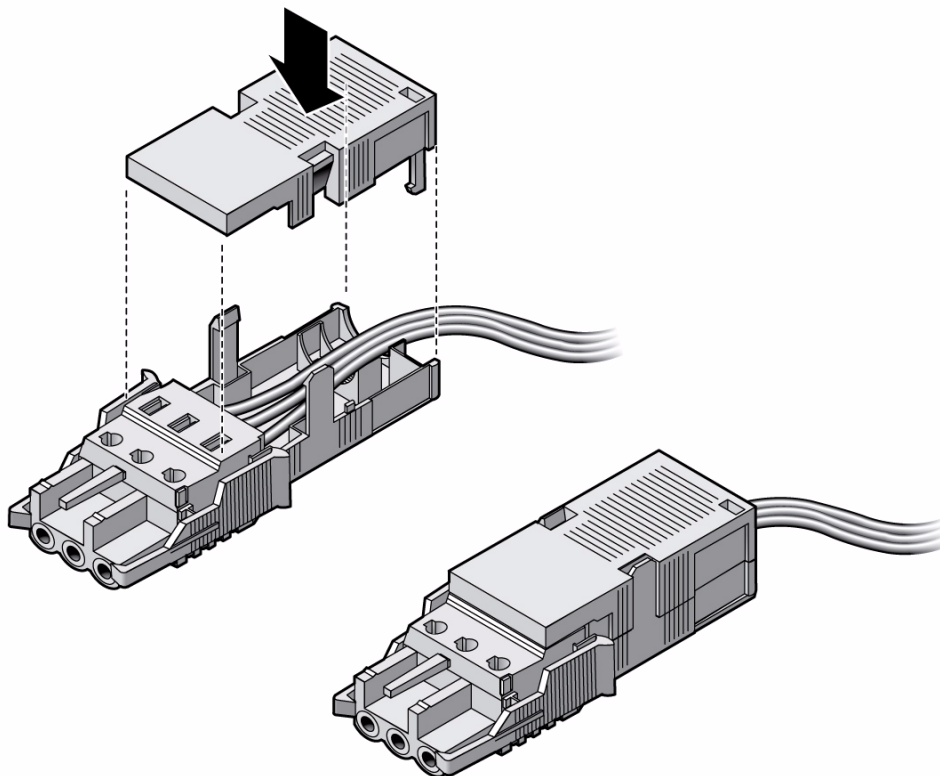
図 9 保護カバーの組み立て
