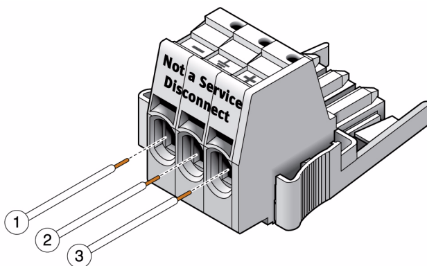
図 4 コネクタの配線の割り当て
