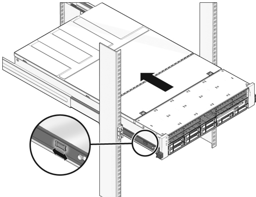
図9 Express レールのリリースタブのスライドと、ラックへのサーバの固定
