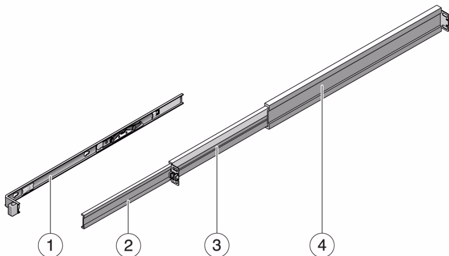
図1 Express レールのスライドレール構成部品のセクション
