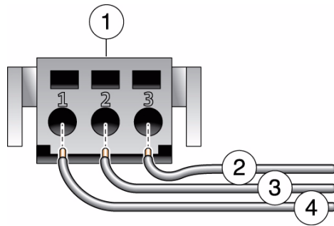
図 5 コネクタの配線の割り当て
