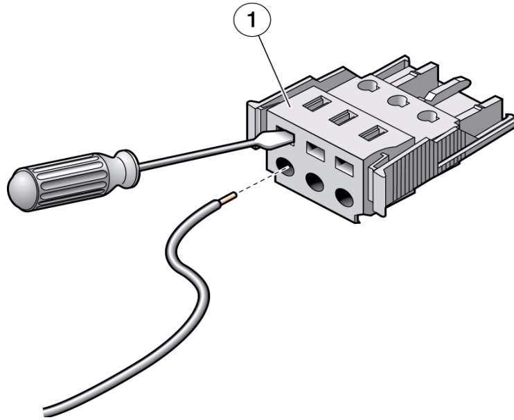
図 4 ねじ回しを使用して、ケージランプを開く方法
