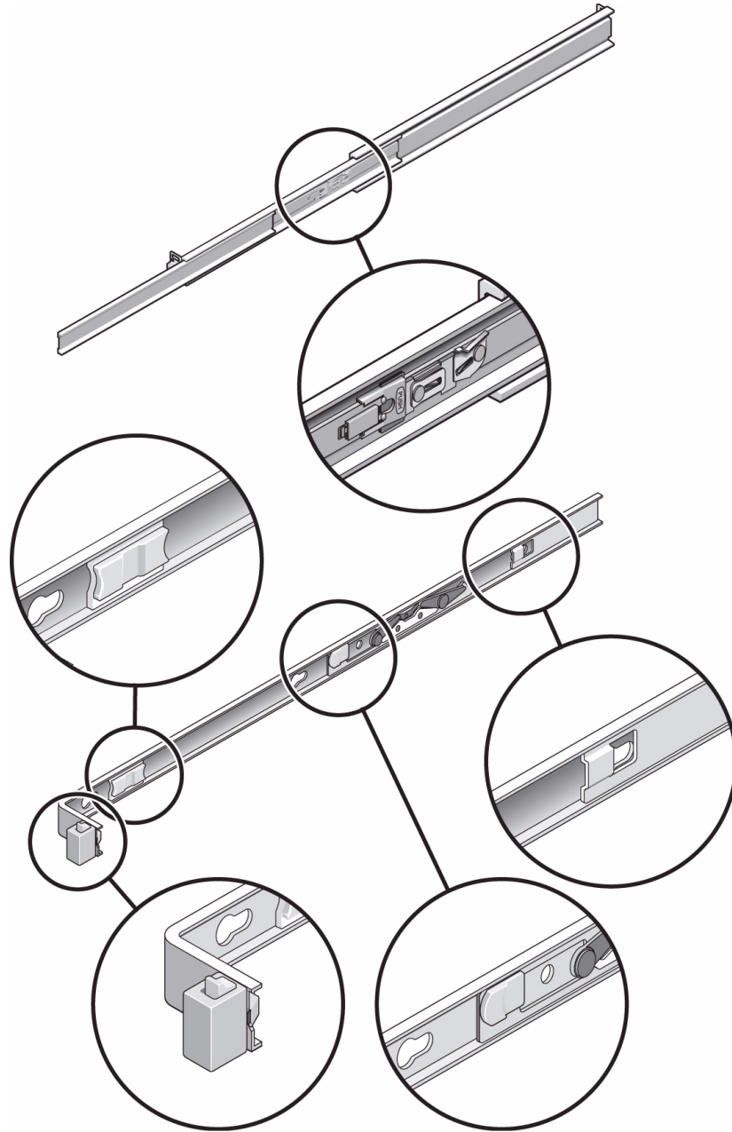
図 9 Sun SPARC Enterprise T5240 サーバのスライドレール構成部品のロックの位置
