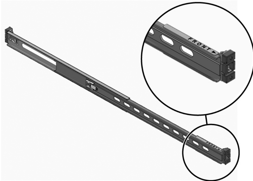
図 6 取り付け時の Express レールのスライドレールの向き
