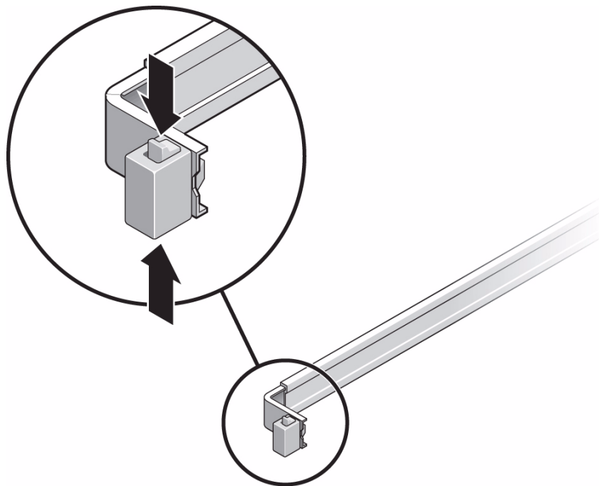
図3 Express レールのスライドレール構成部品のロックの解除
