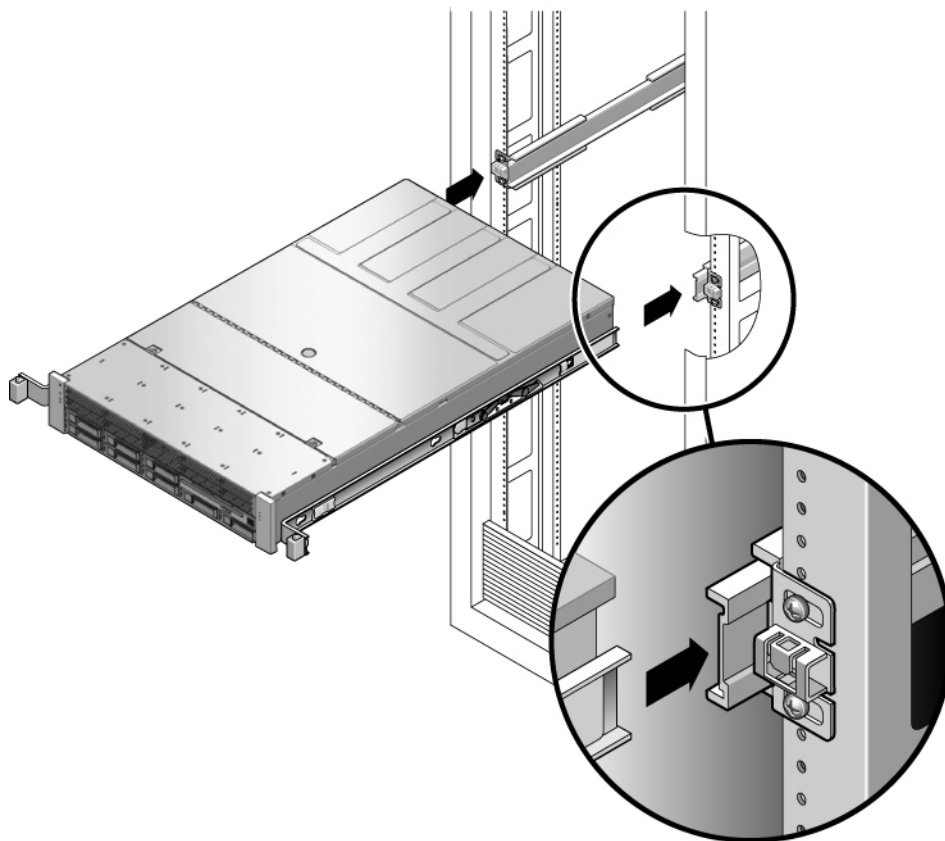
図 7 スライドレールへのシャーシの取り付け (両方のサーバに適用)
