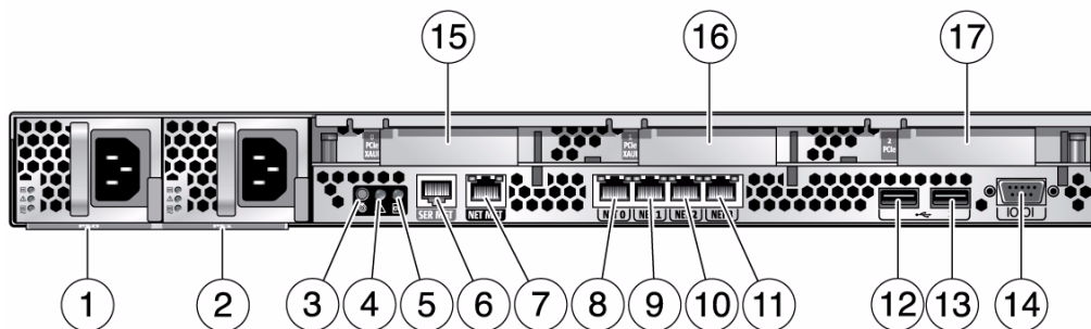
図 4 Sun SPARC Enterprise T5140 サーバの背面パネルのケーブルコネクタおよび LED
