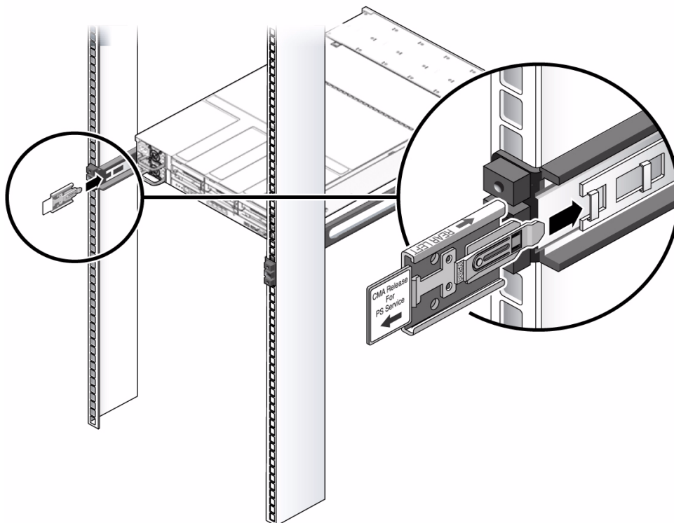
図 8 左のスライドレールの背面側への CMA レール拡張部品の挿入 (両方のサーバに適用)
