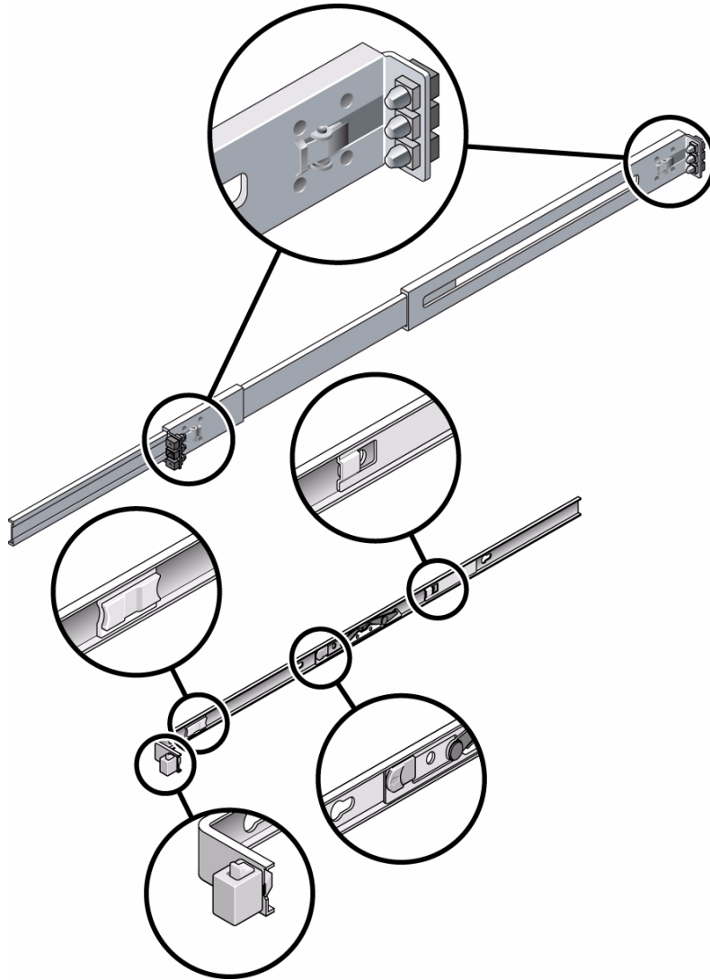
図 2 Sun SPARC Enterprise T5240 サーバのスライドレール構成部品のロックの位置
