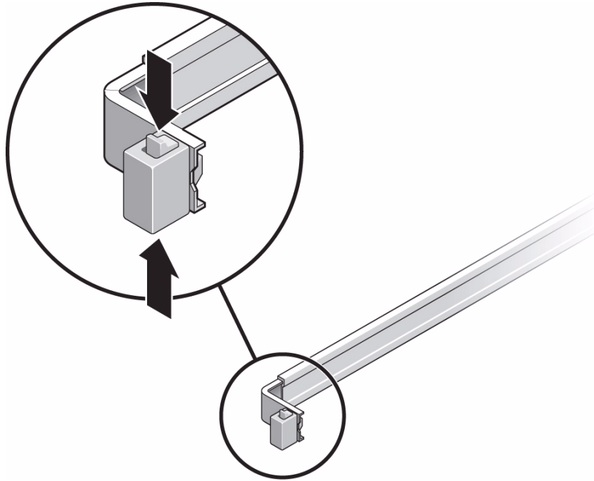
図 12 スライドレール構成部品のロックの解除 (両方のサーバに適用)
