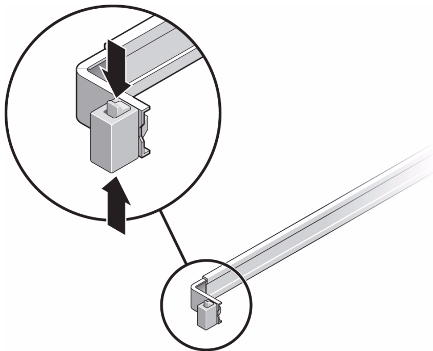
図 1 スライドレール構成部品のロックの解除 (両方のサーバに適用)
