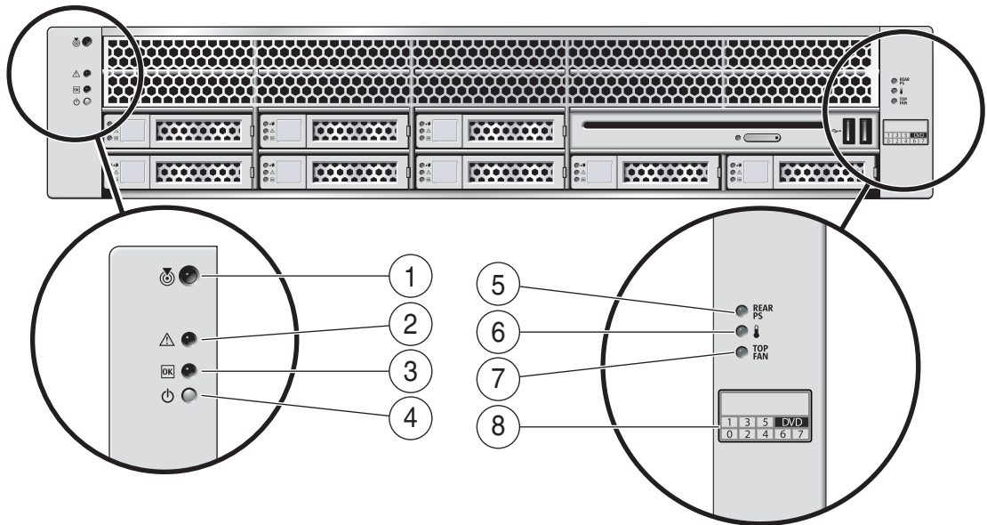
FIGURA 1-2 Acceso a los componentes frontales (servidor Sun SPARC Enterprise T5240 con ocho discos)
