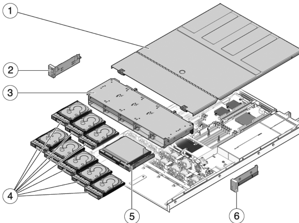
FIGURA A-2 Componentes de E/S (servidor Sun SPARC Enterprise T5140)
