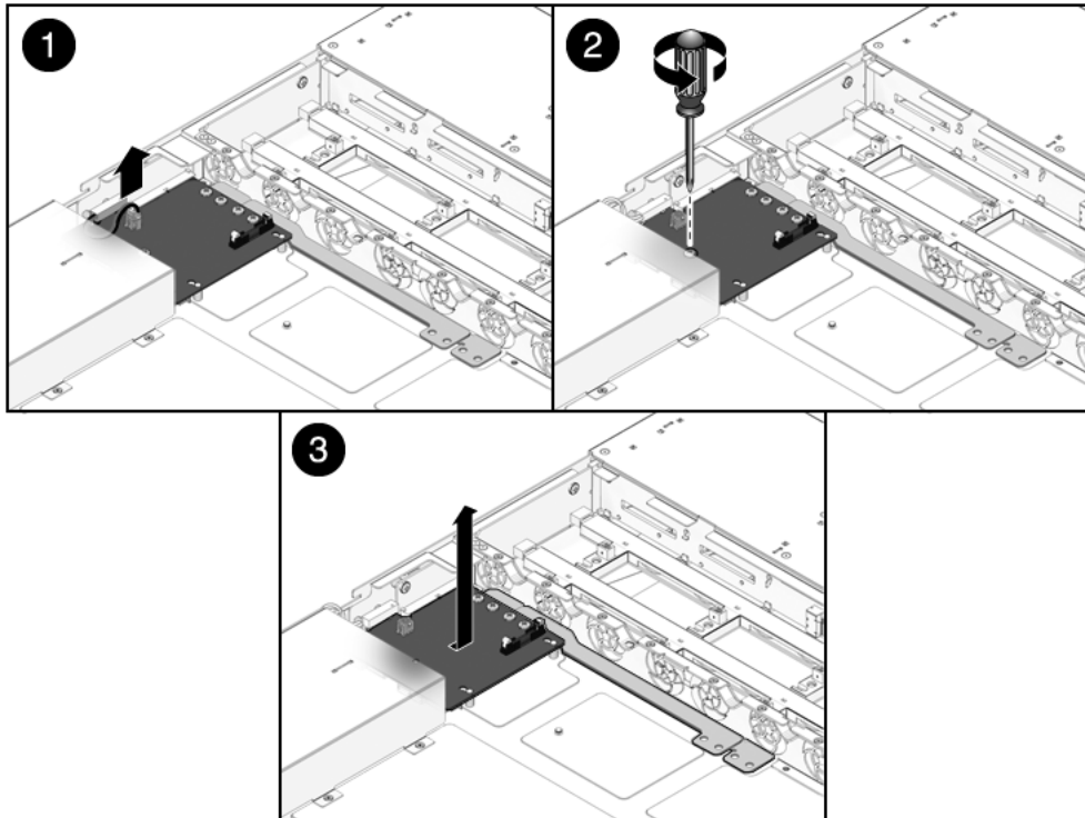
FIGURA 6-15 Extracción de la placa de distribución de alimentación (servidor Sun SPARC Enterprise T5140)
