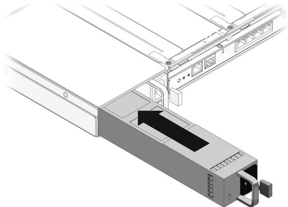
FIGURA 6-18 Instalación de la fuente de alimentación (servidor Sun SPARC Enterprise T5140)
