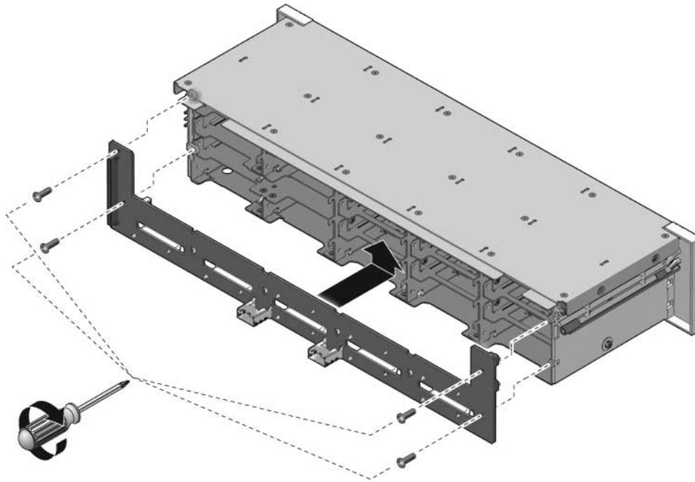
FIGURA 6-10 Instalación de la placa posterior de unidades de disco (servidor Sun SPARC Enterprise T5240)
