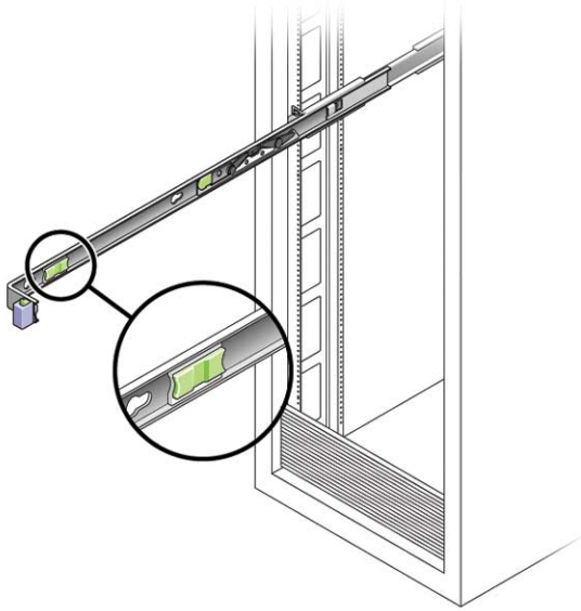
FIGURA 3-3 Lengüetas de liberación y conjunto de guías
