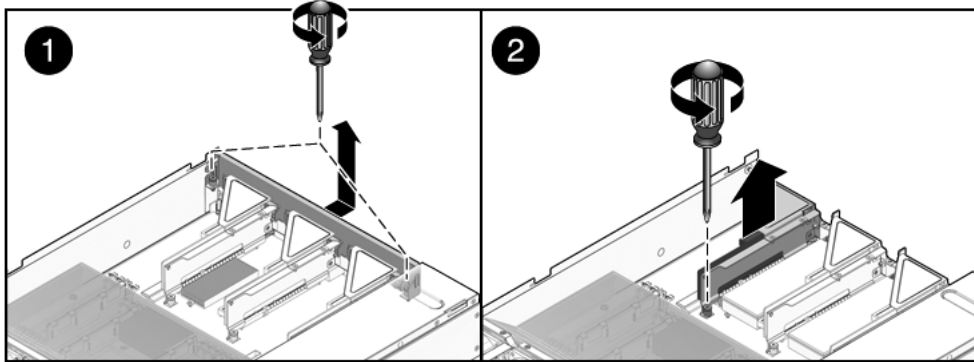
FIGURA 5-11 Extracción de la placa vertical PCIe/XAUI (Sun SPARC Enterprise T5140)
