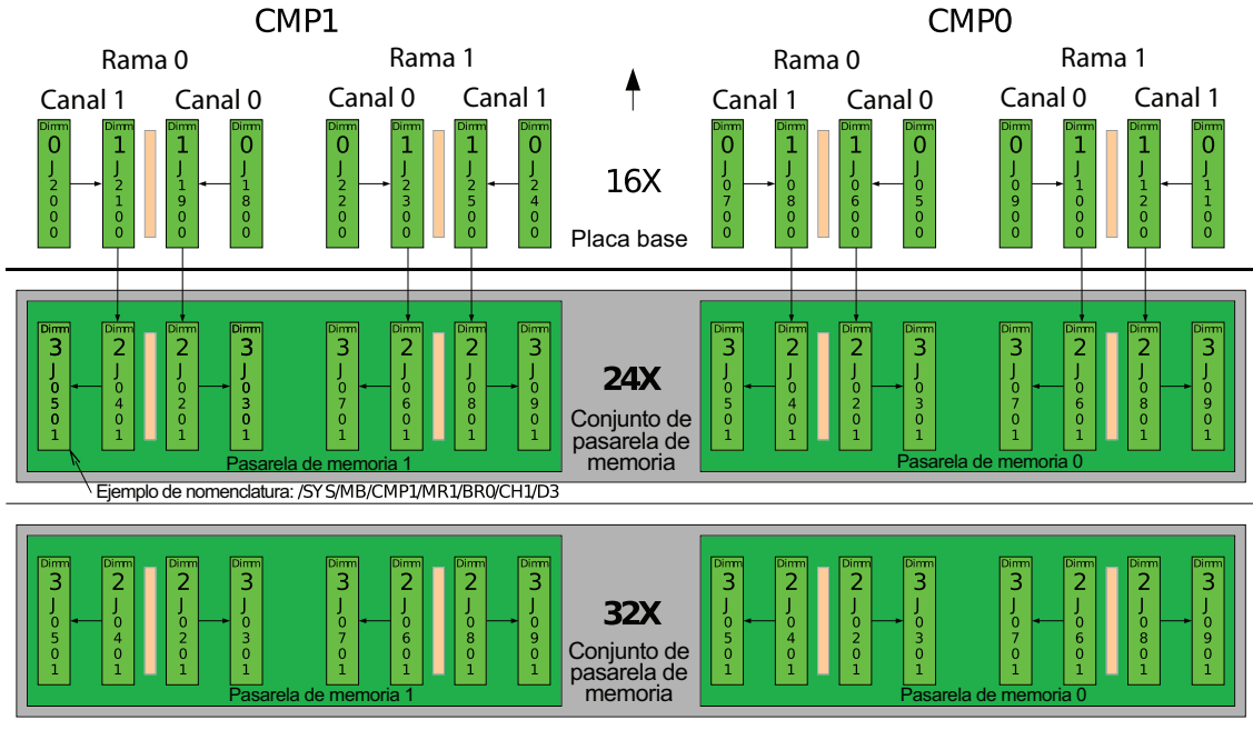
FIGURA 5-7 Configuración de los FB-DIMM (conjunto de pasarela de memoria de Sun SPARC Enterprise T5240)
