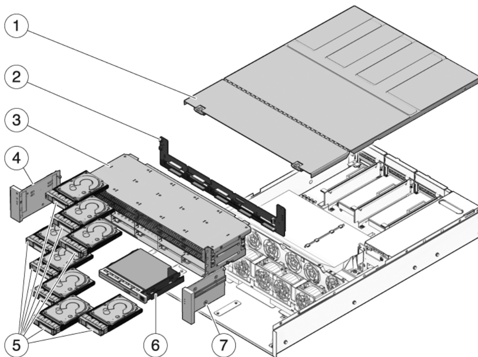
FIGURA A-9 Componentes de E/S (servidor Sun SPARC Enterprise T5240)
