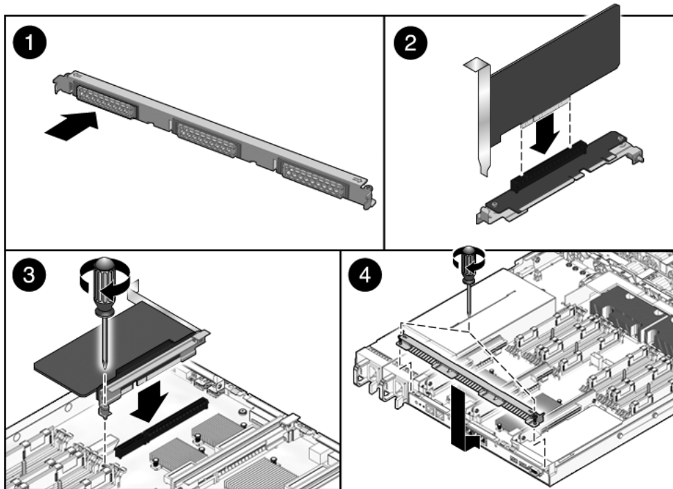
FIGURA 5-15 Instalación de la tarjeta PCIe (Sun SPARC Enterprise T5140)
