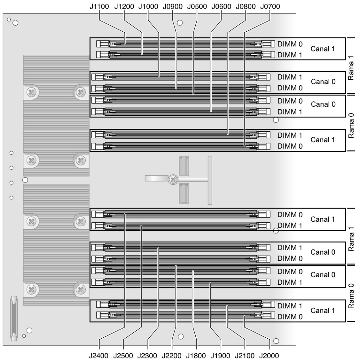
FIGURA 5-4 Ubicación física de los FB-DIMM (Sun SPARC Enterprise T5140)
