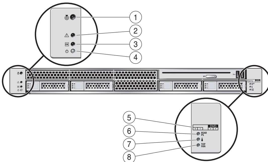
FIGURA 1-1 Acceso a los componentes frontales (servidor Sun SPARC Enterprise T5140)
