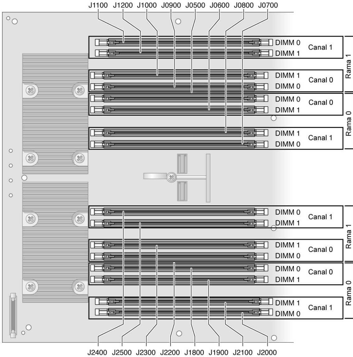
FIGURA 5-6 Ubicación física de los FB-DIMM en la placa base (Sun SPARC Enterprise T5240)
