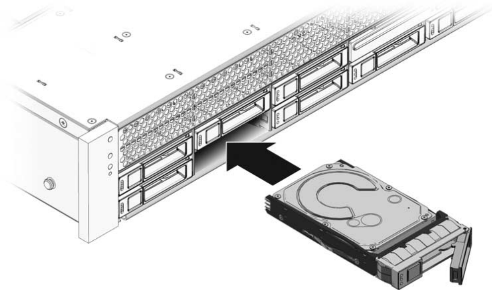
FIGURA 4-3 Instalación de una unidad de disco (servidor Sun SPARC Enterprise T5240)
