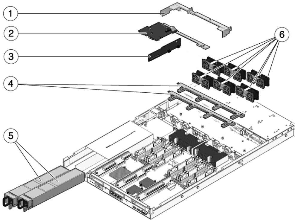
FIGURA A-3 Componentes de distribución de alimentación/módulo de ventiladores (servidor Sun SPARC Enterprise T5140)
