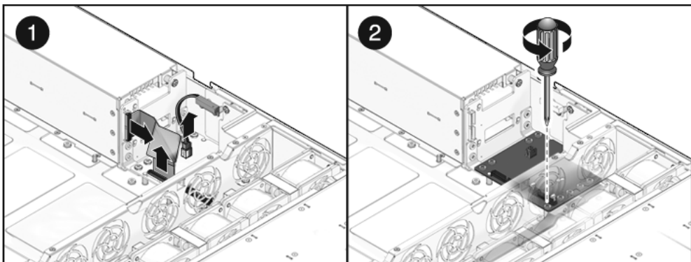
FIGURA 6-14 Extracción de la placa de distribución de alimentación (servidor Sun SPARC Enterprise T5240)
