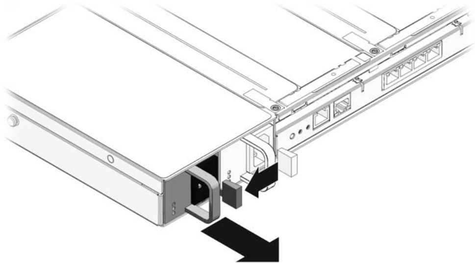
FIGURA 6-13 Extracción de la fuente de alimentación (servidor Sun SPARC Enterprise T5140)
