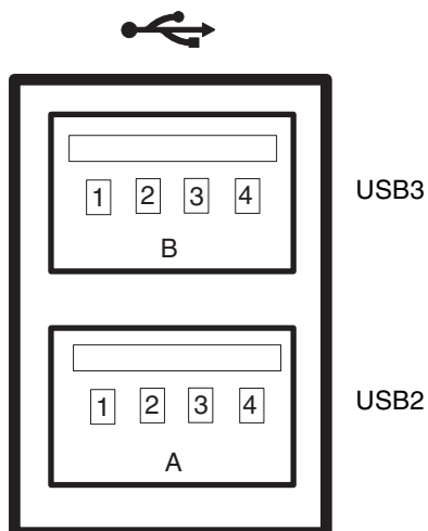
FIGURA B-4 Diagrama de conectores USB
