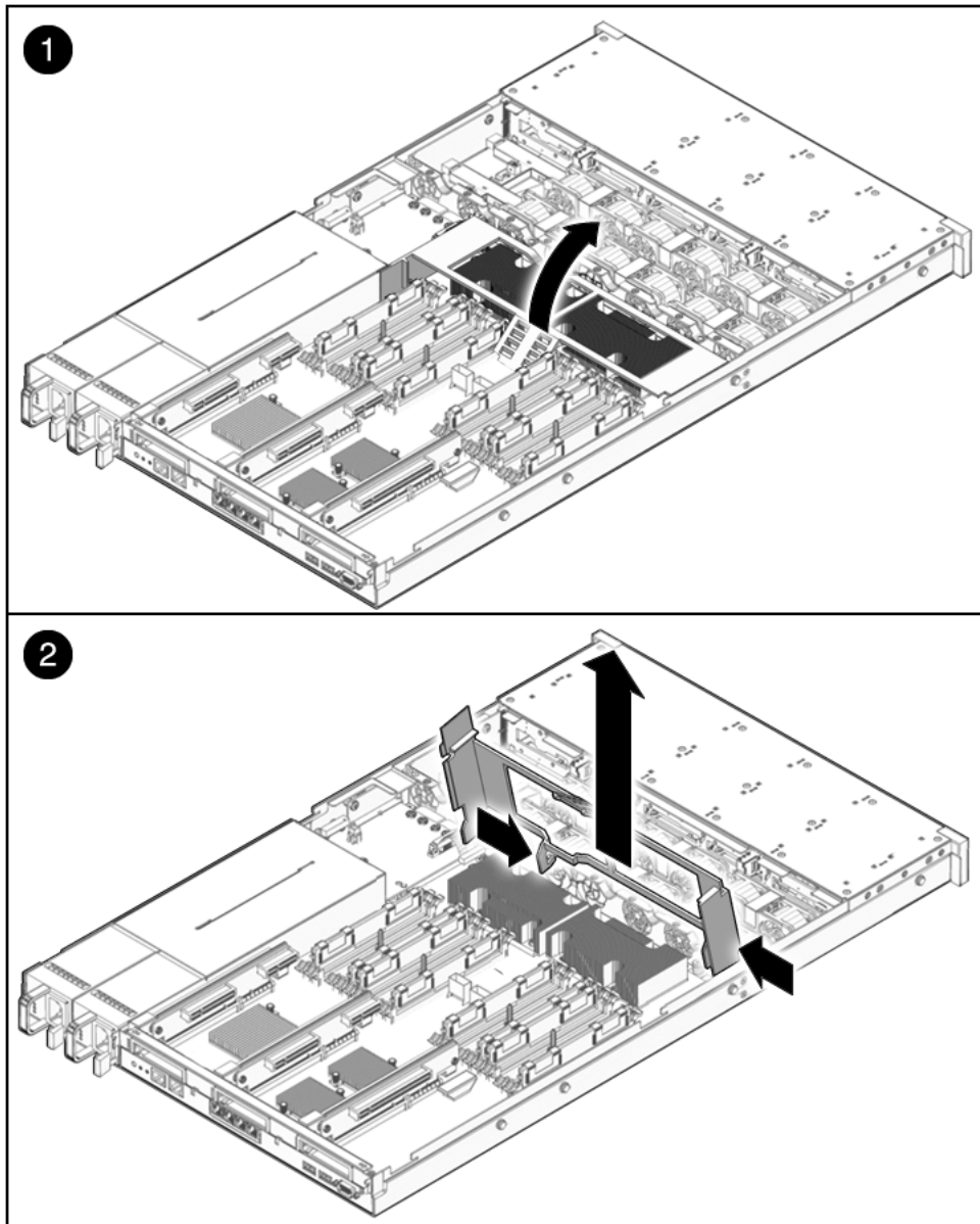
FIGURA 5-9 Extracción del deflector de aire (servidor Sun SPARC Enterprise T5140)
