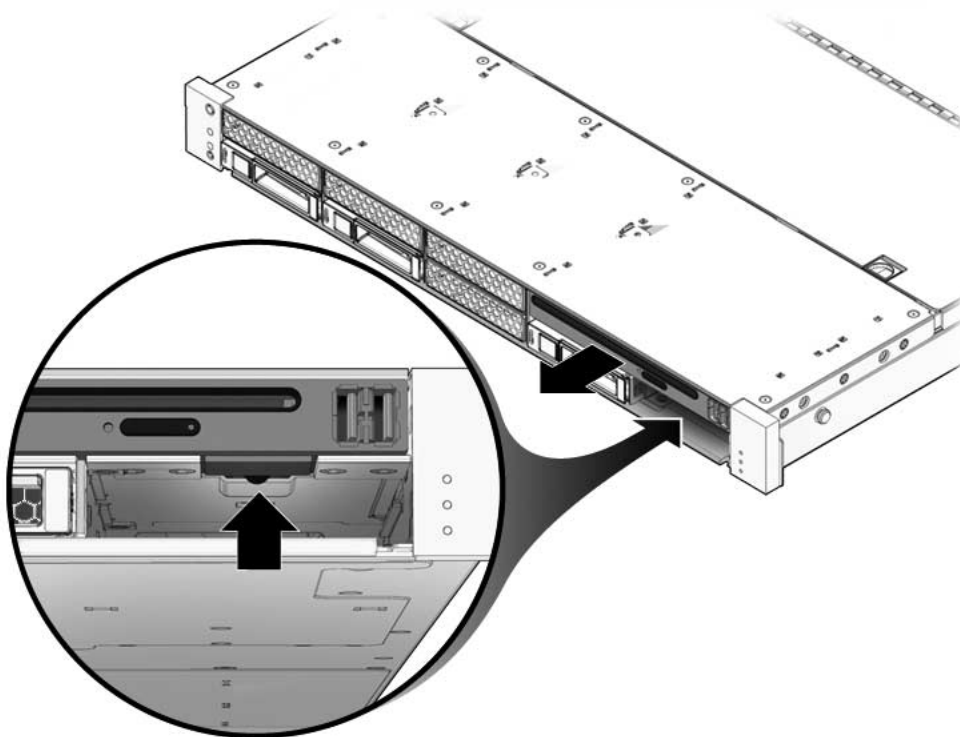
FIGURA 6-1 Extracción del módulo de DVD/USB (Sun SPARC Enterprise T5140)
