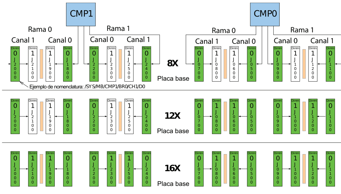
FIGURA 5-3 Configuración de los FB-DIMM (Sun SPARC Enterprise T5140)
