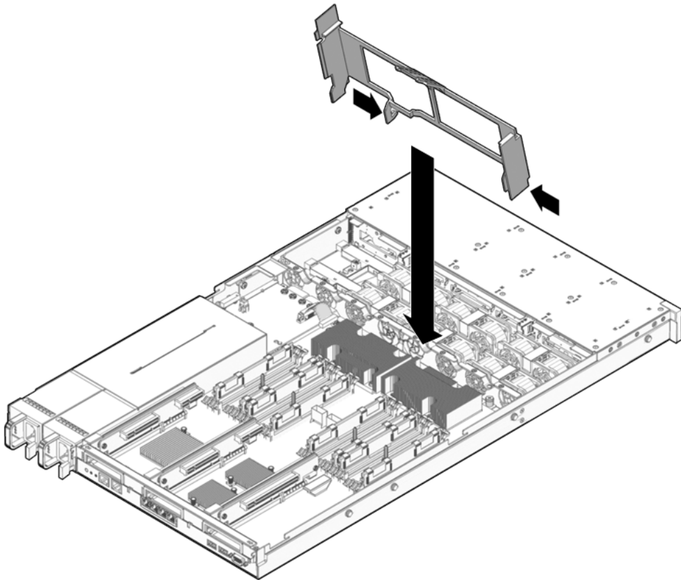
FIGURA 5-10 Instalación del deflector de aire (Sun SPARC Enterprise T5140)
