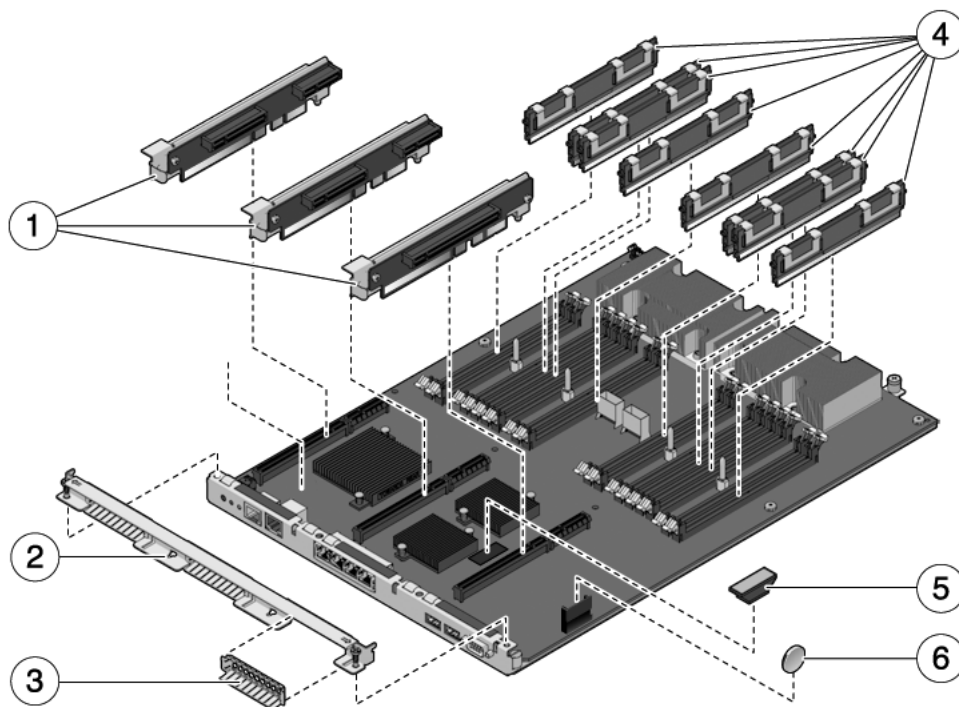
FIGURA A-1 Componentes de la placa base (servidor Sun SPARC Enterprise T5140)
