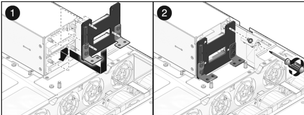
FIGURA 6-21 Instalación de la placa posterior de fuente de alimentación (servidor Sun SPARC Enterprise T5240)
