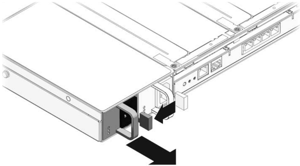
FIGURA 4-8 Manilla de liberación de la fuente de alimentación (Sun SPARC Enterprise T5140)
