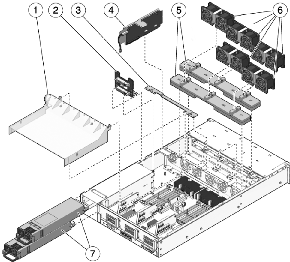
FIGURA A-10 Componentes de distribución de alimentación/módulo de ventiladores (servidor Sun SPARC Enterprise T5240)
