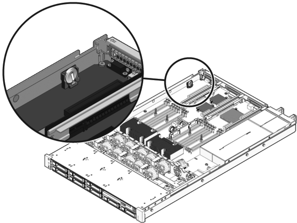
FIGURA 5-17 Ubicación de la batería (servidor Sun SPARC Enterprise T5140)
