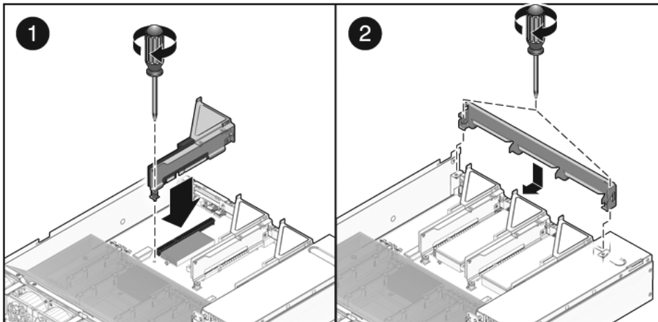
FIGURA 5-12 Extracción de la placa vertical PCIe/XAUI (Sun SPARC Enterprise T5240)
