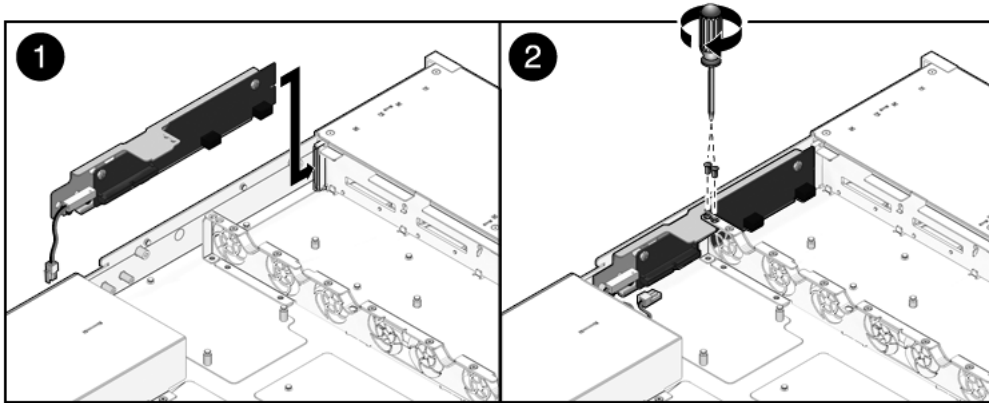
FIGURA 6-24 Instalación de la tarjeta de ranuras (servidor Sun SPARC Enterprise T5140)
