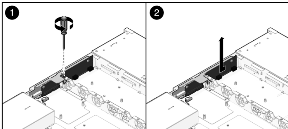
FIGURA 6-23 Extracción de la tarjeta de ranuras (servidor Sun SPARC Enterprise T5140)
