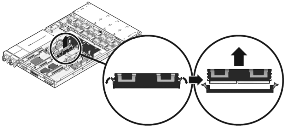
FIGURA 5-2 Extracción de los módulos FB-DIMM
