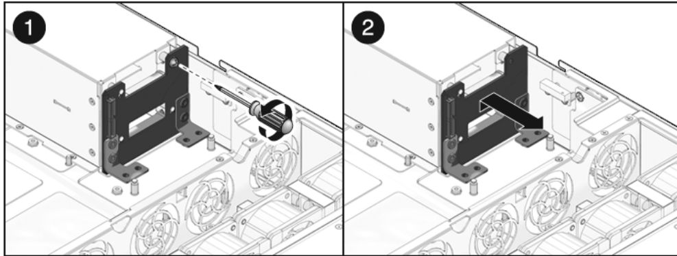
FIGURA 6-20 Extracción de la placa posterior de fuente de alimentación (servidor Sun SPARC Enterprise T5240)
