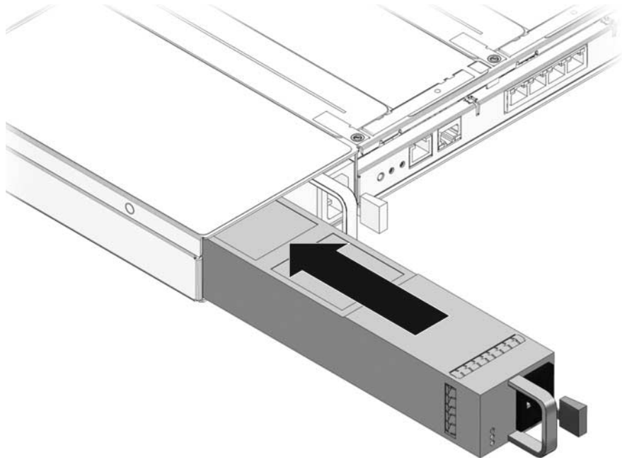
FIGURA 4-10 Instalación de la fuente de alimentación (Sun SPARC Enterprise T5140)
