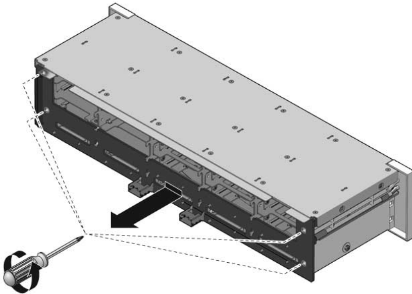
FIGURA 6-8 Extracción de la placa posterior de unidades de disco (servidor Sun SPARC Enterprise T5240)
