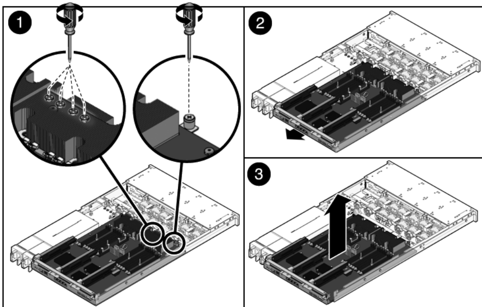
FIGURA 5-21 Extracción del conjunto de la placa base (servidor Sun SPARC Enterprise T5140 ilustrado)
