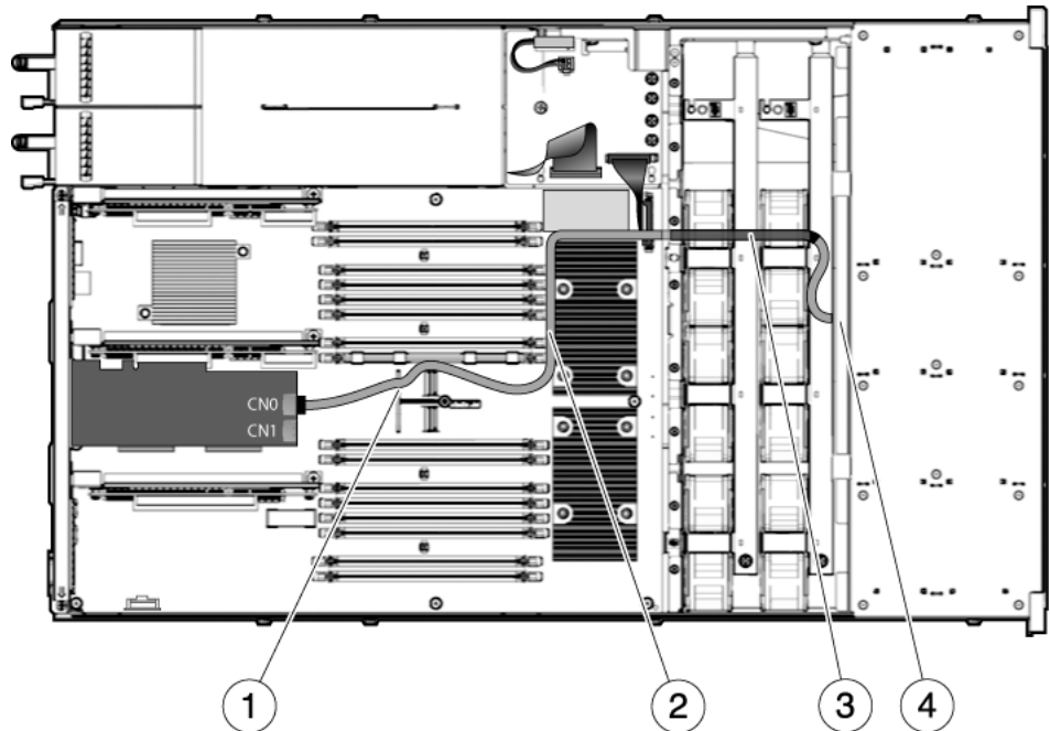
FIGURA A-5 Tendido del cable de datos de disco duro para la tarjeta controladora PCIe SAS RAID en un servidor Sun SPARC Enterprise T5140 con capacidad para cuatro discos
