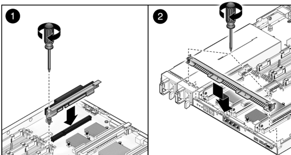
FIGURA 5-13 Instalación de la placa vertical PCIe/XAUI (Sun SPARC Enterprise T5140)
