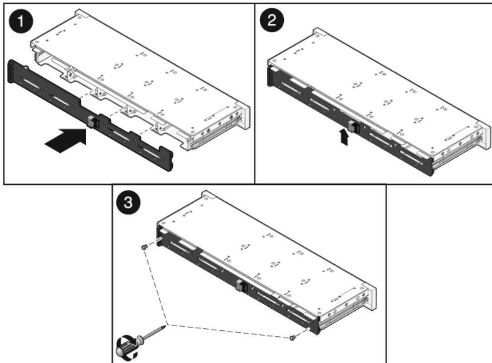
FIGURA 6-9 Instalación de la placa posterior de unidades de disco (servidor Sun SPARC Enterprise T5140)
