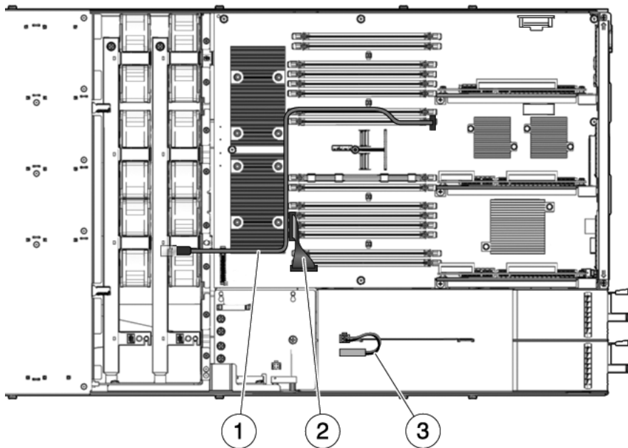
FIGURA A-4 Cables internos para la tarjeta controladora SAS integrada (servidor Sun SPARC Enterprise T5140)
