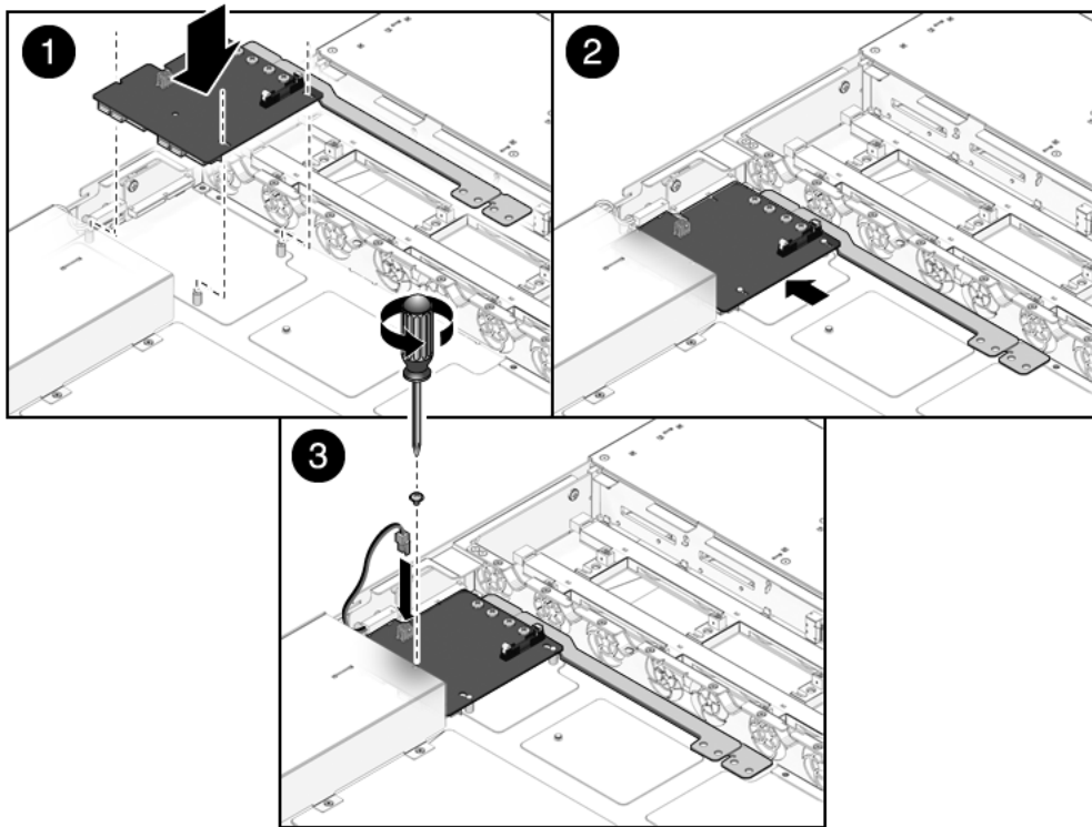
FIGURA 6-16 Instalación de la placa de distribución de alimentación (servidor Sun SPARC Enterprise T5140)
