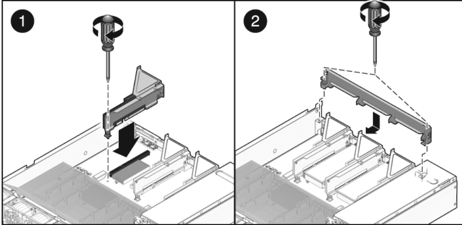
FIGURA 5-14 Instalación de la placa vertical PCIe/XAUI (Sun SPARC Enterprise T5240)
