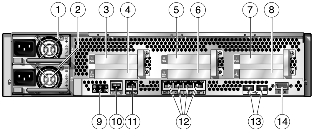
FIGURA 1-4 Acceso a los componentes posteriores (servidor Sun SPARC Enterprise T5240)
