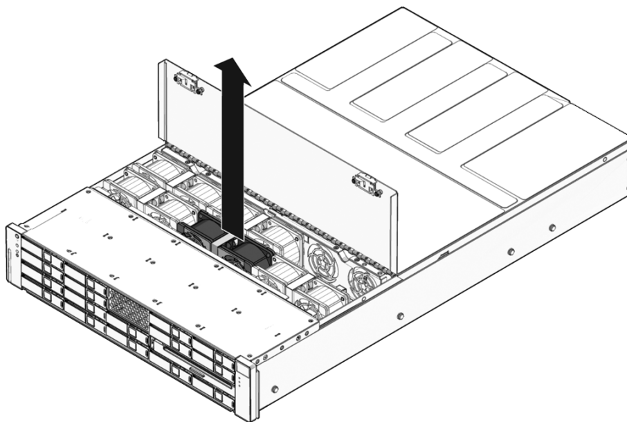
FIGURA 4-4 Extracción de un módulo de ventiladores
