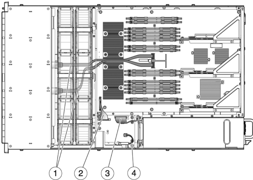
FIGURA A-11 Cables internos para la tarjeta controladora SAS integrada (servidor Sun SPARC Enterprise T5240)
