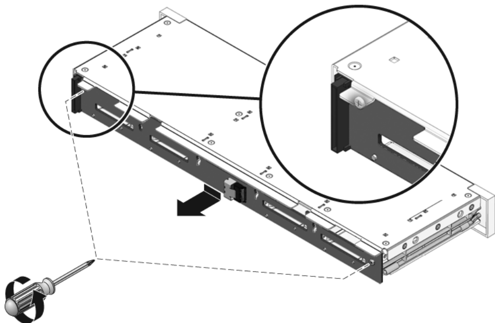
FIGURA 6-7 Extracción de la placa posterior de unidades de disco (servidor Sun SPARC Enterprise T5140)
