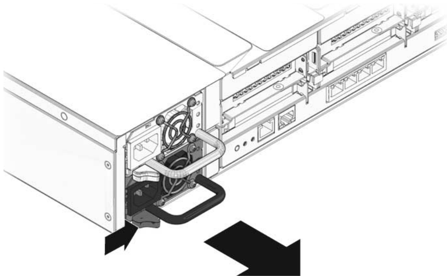
FIGURA 4-9 Manilla de liberación de la fuente de alimentación (Sun SPARC Enterprise T5240)
