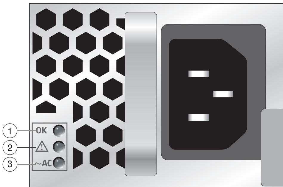
FIGURA 4-6 LED de estado de fuentes de alimentación (servidor Sun SPARC Enterprise T5140 ilustrado)
