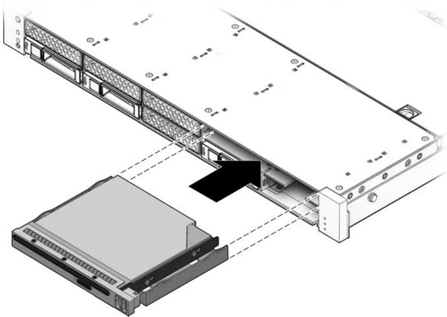
FIGURA 6-2 Instalación del módulo de DVD/USB (Sun SPARC Enterprise T5140)
