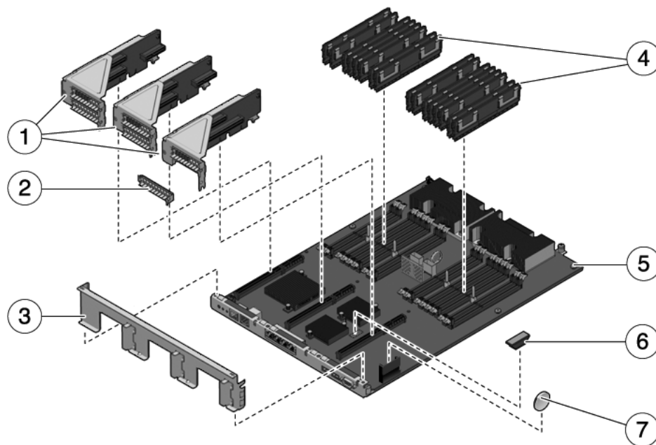
FIGURA A-7 Componentes de la placa base (servidor Sun SPARC Enterprise T5240)
