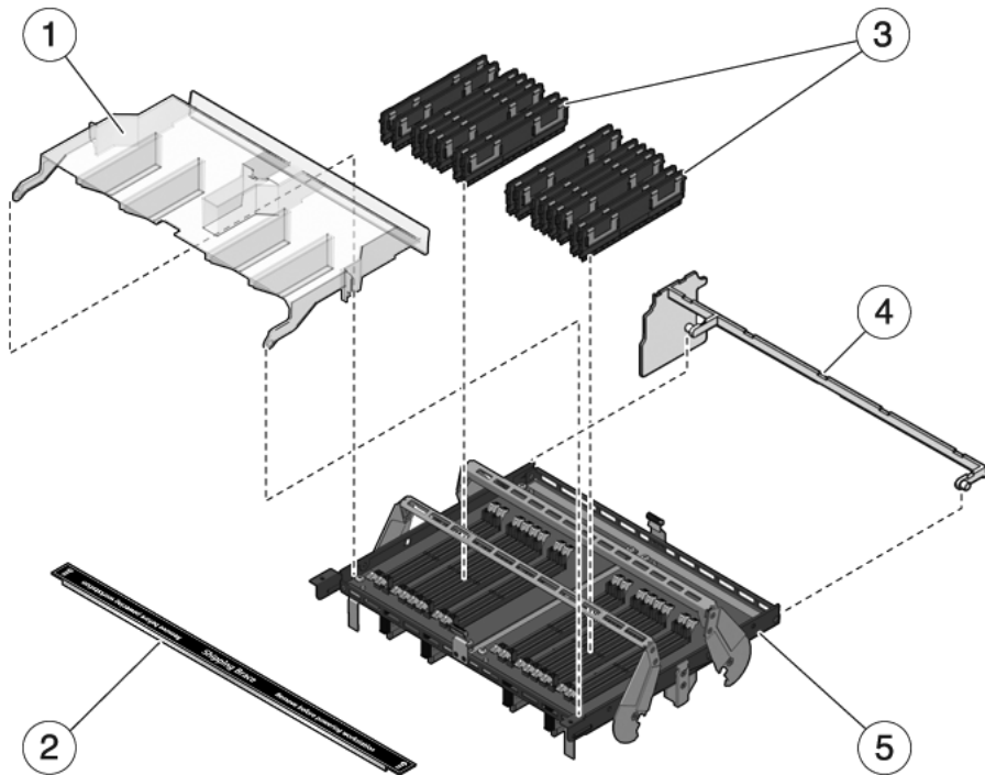
FIGURA A-8 Componentes del conjunto de pasarela de memoria
