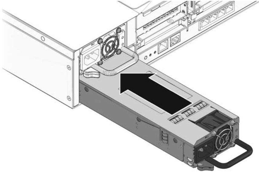
FIGURA 4-11 Instalación de la fuente de alimentación (Sun SPARC Enterprise T5240)
