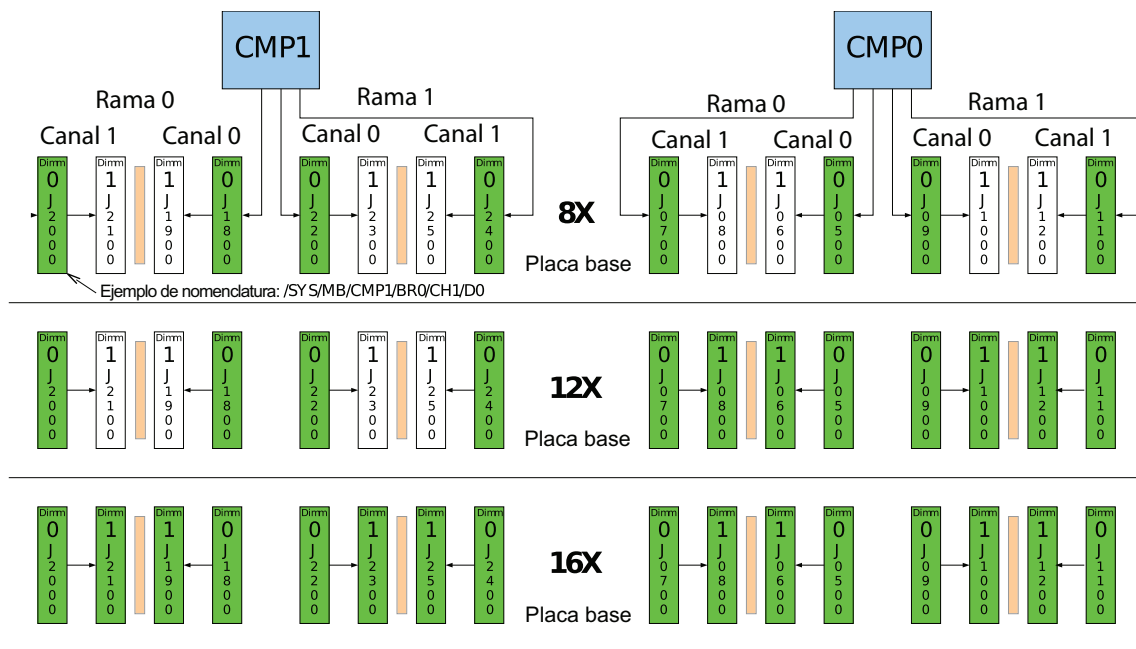
FIGURA 5-5 Configuración de los FB-DIMM (Sun SPARC Enterprise T5240)
