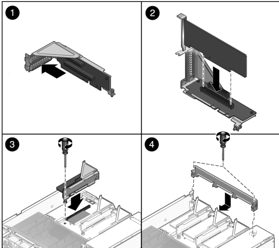
FIGURA 5-16 Instalación de la tarjeta PCIe (Sun SPARC Enterprise T5240)
