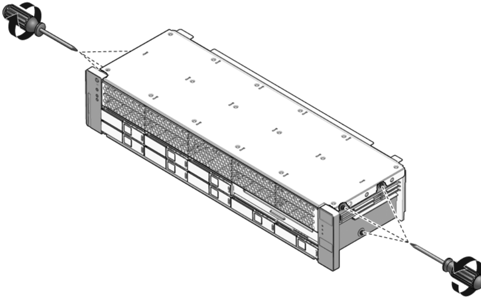
FIGURA 6-11 Extracción del conjunto de canales de luz del panel de control frontal (servidor Sun SPARC Enterprise T5240)
