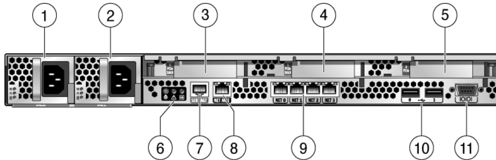
FIGURA 1-3 Acceso a los componentes posteriores (servidor Sun SPARC Enterprise T5140)
