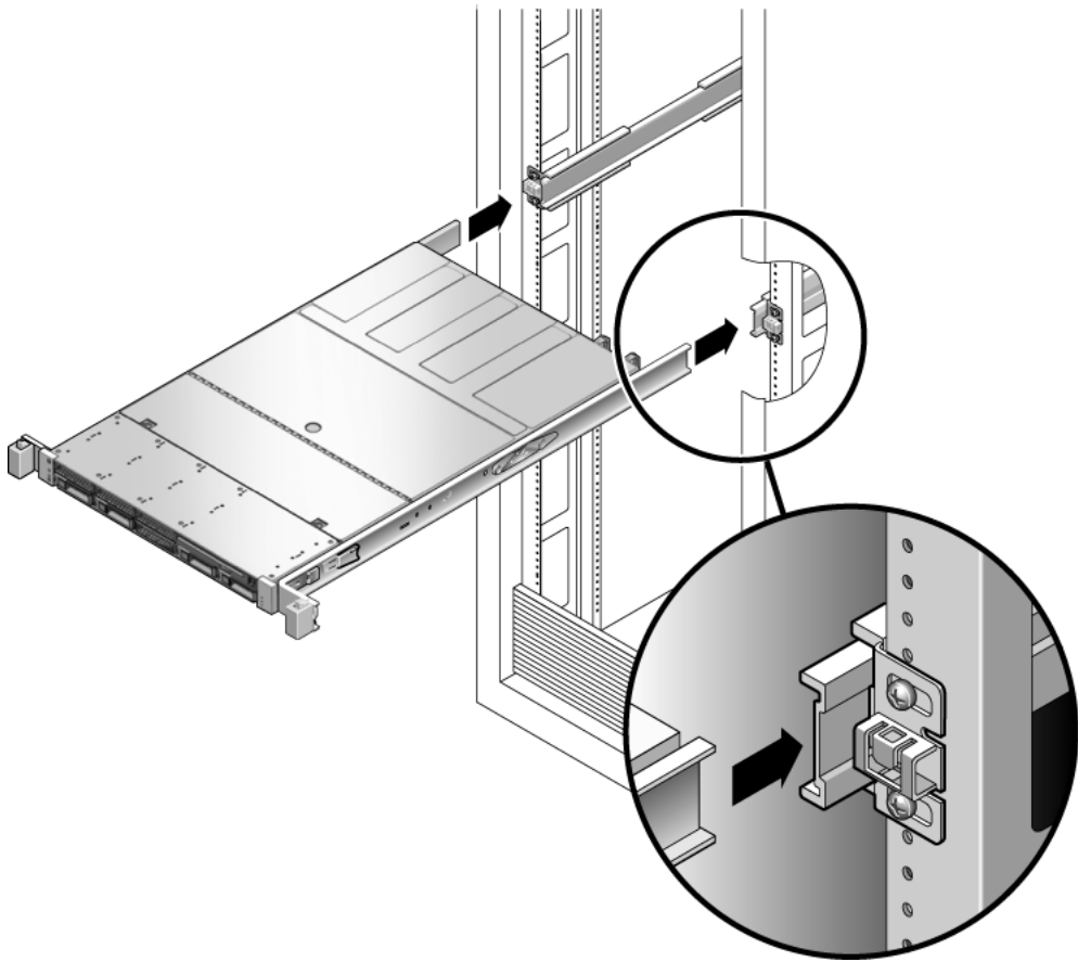
FIGURA 7-2 Colocación del servidor en el bastidor (servidor Sun SPARC Enterprise T5140)
