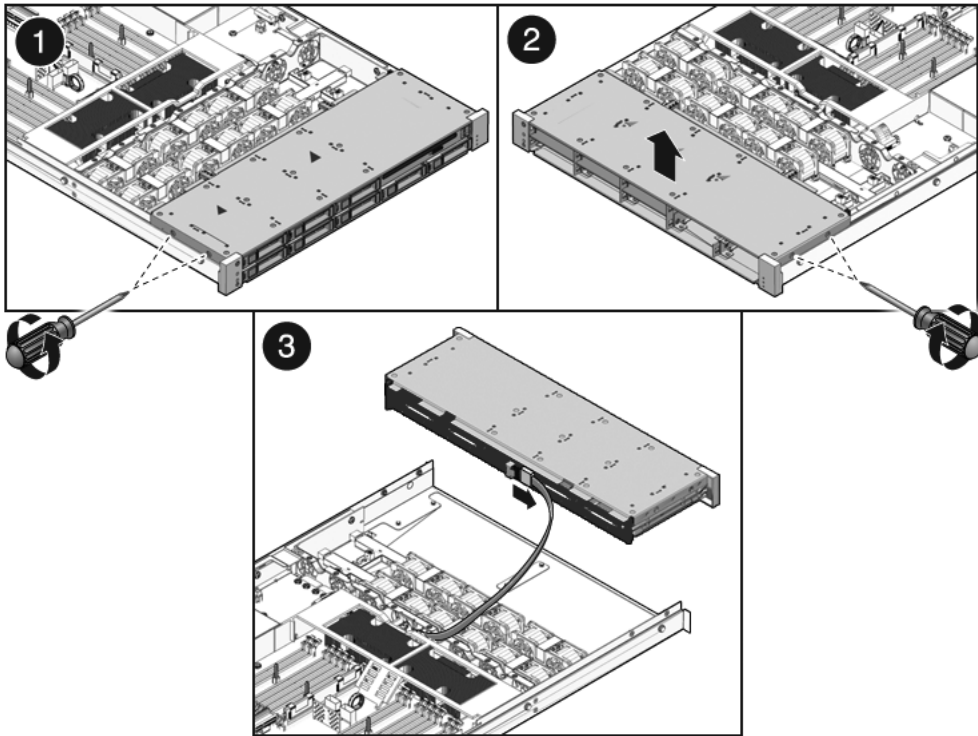
FIGURA 6-5 Extracción de la carcasa de unidades de disco (servidor Sun SPARC Enterprise T5140)
