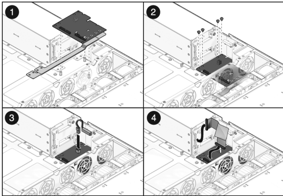
FIGURA 6-17 Instalación de la placa de distribución de alimentación (servidor Sun SPARC Enterprise T5240)
