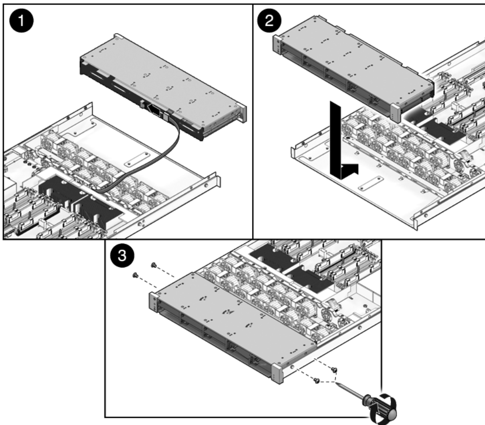
FIGURA 6-6 Instalación de la carcasa de unidades de disco (servidor Sun SPARC Enterprise T5140)
