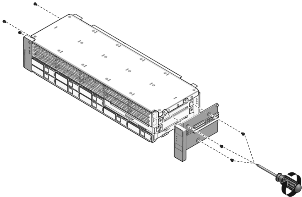
FIGURA 6-12 Instalación del conjunto de canales de luz del panel de control frontal (servidor Sun SPARC Enterprise T5240)
