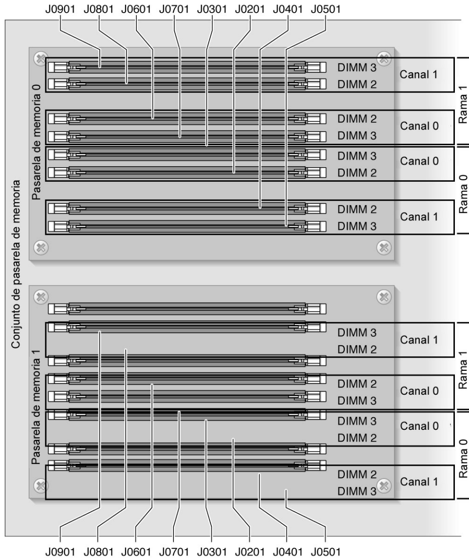
FIGURA 5-8 Ubicación física de los FB-DIMM en la pasarela de memoria (Sun SPARC Enterprise T5240)
