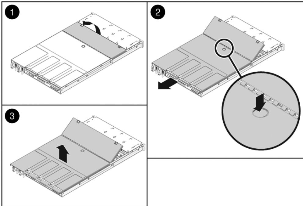
FIGURA 3-4 Extracción de la cubierta superior (servidor Sun SPARC Enterprise T5140)
