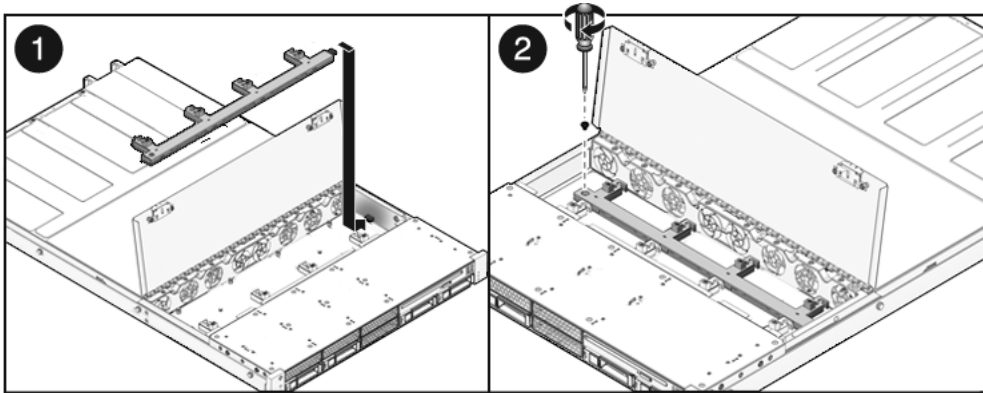
FIGURA 6-4 Instalación de la tarjeta de alimentación de ventilador (servidor Sun SPARC Enterprise T5140)
