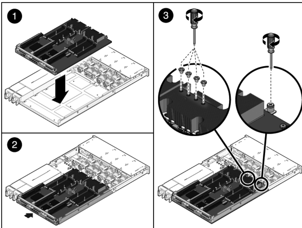
FIGURA 5-22 Instalación del conjunto de la placa base (servidor Sun SPARC Enterprise T5140)
