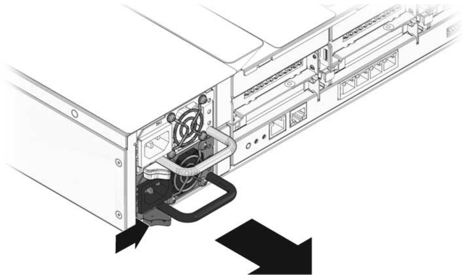
FIGURA 6-19 Extracción de la fuente de alimentación (servidor Sun SPARC Enterprise T5240)
