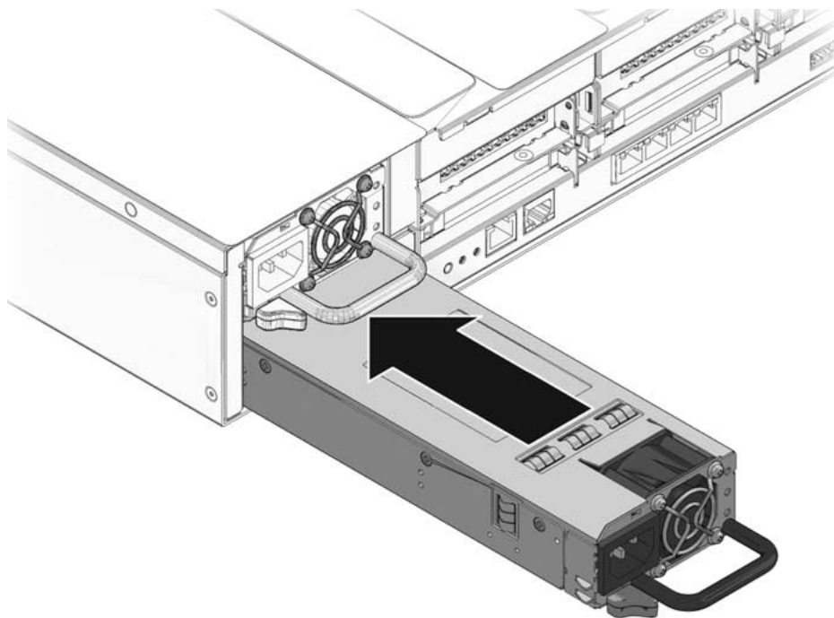
FIGURA 6-22 Instalación de la fuente de alimentación (servidor Sun SPARC Enterprise T5240)
