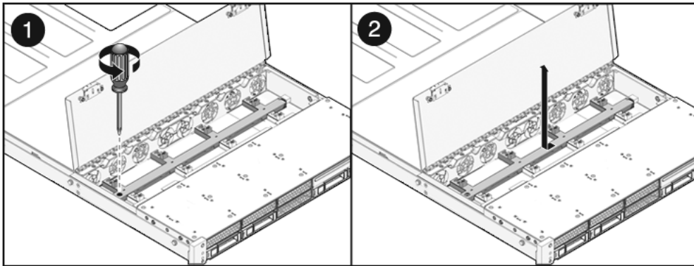
FIGURA 6-3 Extracción de la tarjeta de alimentación de ventilador (Sun SPARC Enterprise T5140)
