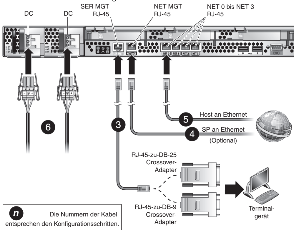
ABBILDUNG 2 Serververbindungen
