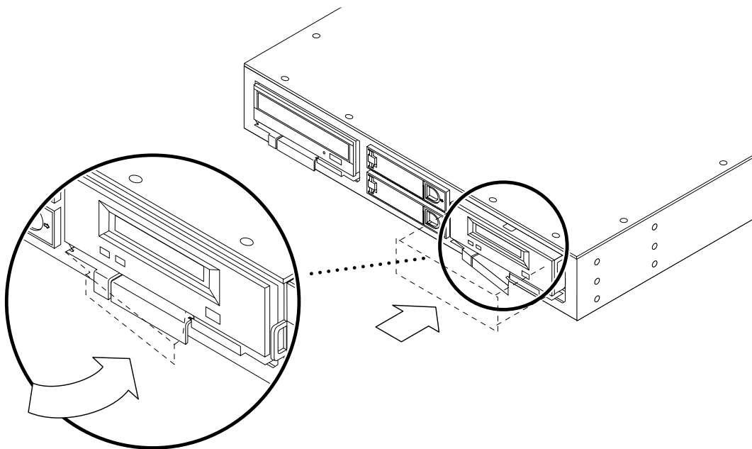
FIGURE 4-3 Fixation du verrou de la glissière de guidage (illustration d'un lecteur de bande)
