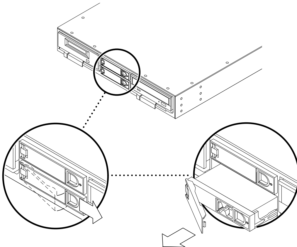
FIGURE 4-1 Ouverture d'un lecteur de disque dur
