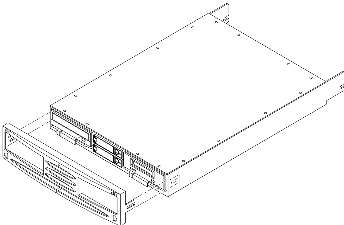
FIGURE 1-2 Plateau de stockage montable en armoire Sun StorEdge D240 avec chanfrein avant amovible
