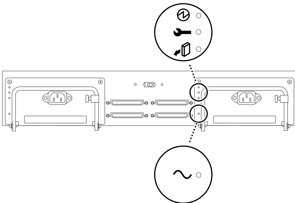
FIGURE 3-8 Emplacement des voyants d'état de l'alimentation
