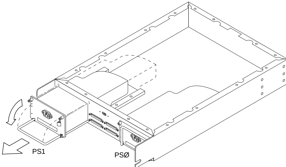
FIGURE 4-4 Retrait d'une unité d'alimentation
