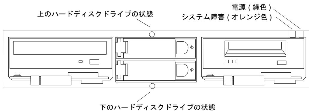
図 3-7 正面の LED (正面ベゼルを外した状態)
