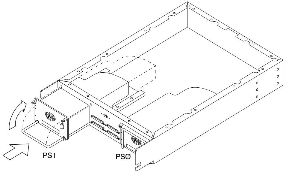
图 4-5 安装电源设备
