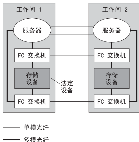
图 4-1 使用基于主机的数据复制的双工作间校园群集（无多路径功能）
