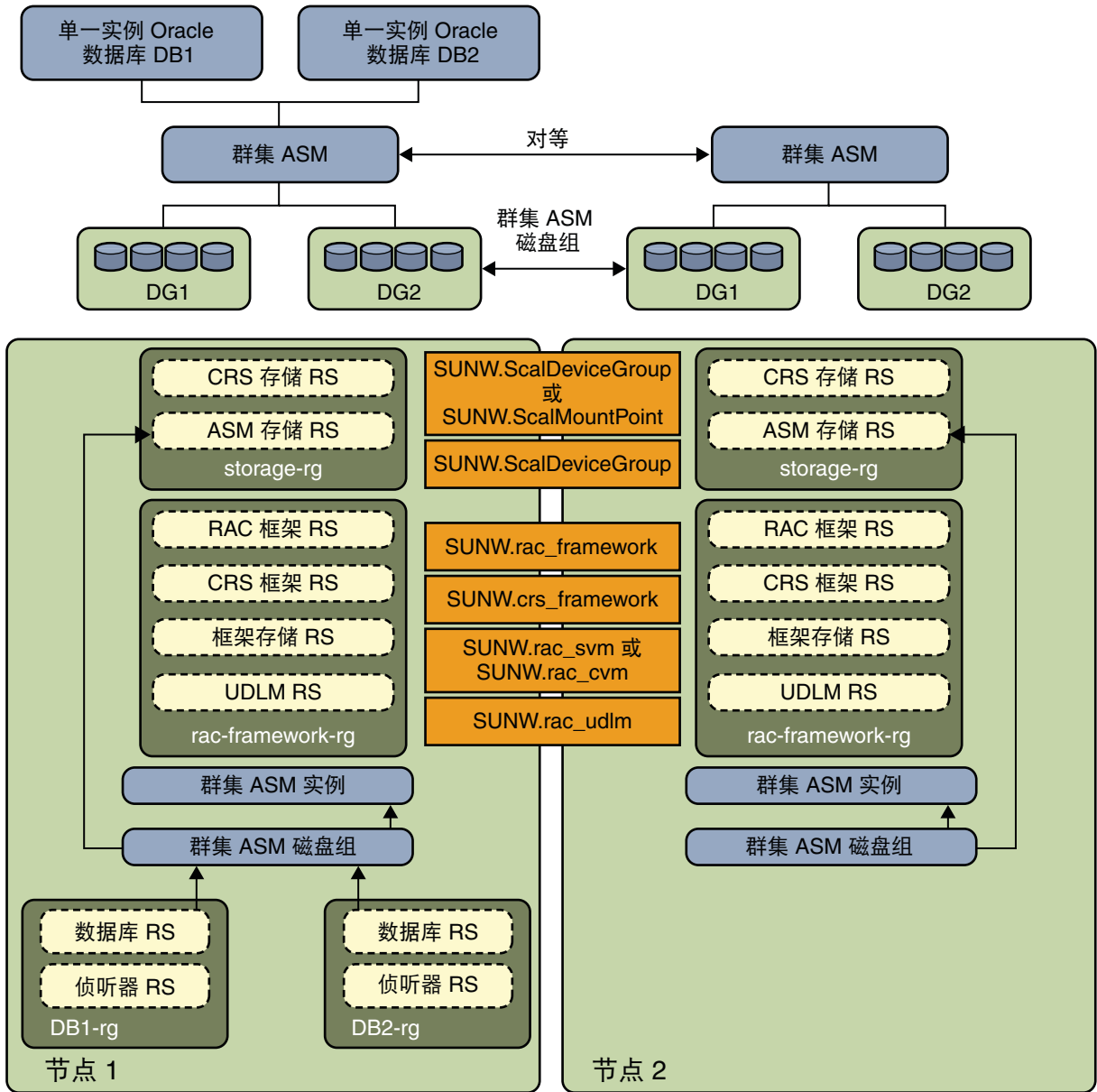
图 4 具有群集磁盘组的群集 ASM [1]
