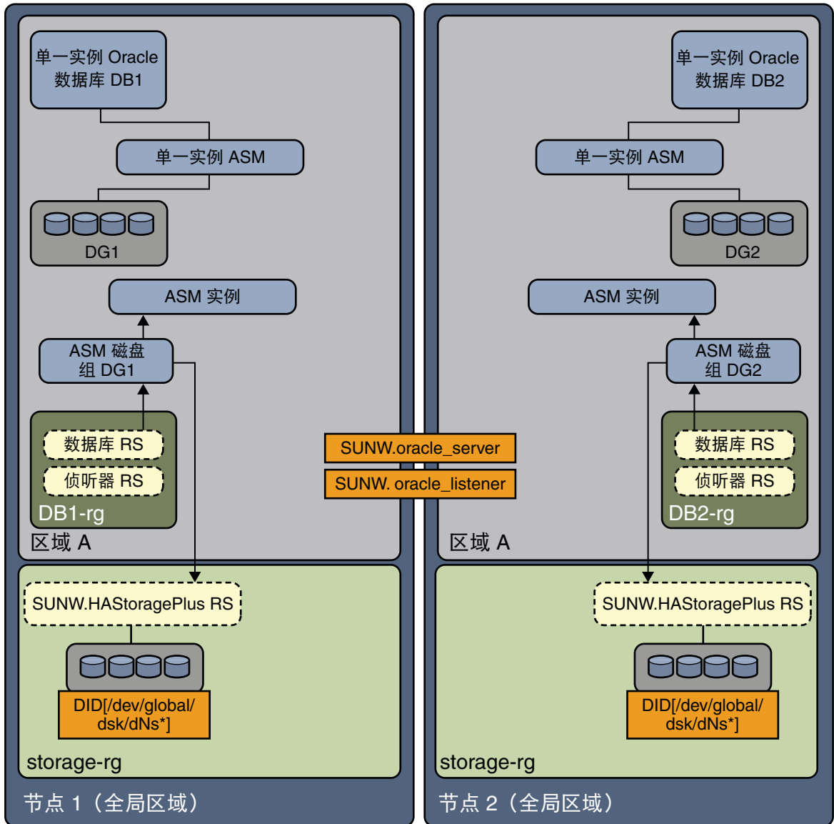
图 7 非全局区域中具有单独磁盘组的单实例 ASM [2]
