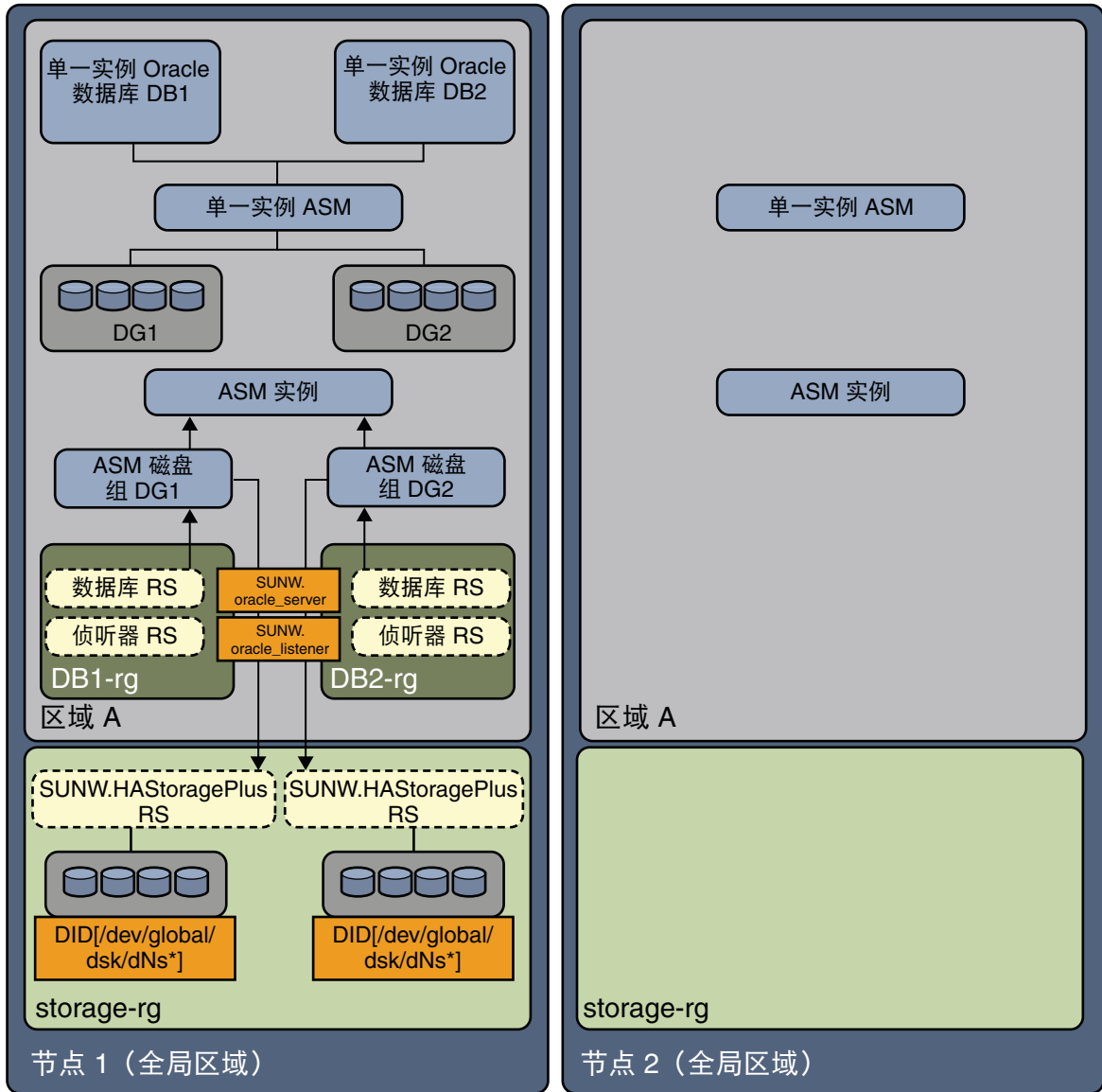
图 6 非全局区域中具有单独磁盘组的单实例 ASM [1]
