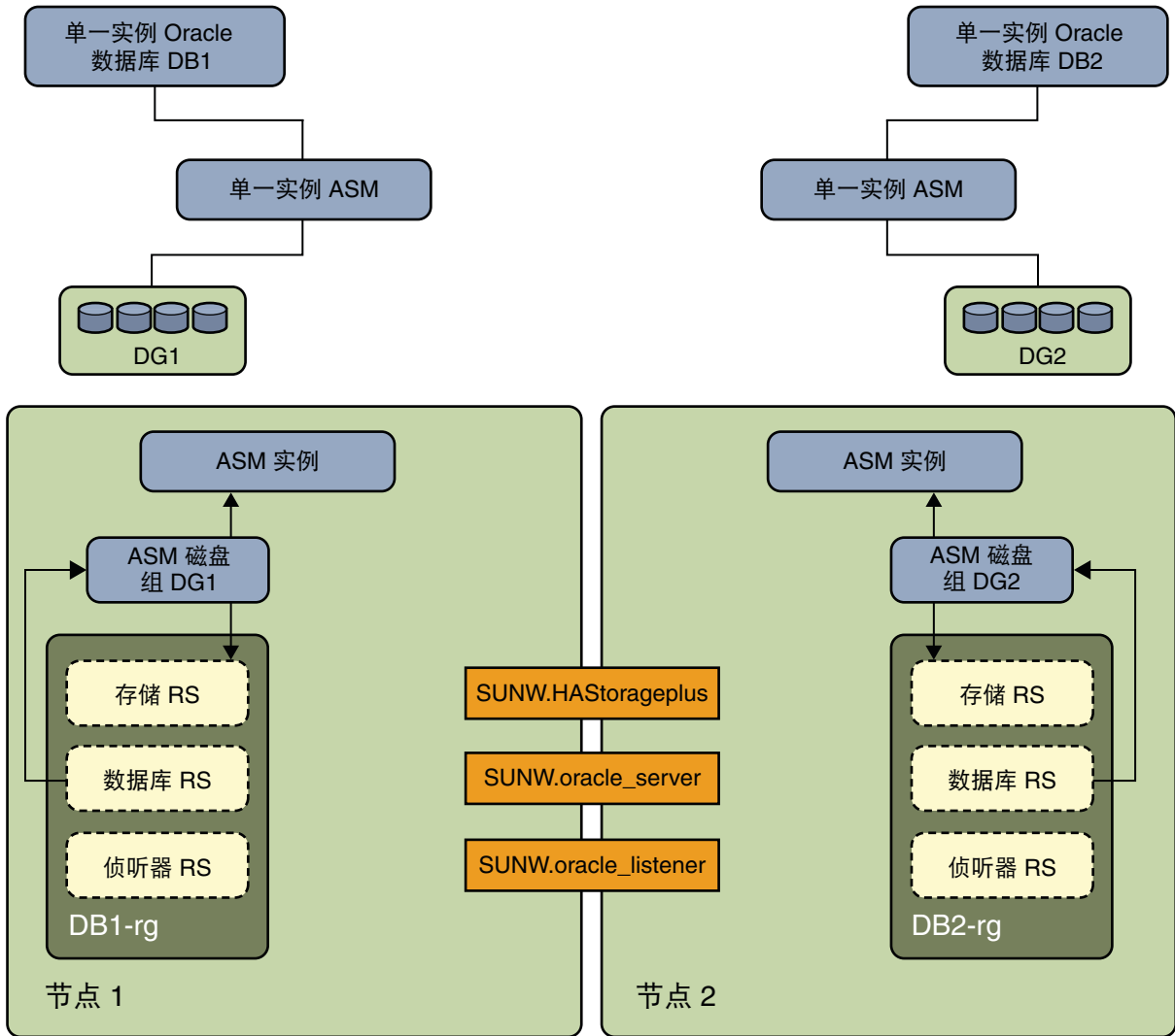
图 3 具有单独磁盘组的单实例 ASM [2]
