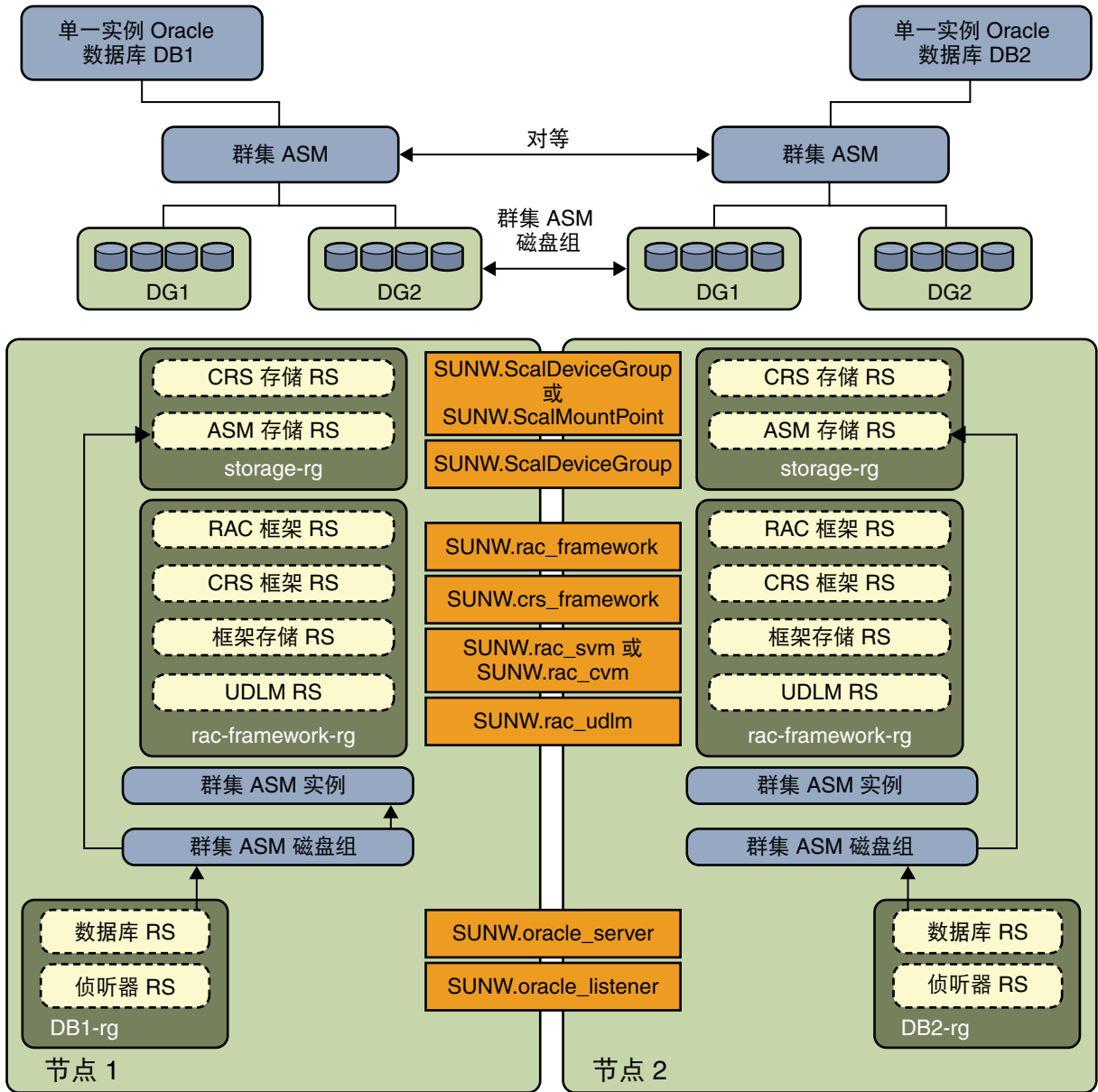
图 5 具有群集磁盘组的群集 ASM [2]
