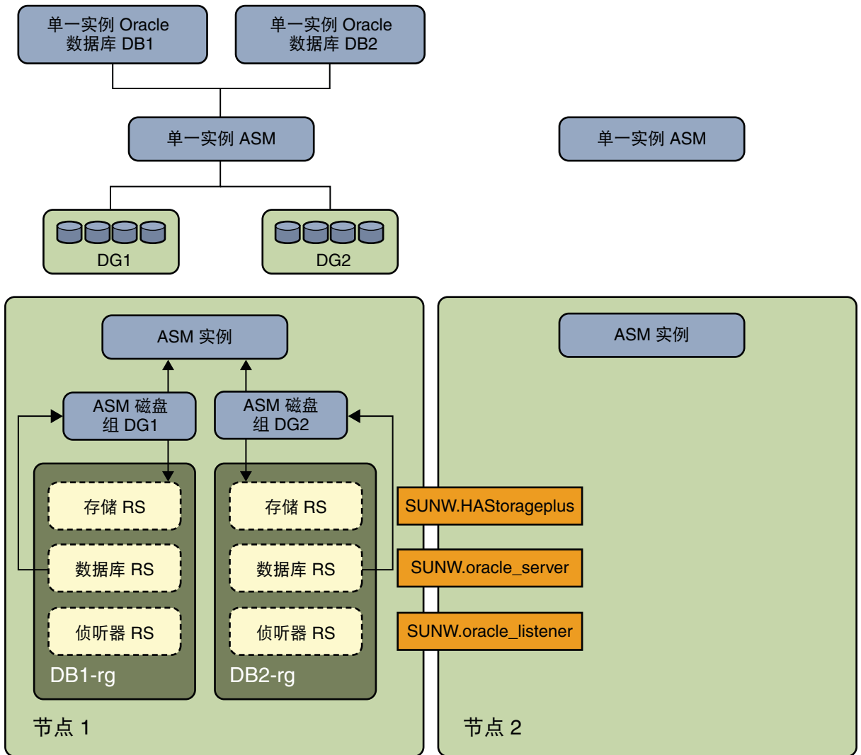
图2 具有单独磁盘组的单实例 ASM [1]
