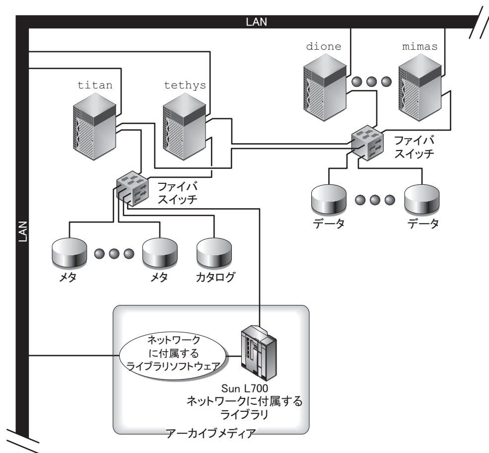
図 2-1 Sun StorEdge QFS 共有ファイルシステムの構成
