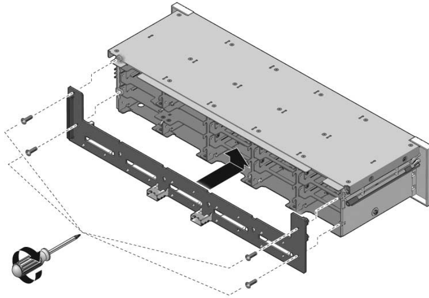
FIGURA 6-10 Installazione del backplane dei dischi rigidi (server Sun SPARC Enterprise T5220)
