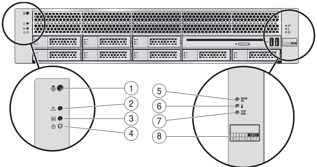
FIGURA 1-2 Accesso ai componenti del pannello anteriore (server Sun SPARC Enterprise T5220)
