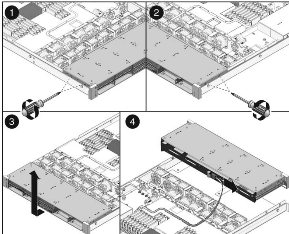
FIGURA 6-5 Rimozione dell'alloggiamento dei dischi rigidi (server Sun SPARC Enterprise T5120)
