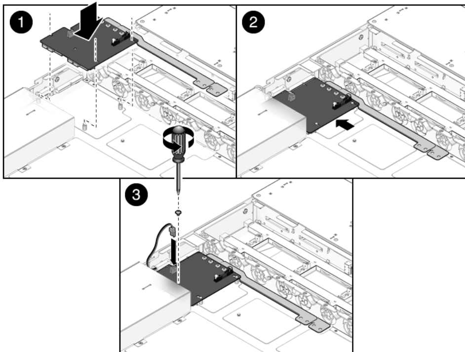
FIGURA 6-16 Installazione della scheda di distribuzione dell'alimentazione (server Sun SPARC Enterprise T5120)
