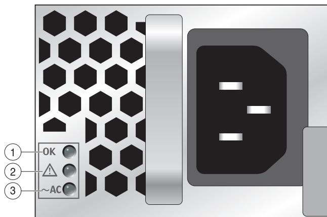
FIGURA 4-6 Spie di stato dell'alimentatore (server Sun SPARC Enterprise T5120)
