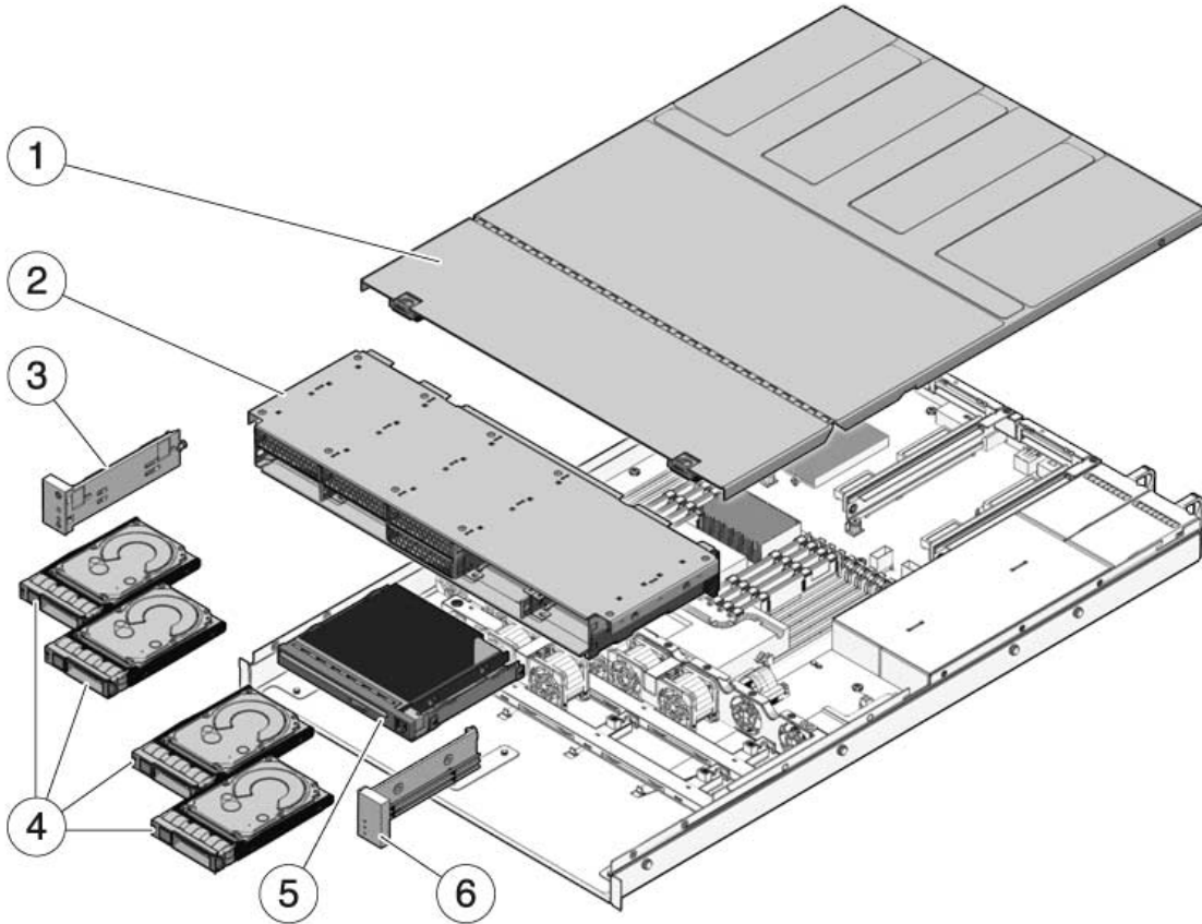
FIGURA A-1 Componenti di I/O (server Sun SPARC Enterprise T5120)
