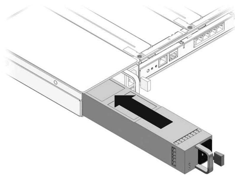
FIGURA 4-10 Installazione di un alimentatore (Sun SPARC Enterprise T5120)
