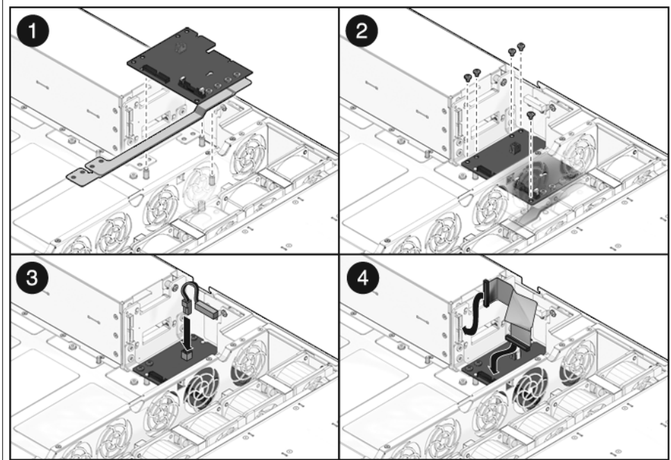
FIGURA 6-17 Installazione della scheda di distribuzione dell'alimentazione (server Sun SPARC Enterprise T5220)
