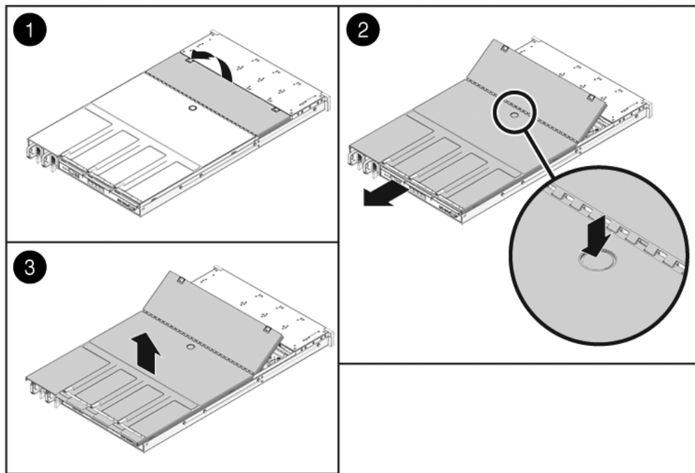
FIGURA 3-4 Rimozione della copertura superiore (server Sun SPARC Enterprise T5120)
