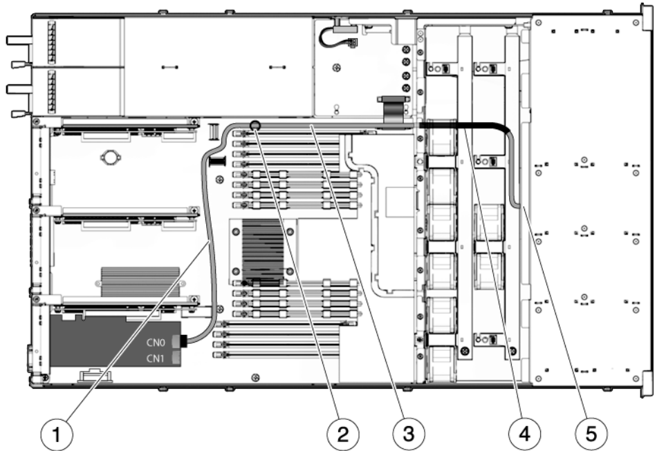
FIGURA A-7 (Server Sun SPARC Enterprise T5120, con quattro dischi) Cavi dal controller PCIe al backplane dei dischi
