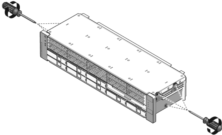
FIGURA 6-11 Rimozione del gruppo luminoso del pannello di controllo anteriore (Sun SPARC Enterprise T5220)
