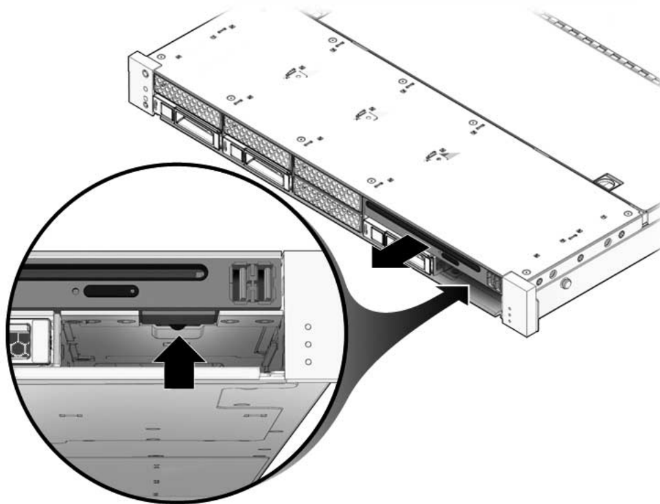
FIGURA 6-1 Rimozione del modulo DVD/USB (Sun SPARC Enterprise T5120)
