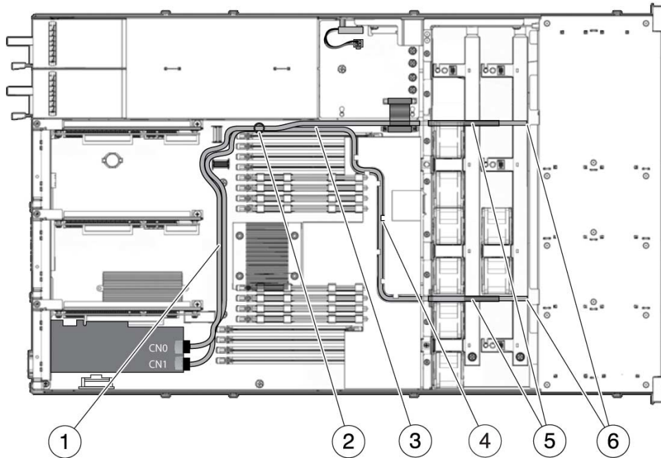
FIGURA A-8 (Server Sun SPARC Enterprise T5120, con otto dischi) Cavi dal controller PCIe al backplane dei dischi
