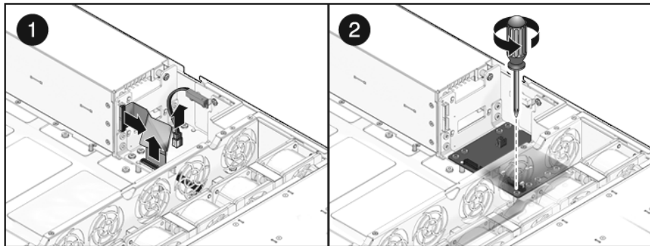
FIGURA 6-14 Rimozione della scheda di distribuzione dell'alimentazione (server Sun SPARC Enterprise T5220)
