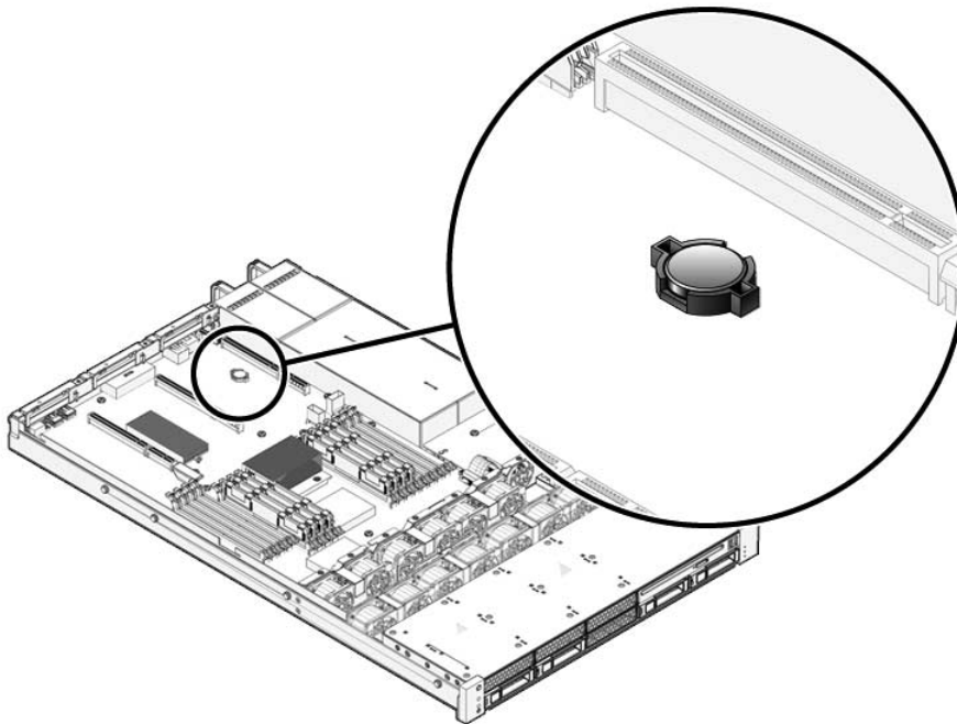
FIGURA 5-10 Posizione della batteria (server Sun SPARC Enterprise T5120)
