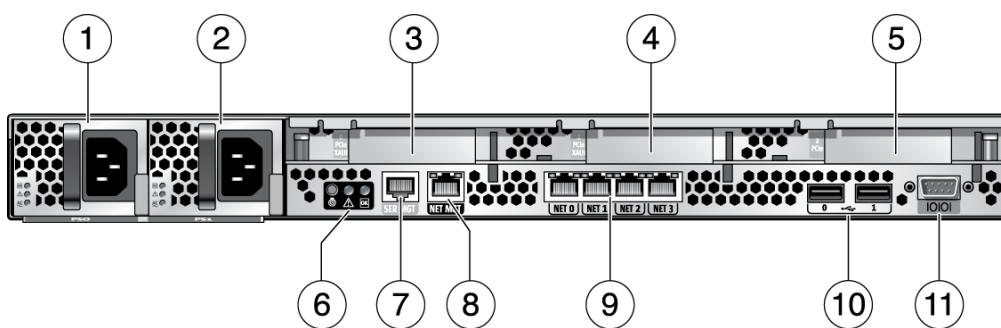
FIGURA 1-3 Accesso ai componenti del pannello posteriore (server Sun SPARC Enterprise T5120)
