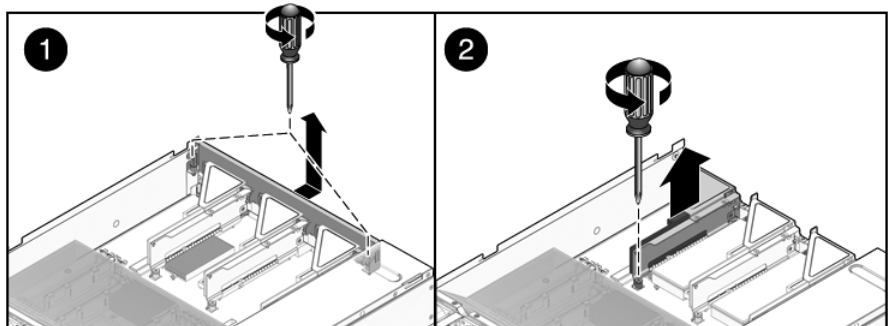
FIGURA 5-5 Rimozione della scheda di espansione PCIe/XAUI (Sun SPARC Enterprise T5220)
