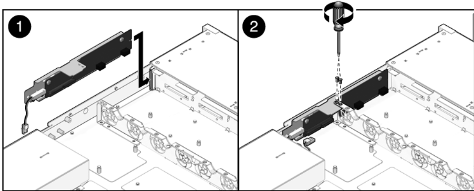
FIGURA 6-24 Installazione della scheda paddle (server Sun SPARC Enterprise T5120)
