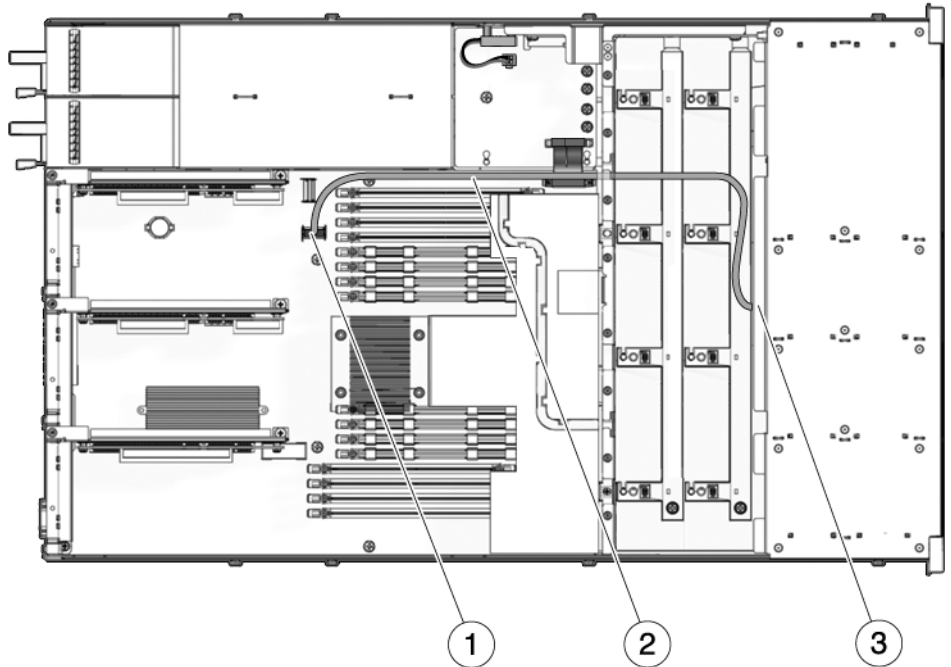
FIGURA A-5 (Server Sun SPARC Enterprise T5120, con quattro dischi) Cavi dal controller SAS al backplane dei dischi
