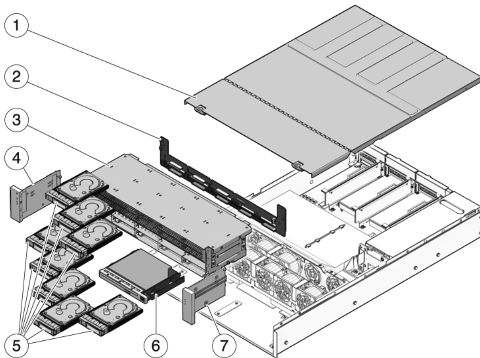
FIGURA A-9 Componenti di I/O (server Sun SPARC Enterprise T5220)
