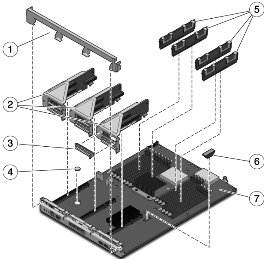
FIGURA A-10 Componenti della scheda madre (Sun SPARC Enterprise T5220)
