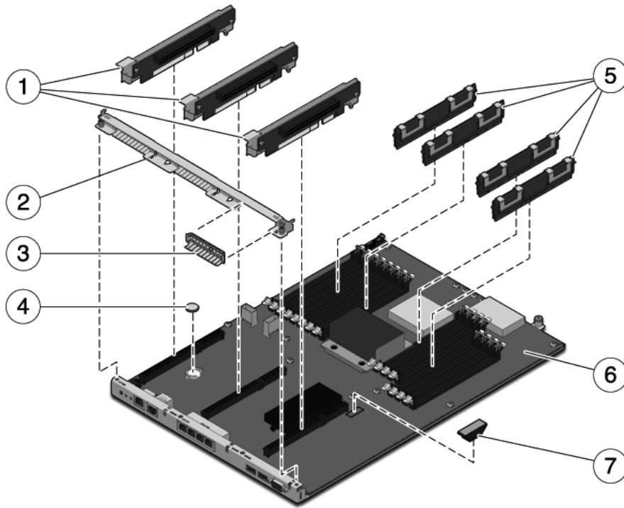
FIGURA A-2 Componenti della scheda madre (Sun SPARC Enterprise T5120)
