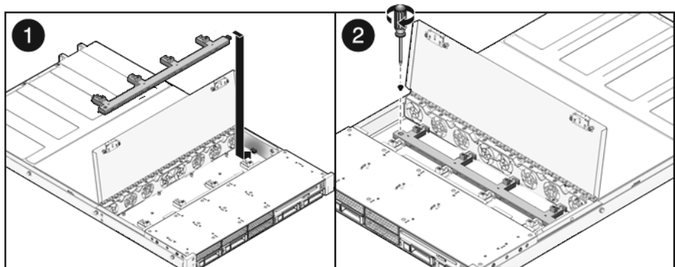
FIGURA 6-4 Installazione di una scheda di alimentazione delle ventole (server Sun SPARC Enterprise T5120)
