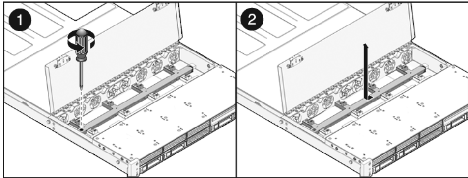
FIGURA 6-3 Rimozione della scheda di alimentazione delle ventole (Sun SPARC Enterprise T5120)
