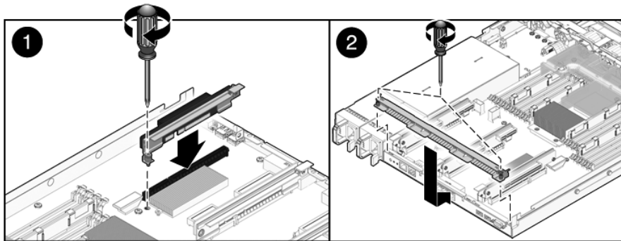
FIGURA 5-6 Installazione della scheda di espansione PCIe/XAUI (Sun SPARC Enterprise T5120)
