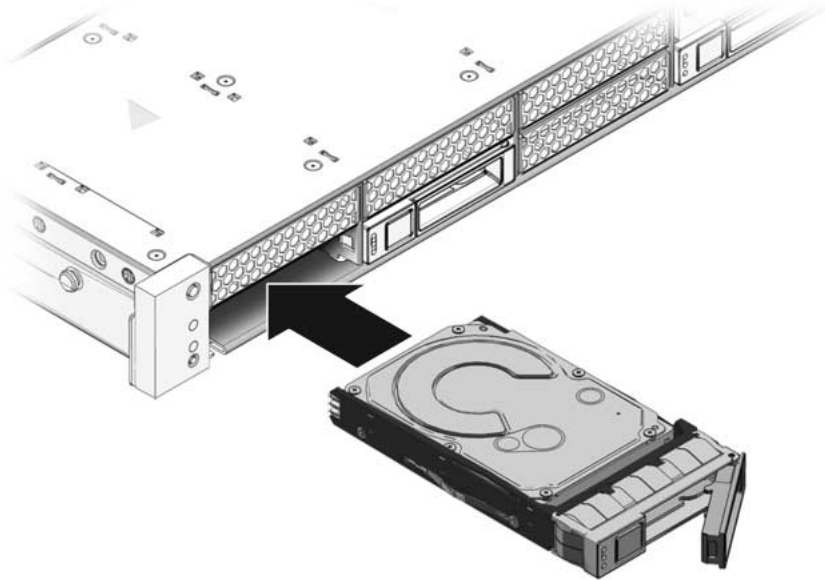
FIGURA 4-3 Installazione di un disco rigido (server Sun SPARC Enterprise T5220)
