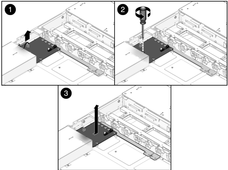
FIGURA 6-15 Rimozione della scheda di distribuzione dell'alimentazione (server Sun SPARC Enterprise T5120)
