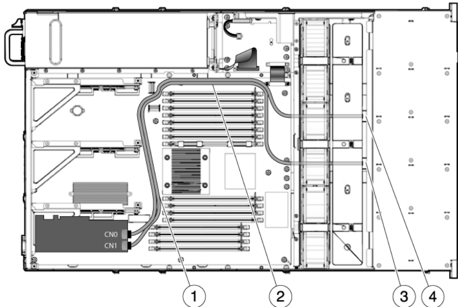
FIGURA A-14 (Server Sun SPARC Enterprise T5220) Cavi dal controller PCIe al backplane dei dischi rigidi
