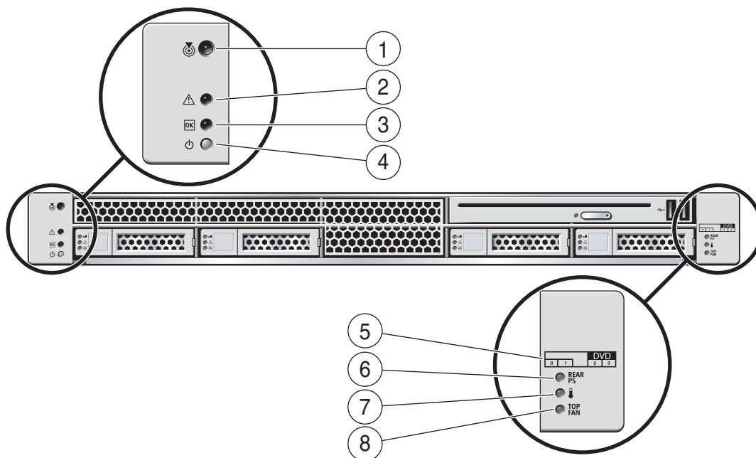
FIGURA 1-1 Accesso ai componenti del pannello anteriore (server Sun SPARC Enterprise T5120)
