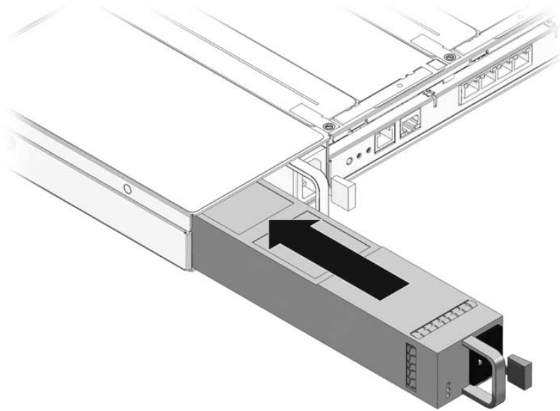
FIGURA 6-18 Installazione di un alimentatore (server Sun SPARC Enterprise T5120)
