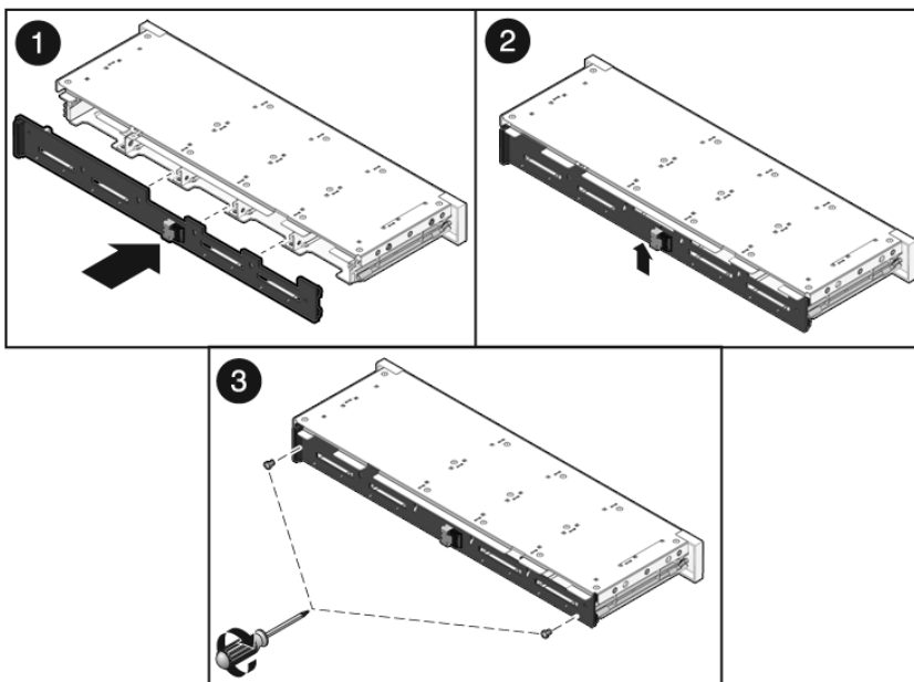
FIGURA 6-9 Installazione del backplane dei dischi rigidi (server Sun SPARC Enterprise T5120)
