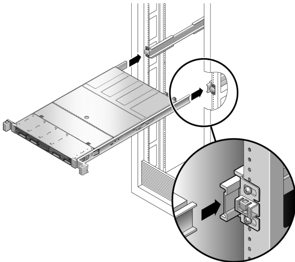
FIGURA 7-2 Reinserimento del server nel rack (server Sun SPARC Enterprise T5120)
