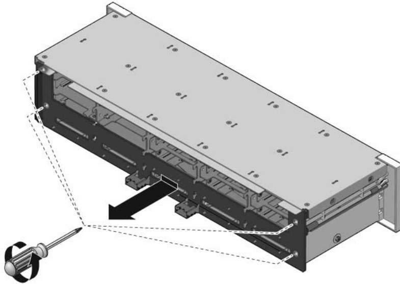
FIGURA 6-8 Rimozione del backplane dei dischi rigidi (server Sun SPARC Enterprise T5220)
