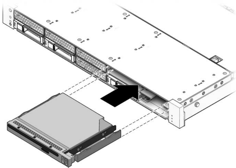
FIGURA 6-2 Installazione del modulo DVD/USB (Sun SPARC Enterprise T5120)
