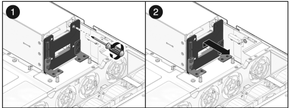
FIGURA 6-20 Rimozione del backplane degli alimentatori (server Sun SPARC Enterprise T5220)
