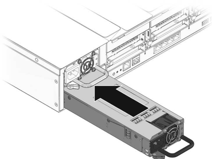
FIGURA 6-22 Installazione di un alimentatore (server Sun SPARC Enterprise T5220)
