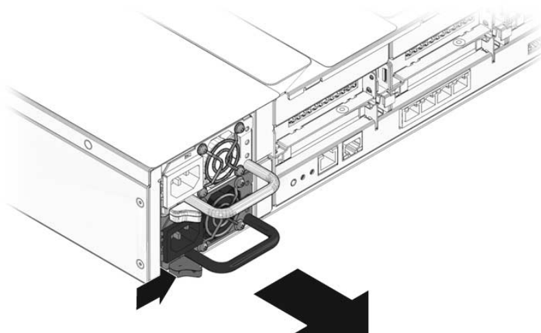
FIGURA 4-9 Impugnatura di estrazione dell'alimentatore (Sun SPARC Enterprise T5220)
