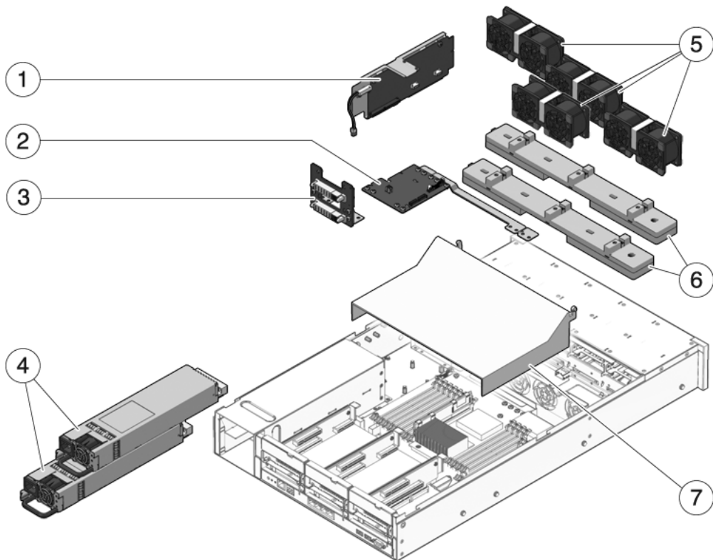
FIGURA A-11 Componenti del modulo di distribuzione dell'alimentazione e del modulo ventole (server Sun SPARC Enterprise T5220)
