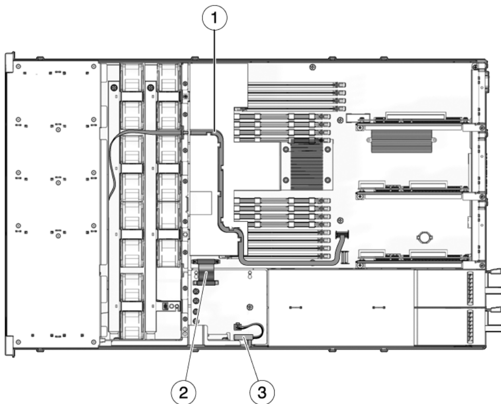
FIGURA A-4 Cavi (server Sun SPARC Enterprise T5120)
