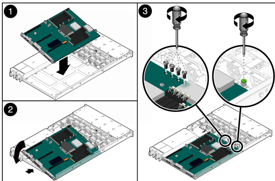
FIGURA 5-12 Installazione della scheda madre (server Sun SPARC Enterprise T5120)
