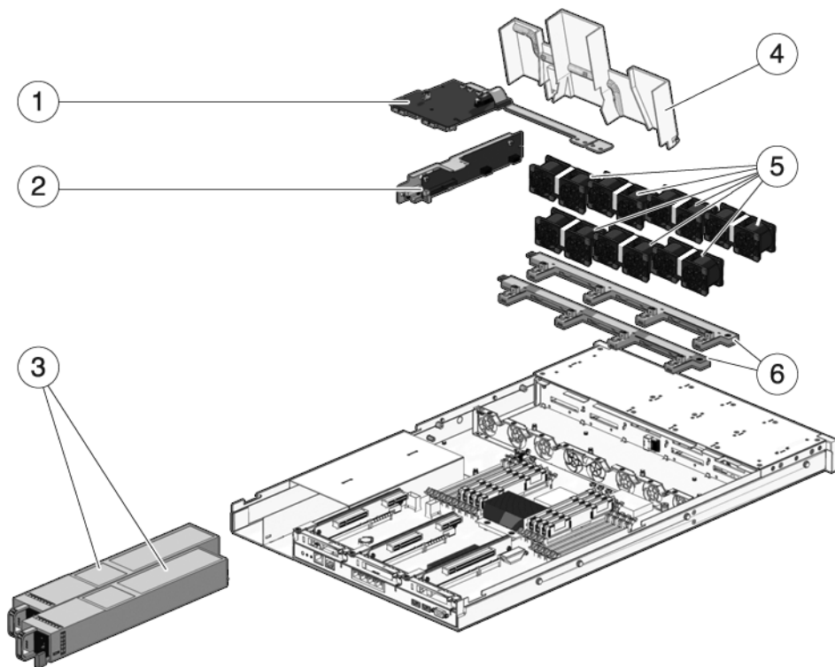
FIGURA A-3 Componenti del modulo di distribuzione dell'alimentazione e del modulo ventole (server Sun SPARC Enterprise T5120)
