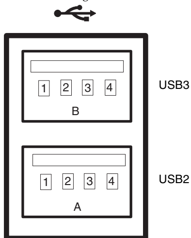
FIGURA B-4 Diagramma del connettore USB
