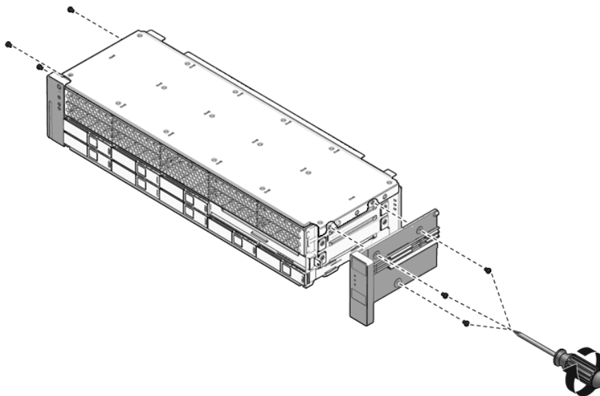
FIGURA 6-12 Installazione del gruppo luminoso del pannello di controllo anteriore (server Sun SPARC Enterprise T5220)
