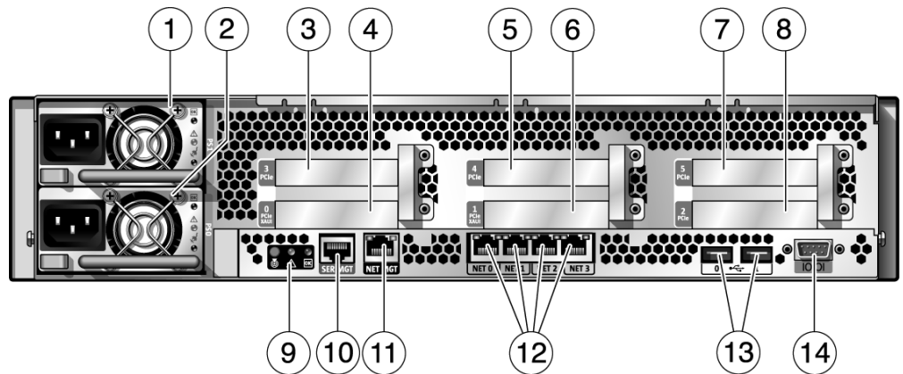
FIGURA 1-4 Accesso ai componenti del pannello posteriore (server Sun SPARC Enterprise T5220)
