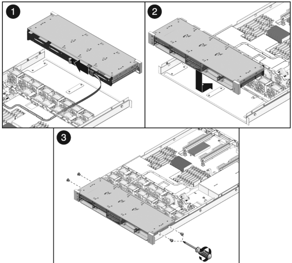
FIGURA 6-6 Installazione dell'alloggiamento dei dischi rigidi (server Sun SPARC Enterprise T5120)
