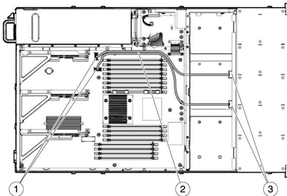
FIGURA A-13 (Server Sun SPARC Enterprise T5220) Cavi dal controller SAS integrato al backplane dei dischi rigidi
