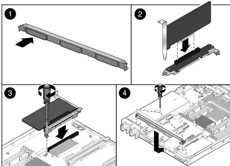
FIGURA 5-8 Installazione di una scheda PCIe (Sun SPARC Enterprise T5120)
