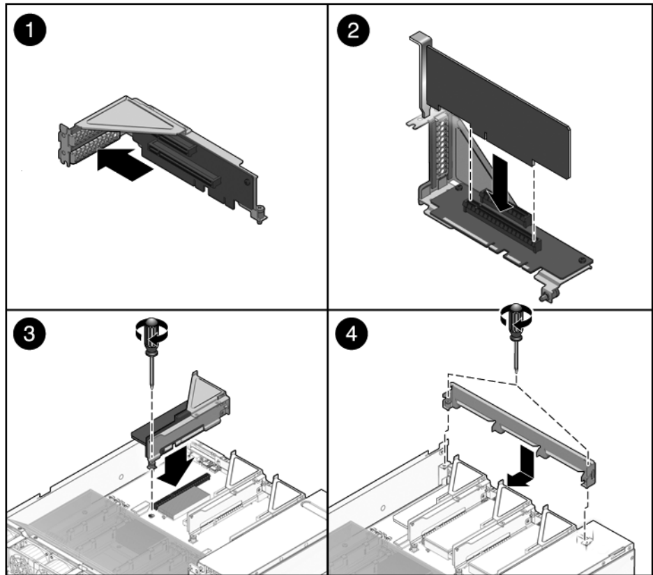
FIGURA 5-9 Installazione di una scheda PCIe (Sun SPARC Enterprise T5220)
