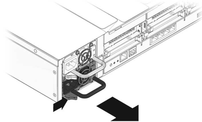
FIGURA 6-19 Rimozione di un alimentatore (server Sun SPARC Enterprise T5220)
