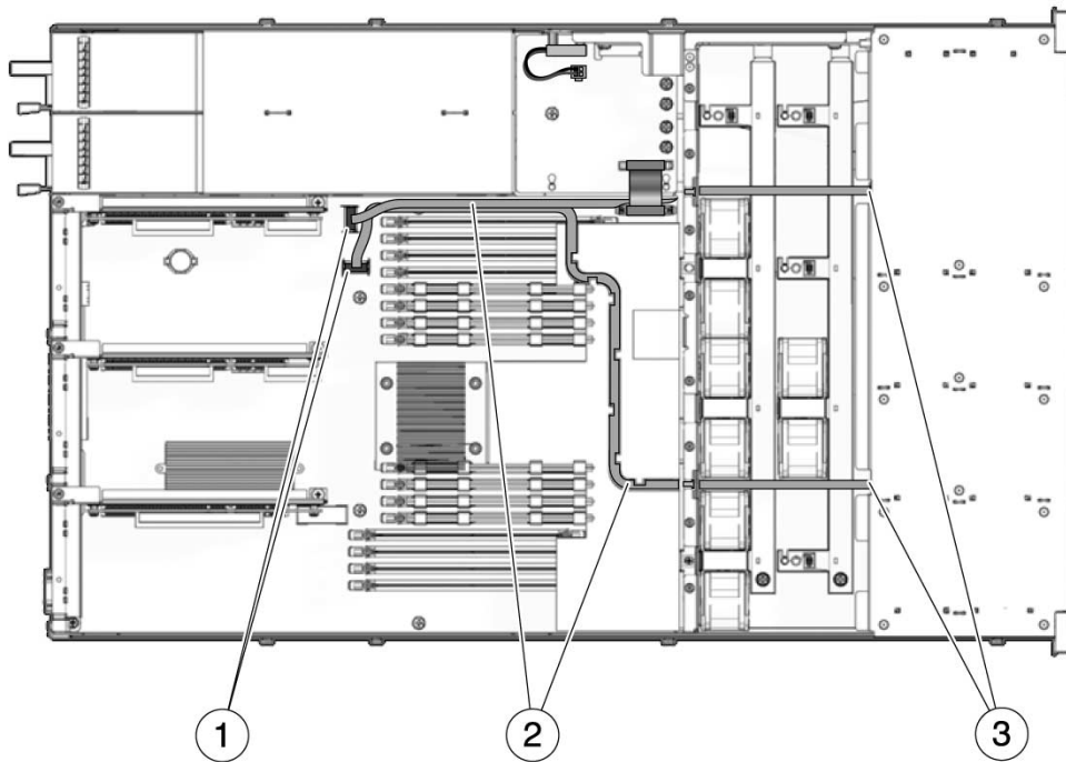
FIGURA A-6 (Server Sun SPARC Enterprise T5120, con otto dischi) Cavi dal controller SAS al backplane dei dischi
