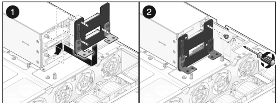
FIGURA 6-21 Installazione del backplane degli alimentatori (server Sun SPARC Enterprise T5220)
