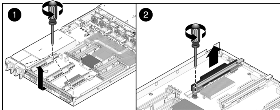
FIGURA 5-4 Rimozione della scheda di espansione PCIe/XAUI (Sun SPARC Enterprise T5120)
