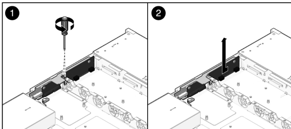
FIGURA 6-23 Rimozione della scheda paddle (server Sun SPARC Enterprise T5120)
