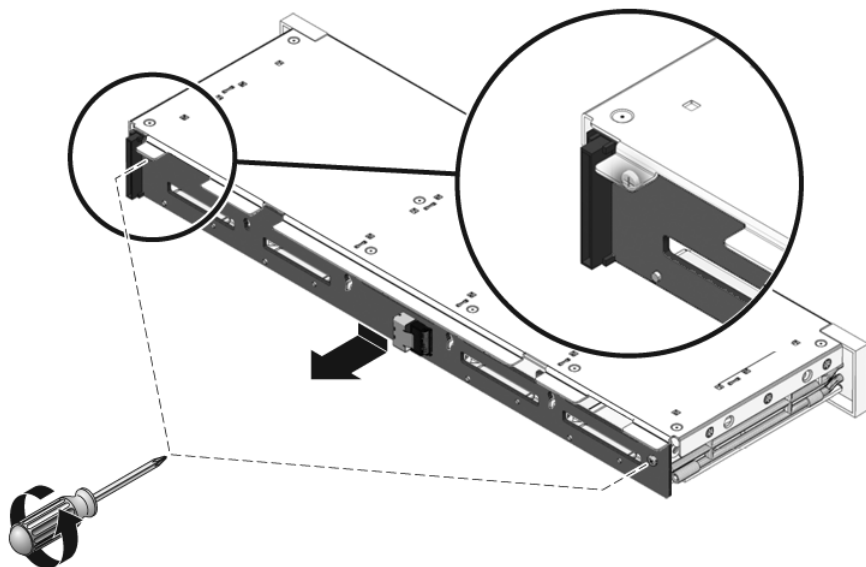
FIGURA 6-7 Rimozione del backplane dei dischi rigidi (server Sun SPARC Enterprise T5120)
