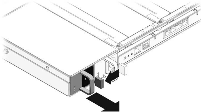
FIGURA 6-13 Rimozione di un alimentatore (server Sun SPARC Enterprise T5120)
