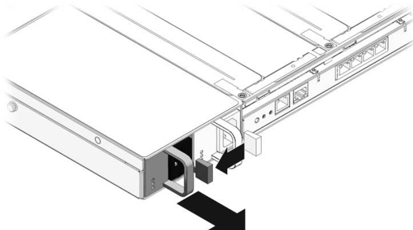
FIGURA 4-9 Impugnatura di estrazione dell'alimentatore (Sun SPARC Enterprise T5220)
