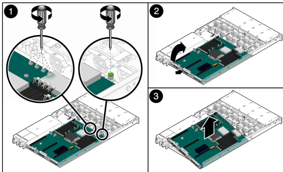
FIGURA 5-11 Rimozione della scheda madre (server Sun SPARC Enterprise T5120)
