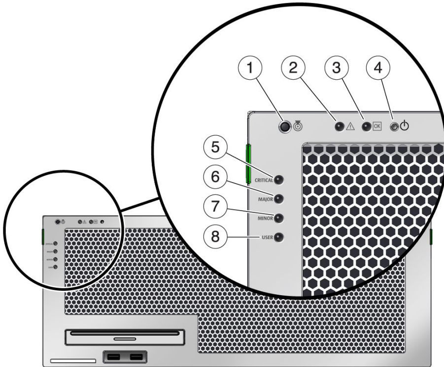
圖 2-1 擋板伺服器狀態與警報狀態指示燈的位置
