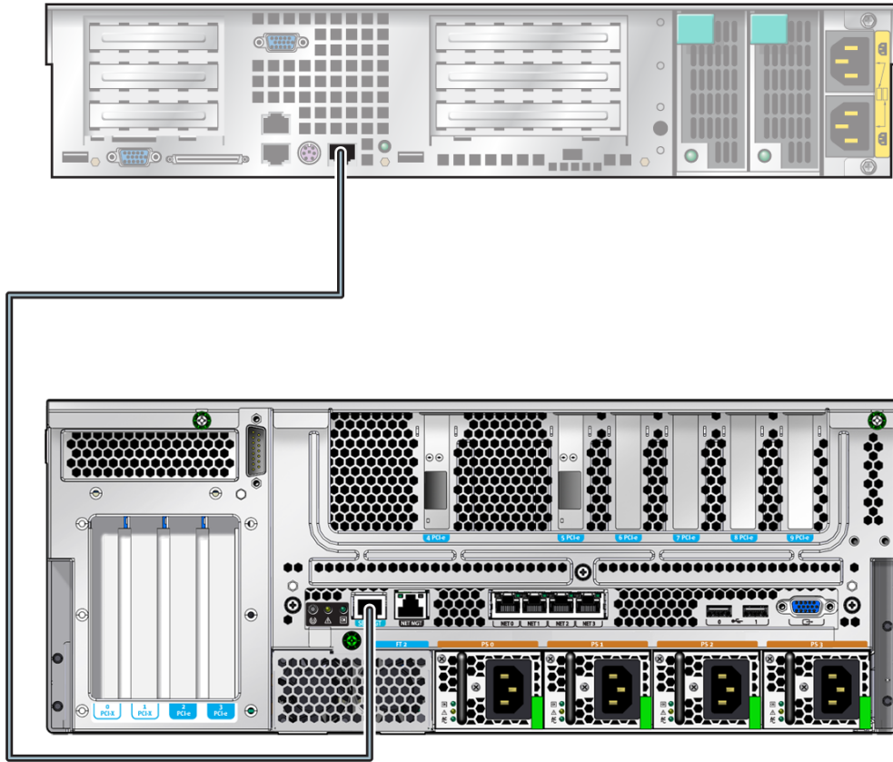
圖 1-4 Sun Netra T5440 伺服器與另一個系統之間的 Tip 連線
