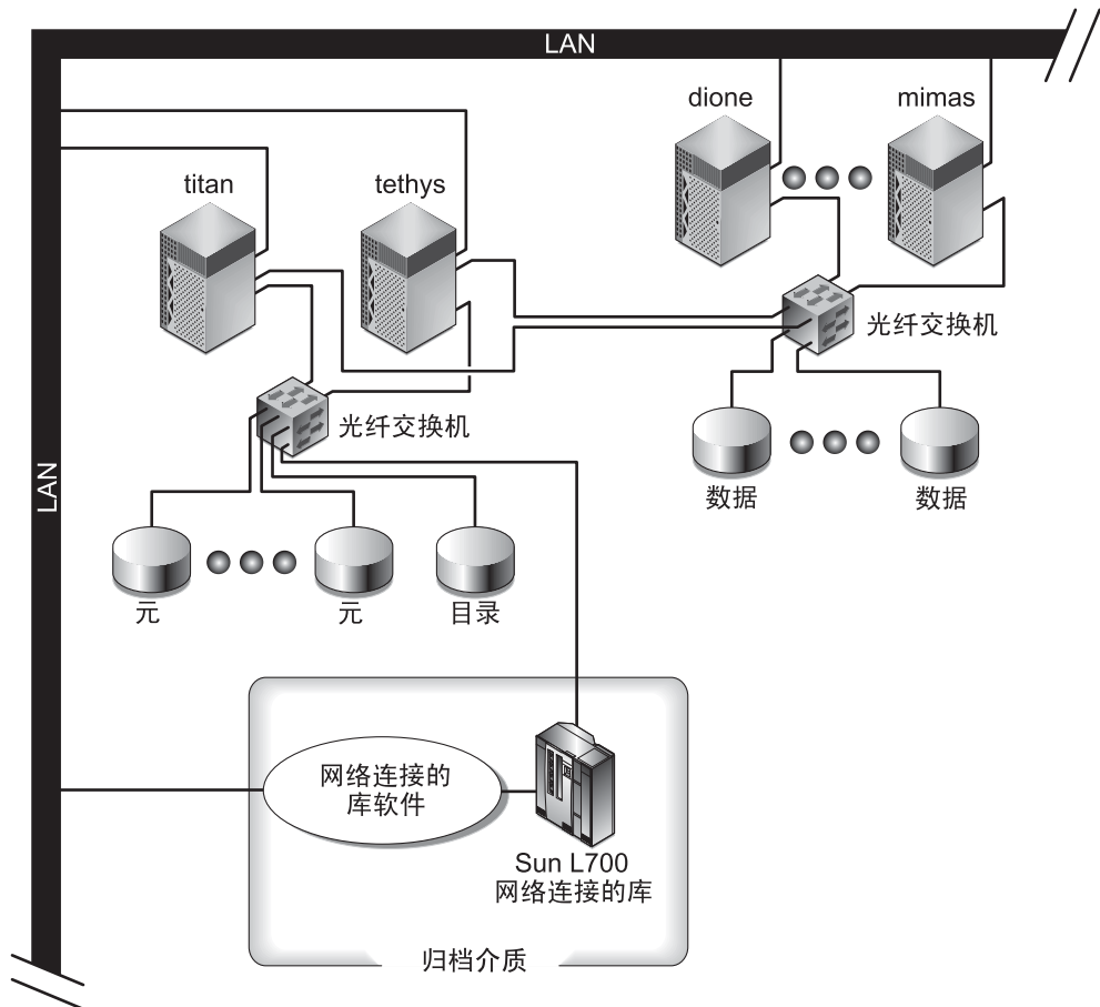
图 D-1 共享的 Sun SAM-QFS 环境。显示连接到 LAN 的主机 titan 、 tethys 、 dione 和 mimas 。 Sun L700 库连接到 LAN、 titan 和 tethys 。
