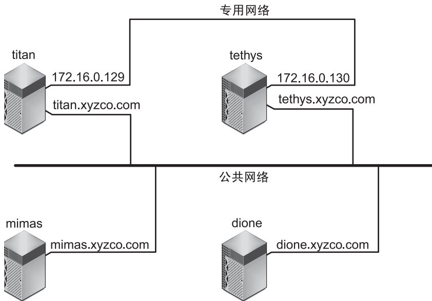
图 4-1 网络接口
