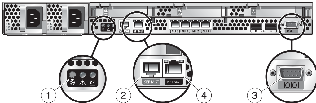
圖 1-2 Sun SPARC Enterprise T5140 機殼的後方 I/O 面板
