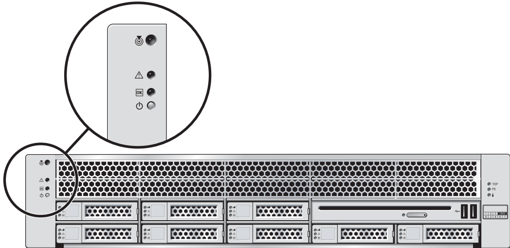
圖 2-2 Sun SPARC Enterprise T5240 機殼上的定位器按鈕 (上方按鈕)
