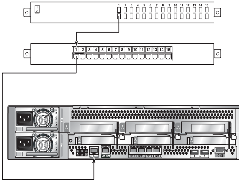
圖 1-4 終端機伺服器與 Sun SPARC Enterprise T5140 或 T5240 伺服器之間的控制面板連線
