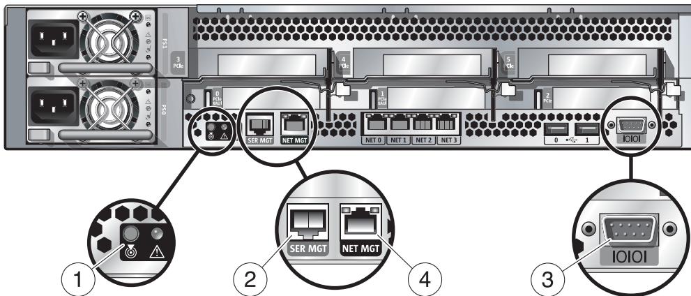
圖 1-3 Sun SPARC Enterprise T5240 機殼的後方 I/O 面板
