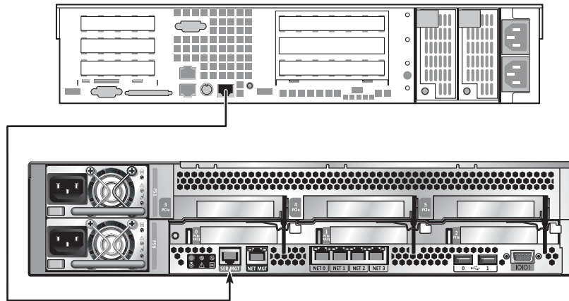
圖 1-5 Sun SPARC Enterprise T5140 或 T5240 伺服器與另一個系統之間的 Tip 連線
