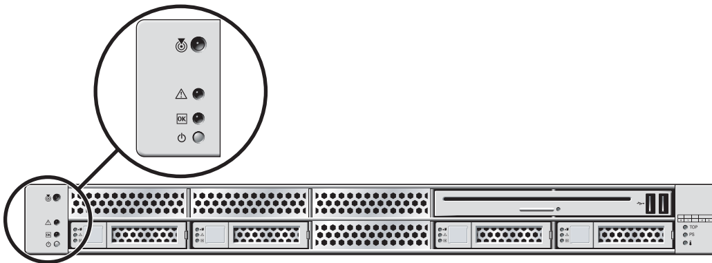
圖 2-1 Sun SPARC Enterprise T5140 機殼上的定位器按鈕 (上方按鈕)
