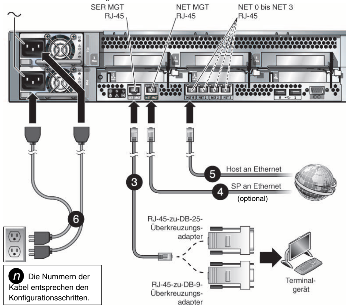
ABBILDUNG 2 Serververbindungen
