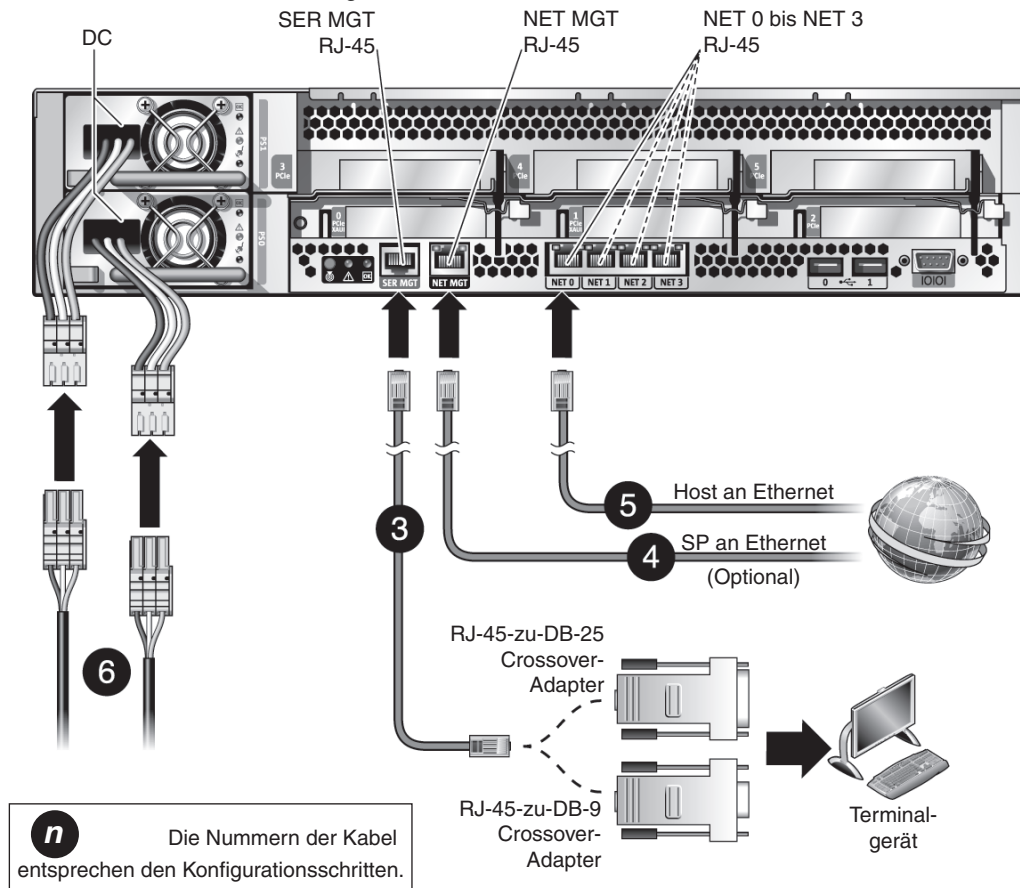
ABBILDUNG 2 Serververbindungen
