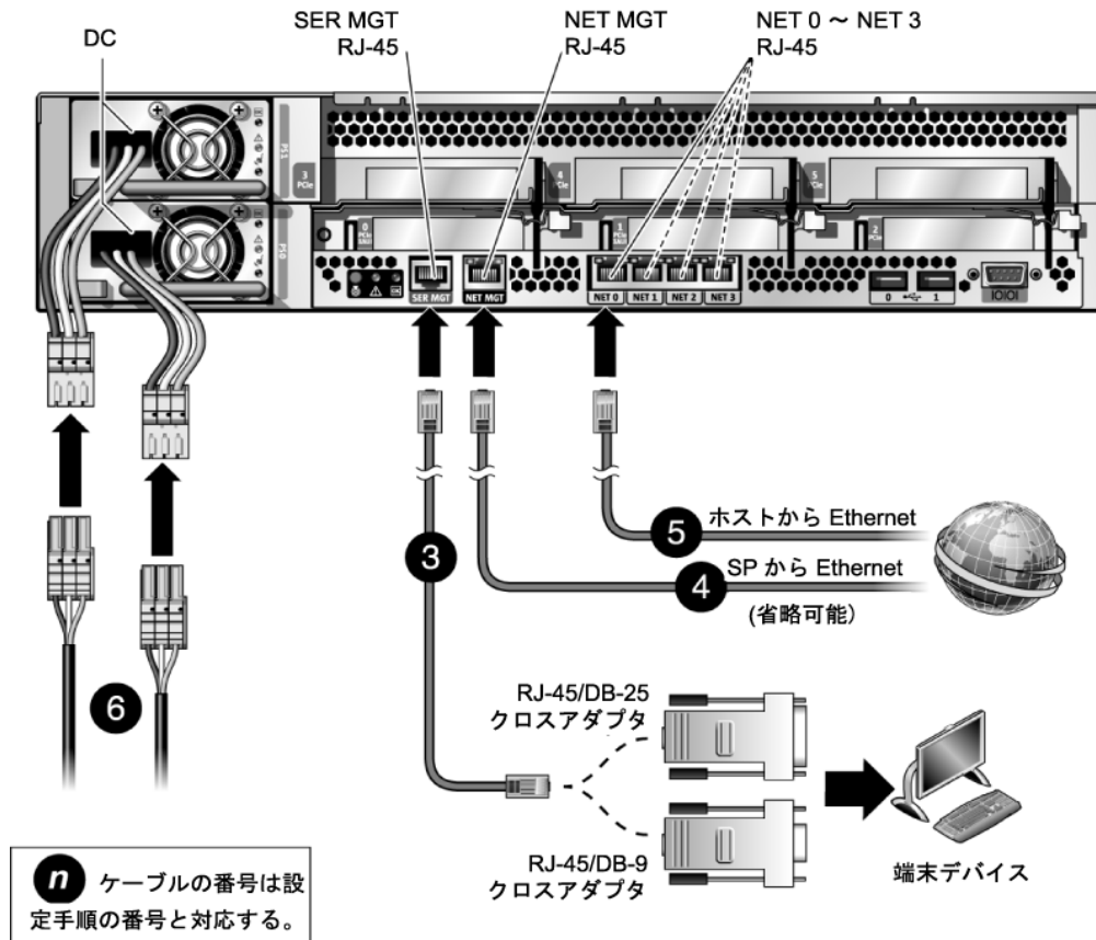
図 2 サーバの接続
