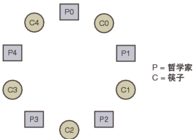
图 3-1 哲学家就餐
