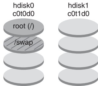
ABBILDUNG 9-2 Festplattenlayout für ein RAID-1-Volume
