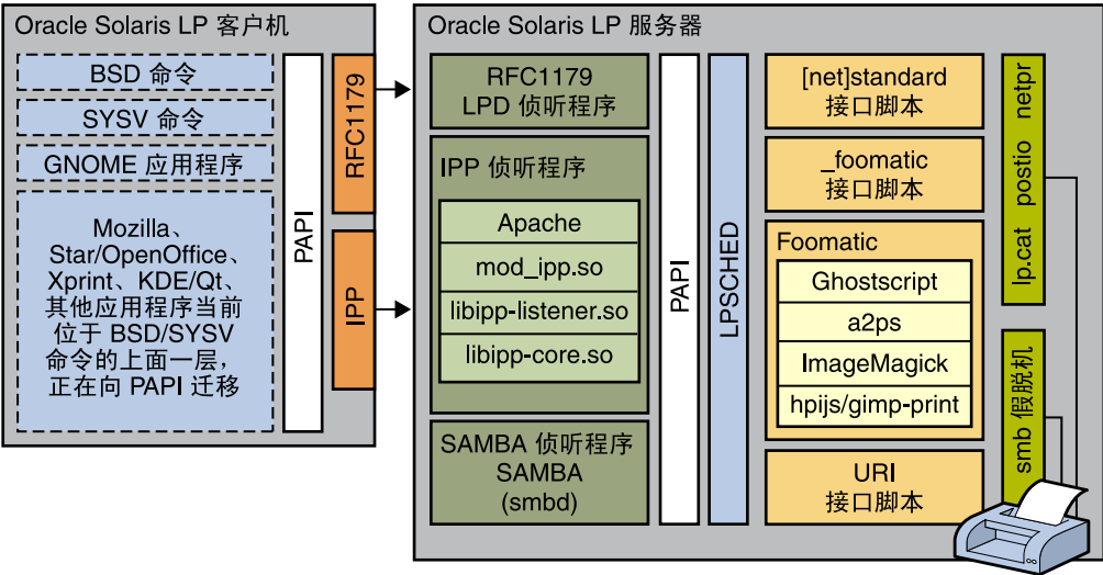
图 1-1 行式打印机 (Line Printer, LP) 客户机/服务器关系
