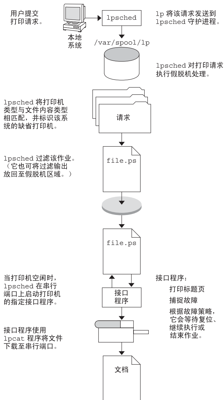
图 1-6 LP 打印服务打印调度过程
