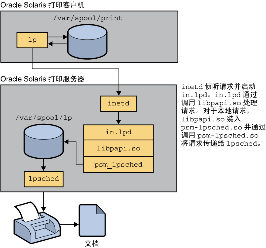
图 1-9 如何处理打印请求
