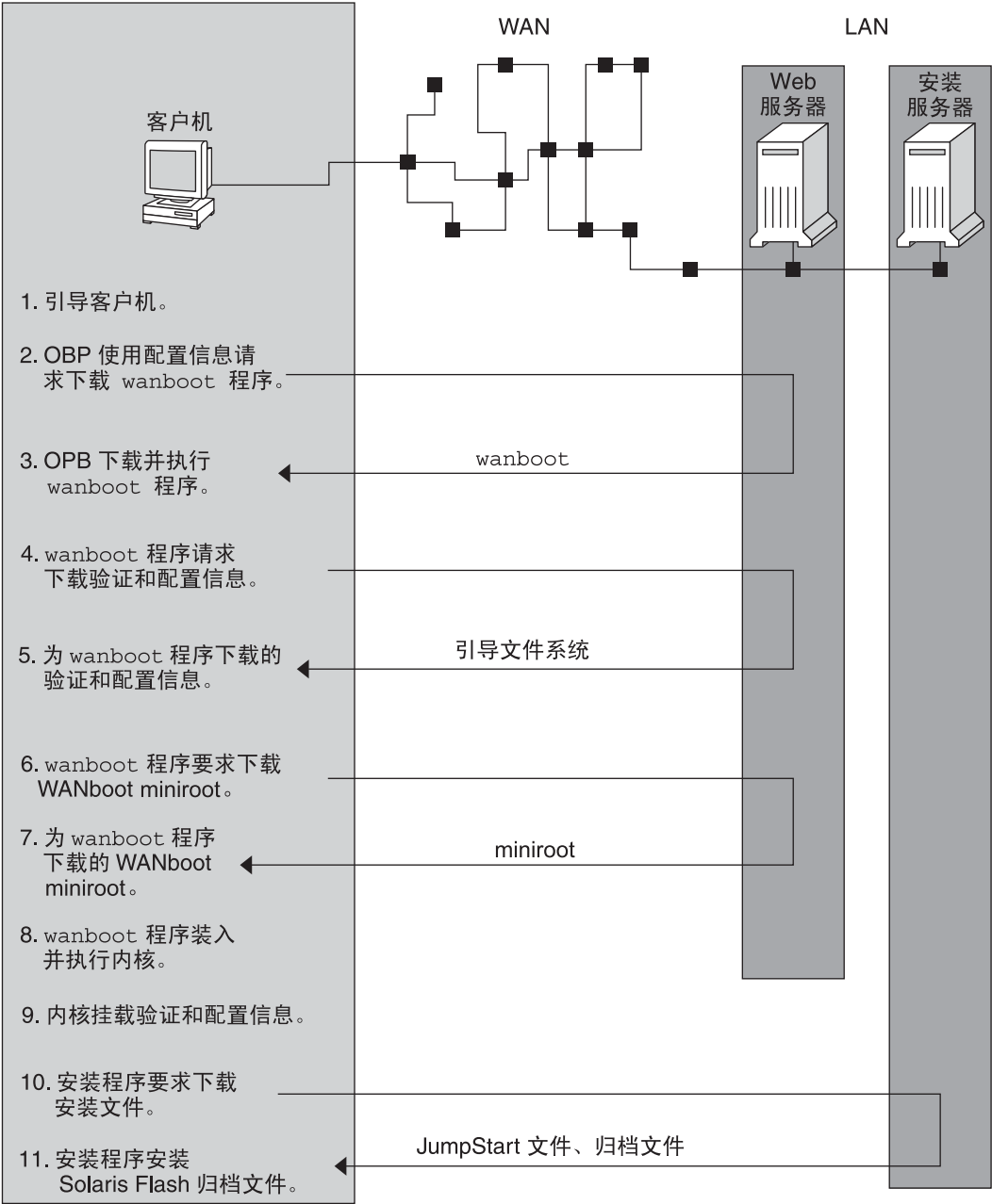
图 10-1 WAN Boot 安装中的事件序列
