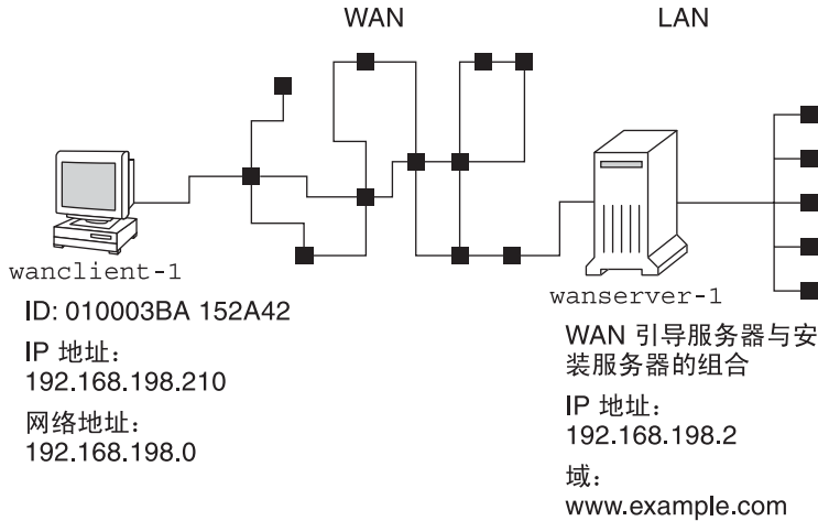
图 14-1 WAN Boot 安装的样例站点
