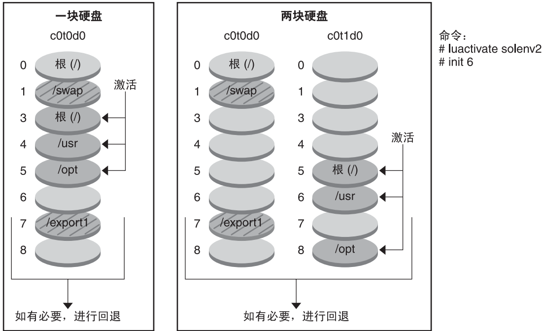
图 2-10 激活非活动的引导环境
