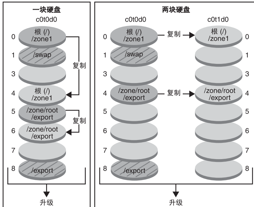
图 8-2 创建引导环境—从非全局区域复制共享文件系统
