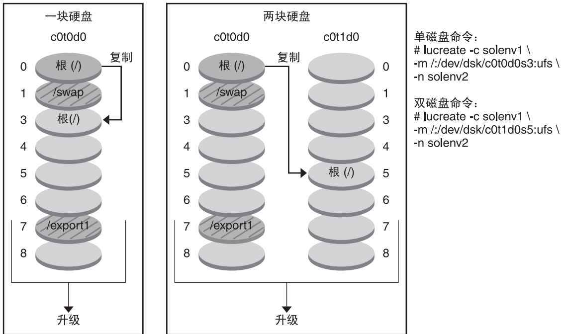
图 2-2 创建非活动的引导环境—复制根 (/) 文件系统
