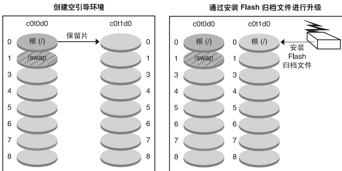
图 2-9 在双磁盘上安装 Solaris Flash 归档文件
