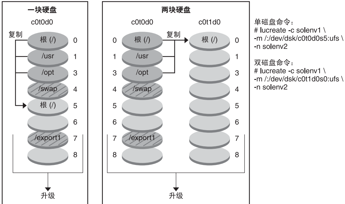
图 2-4 创建非活动的引导环境—合并文件系统
