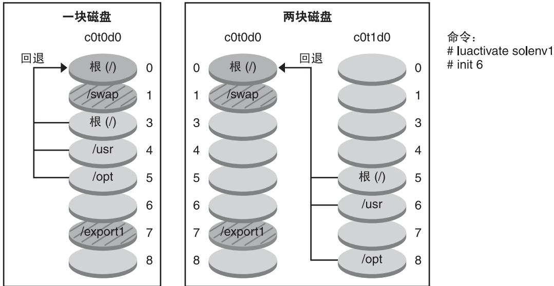
图 2-11 回退到初始引导环境
