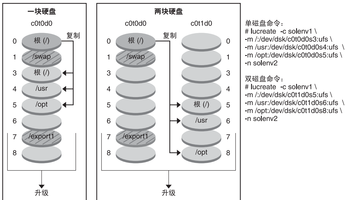
图 2-3 创建非活动的引导环境 – 拆分文件系统
