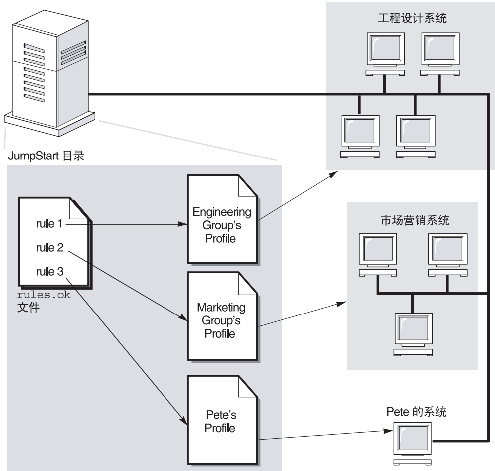
图 2-3 说明了 JumpStart 程序搜索定制 JumpStart 文件的顺序。
