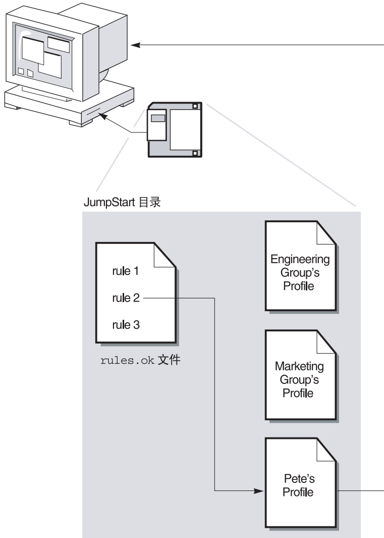
图 2-1 定制 JumpStart 安装的工作原理：非联网示例
