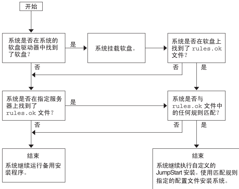
图 2-3 定制 JumpStart 安装过程中执行的操作
