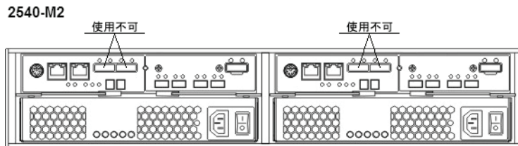
図 1 2540-M2 の SAS ホストポート
