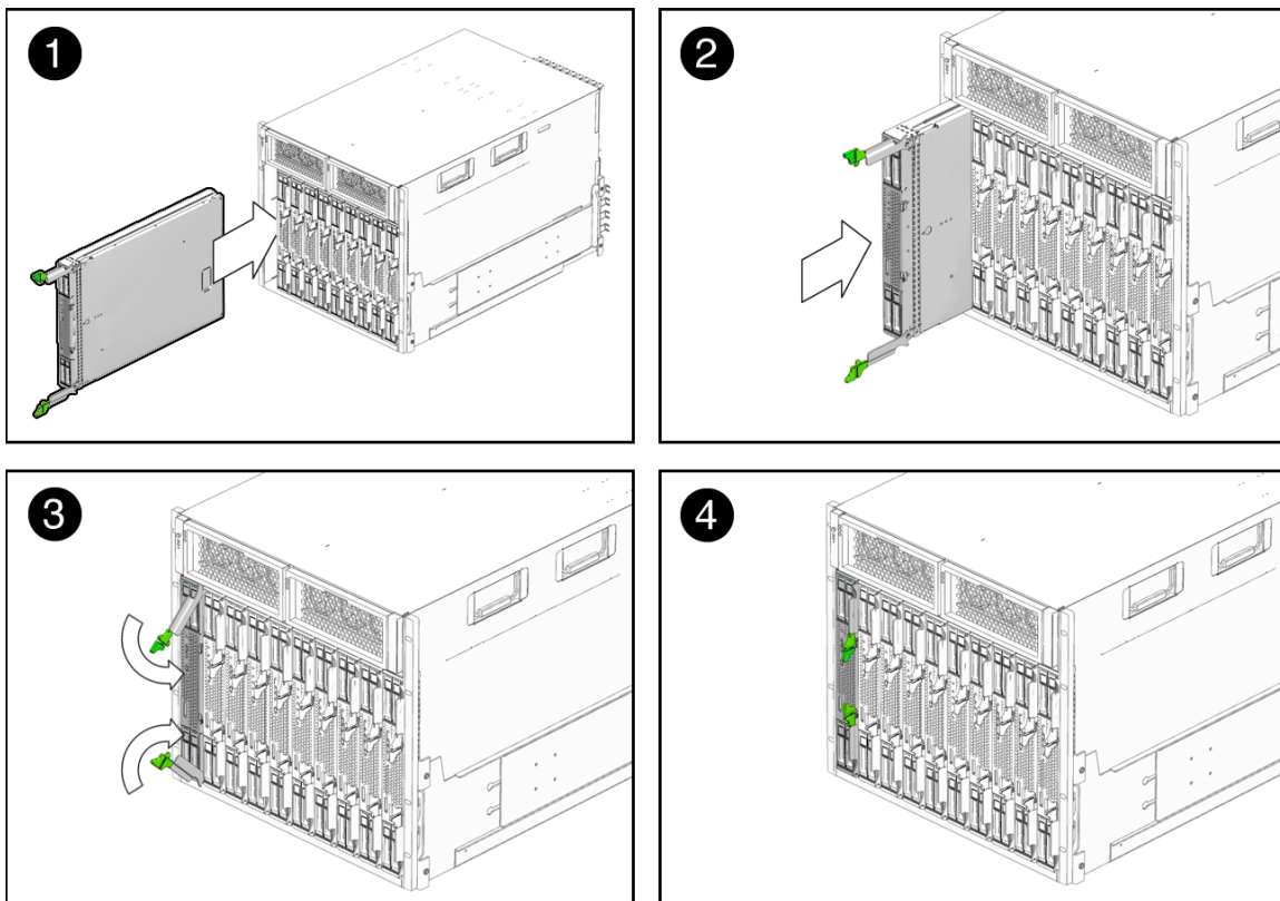
図 2-2 サーバーモジュールのシャーシへの挿入
