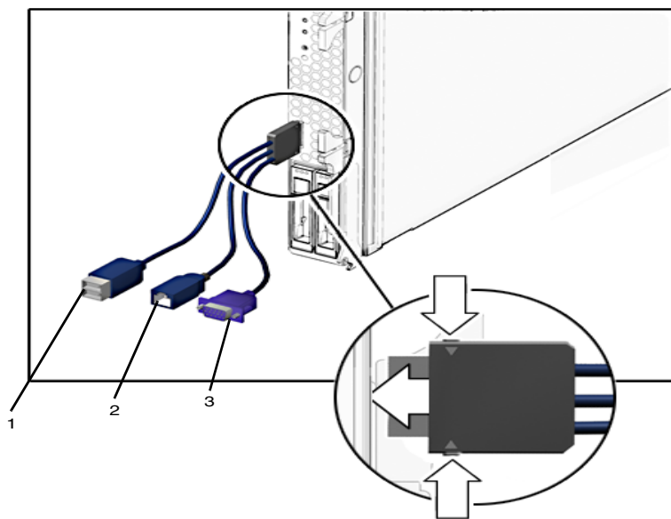
図 2-3 ドングルケーブルの接続
