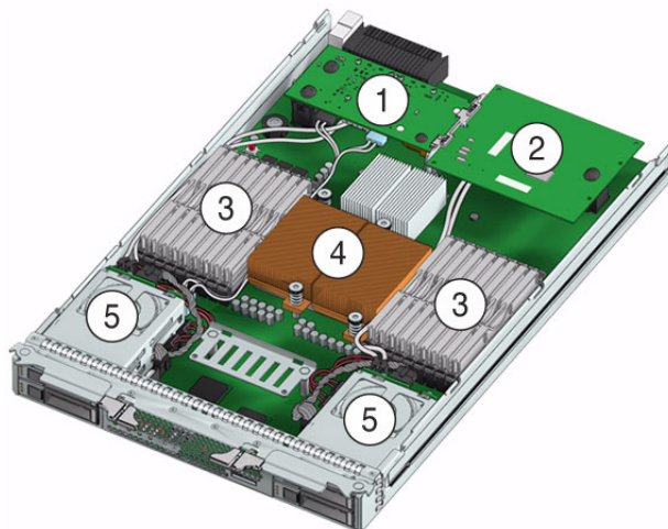
図 1-1 オプションコンポーネントのサーバーモジュール内の位置
