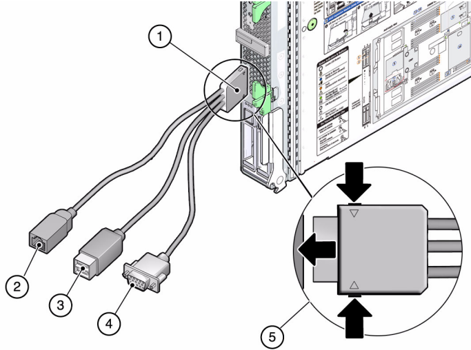
그림: 커넥터가 3개인 UCP-3 동글 케이블
