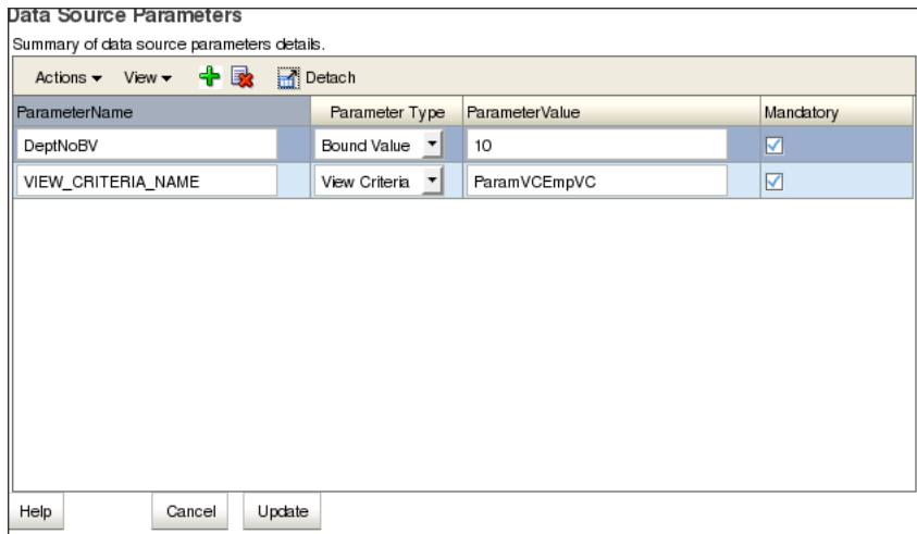
Figure 19–6 Parameters in Data Source Parameter UI
