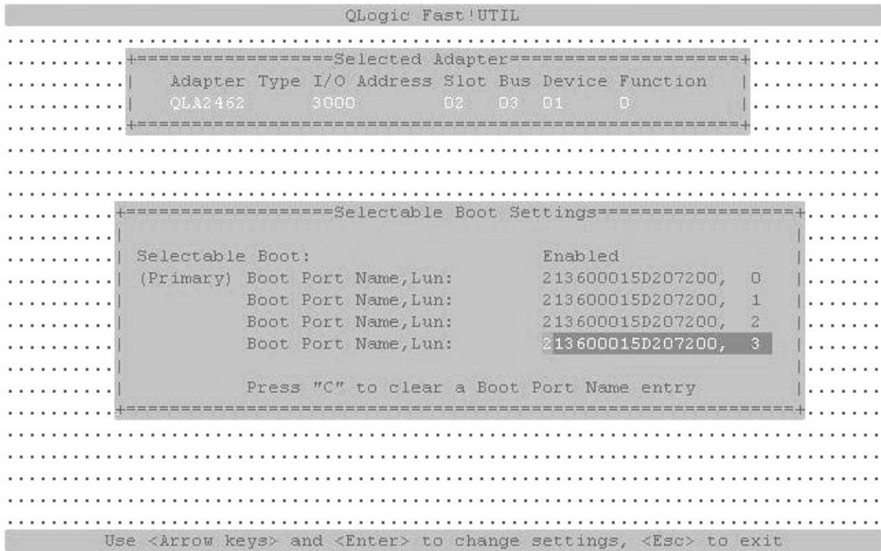
FIGURA 11-3 Pantalla de BIOS de HBA para activar el inicio desde el LUN FC
