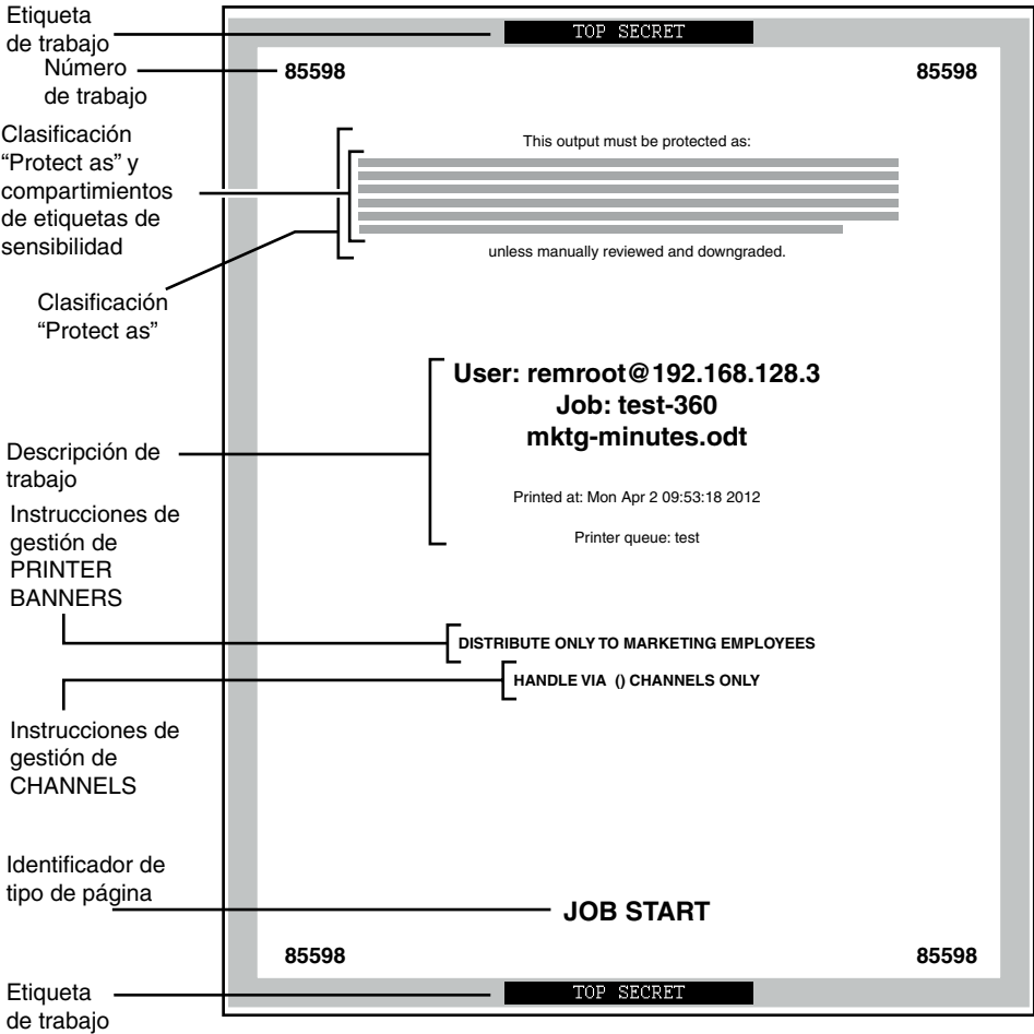
FIGURA 19-1 Página de carátula típica de un trabajo de impresión con etiquetas
