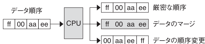
図 A-2 データ順序のホストバス依存性
