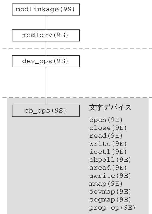
図 15-1 文字ドライバのロードマップ
