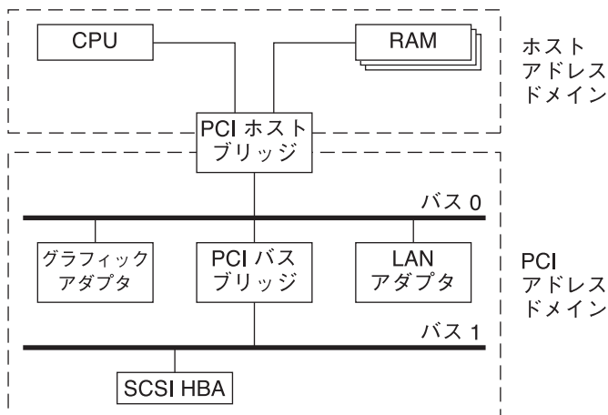
図 A-3 マシンのブロック図
