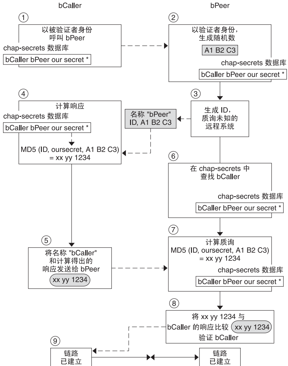
图 8-2 CHAP 验证顺序
