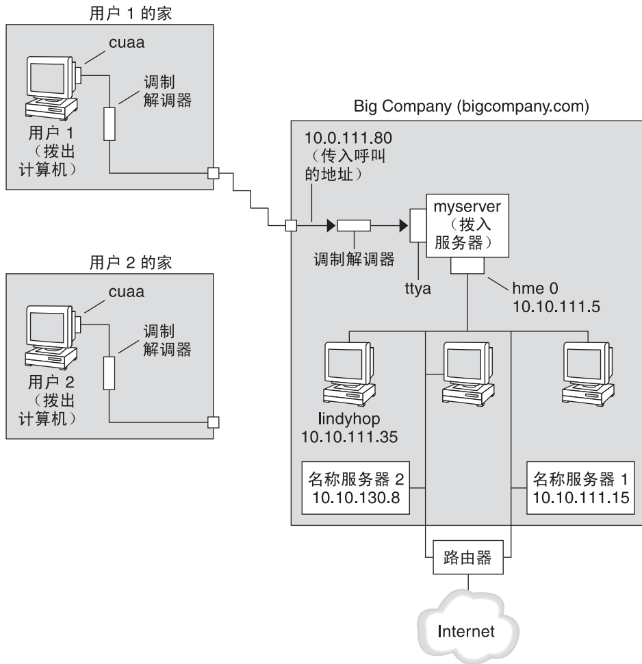
图 2-1 拨号链路样例
