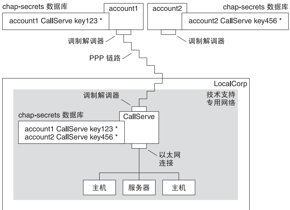
图 2-4 CHAP 验证方案示例（呼叫专用网络）
