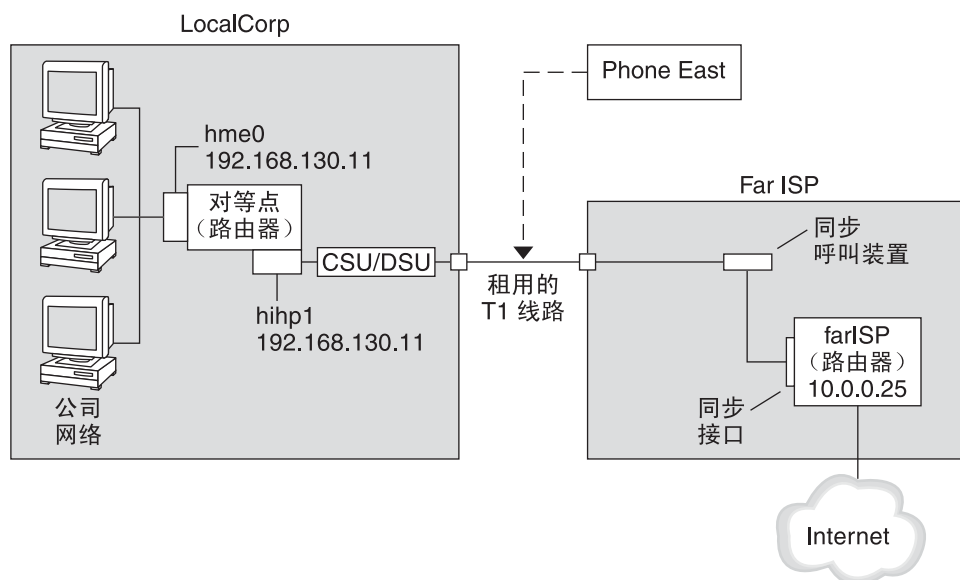
图 2-2 租用线路配置示例
