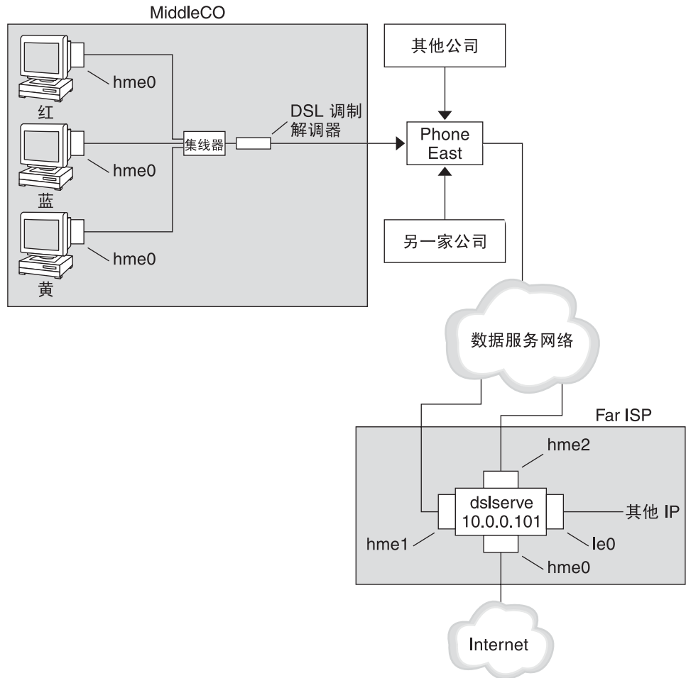
图 2-5 PPPoE 隧道示例
