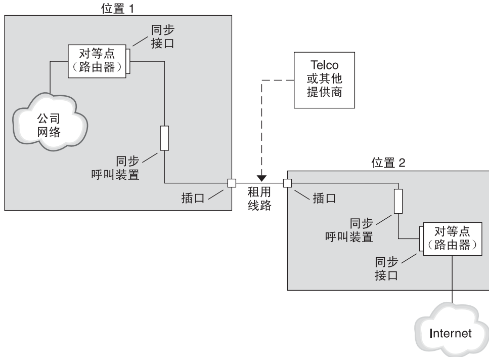
图 1-3 基本租用线路配置
