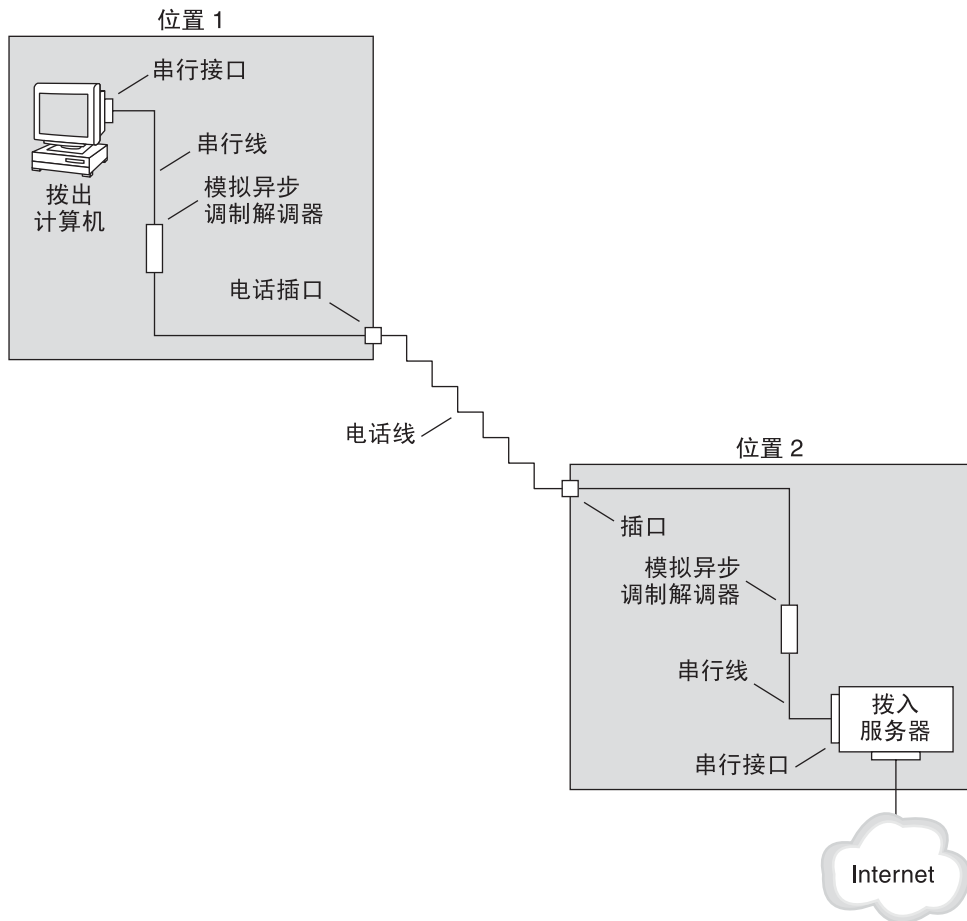
图 1-2 基本模拟拨号 PPP 链路
