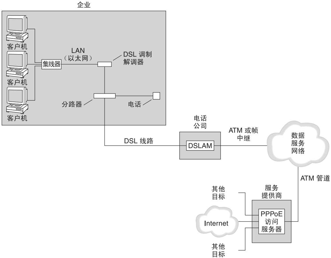
图 1-4 PPPoE 隧道中的参与者
