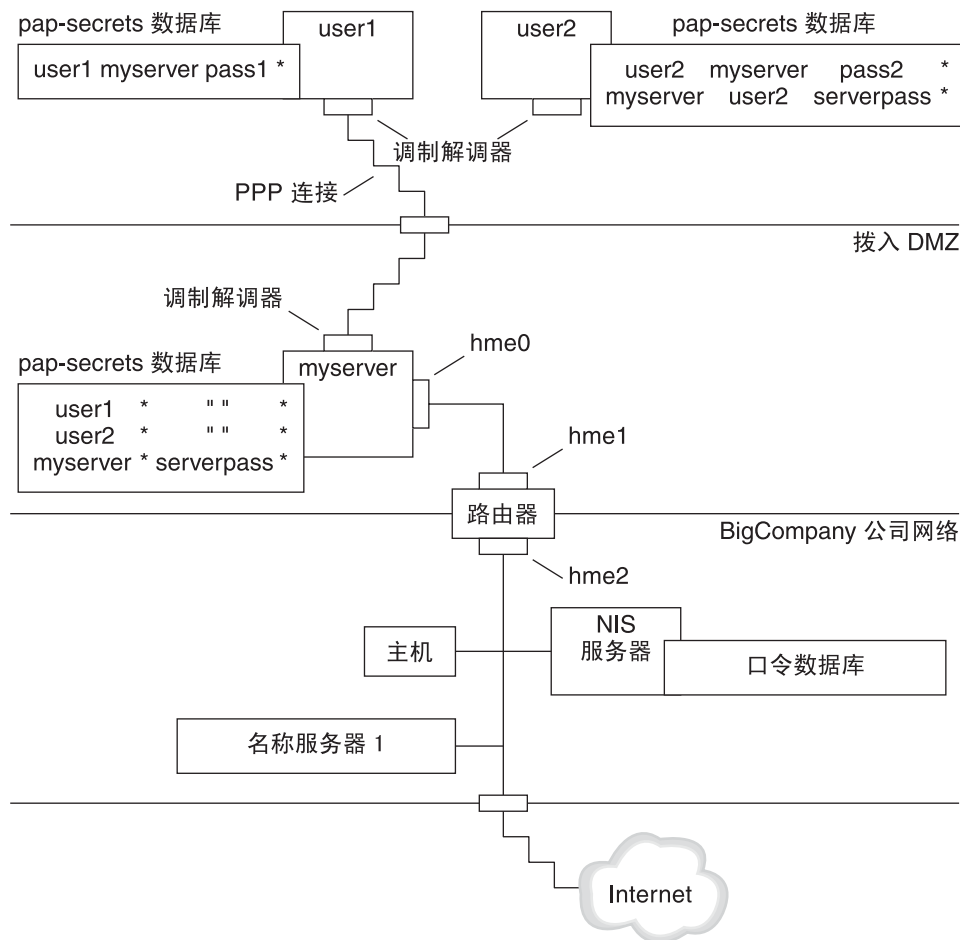
图 2-3 PAP 验证方案示例（在家工作）
