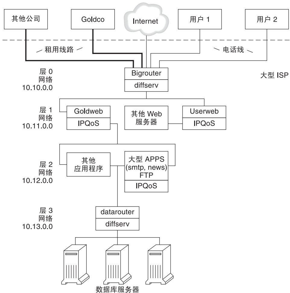
图 2-4 IPQoS 拓扑示例
