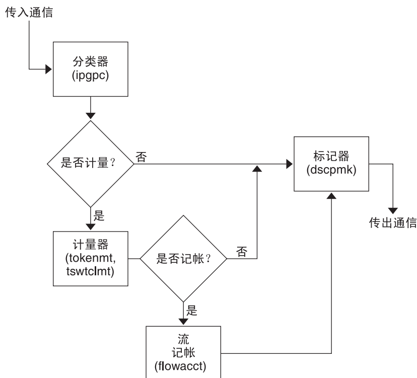
图 1-1 通信流经过 Diffserv 模型的 IPQoS 实现
