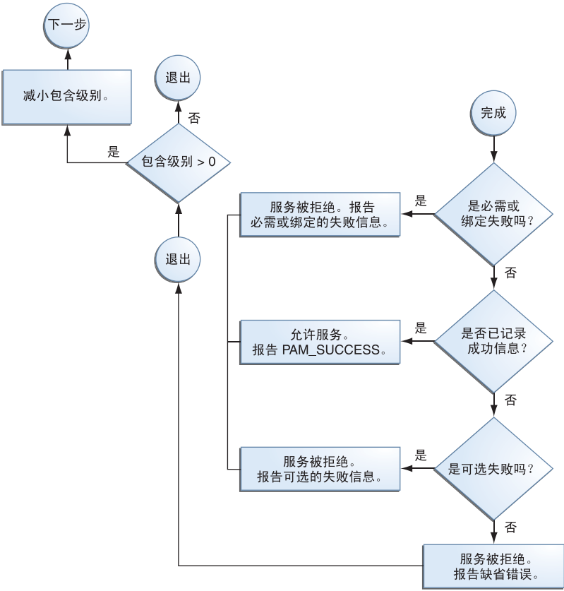
图 14-3 PAM 栈：如何确定集成值
