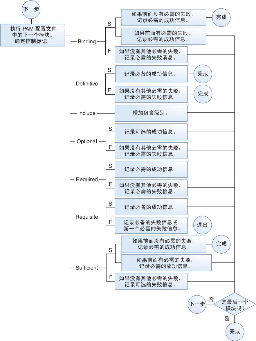
图 14-2 PAM 栈：控制标志的作用
