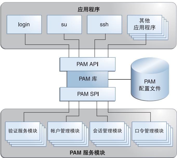
图 14-1 PAM 体系结构
