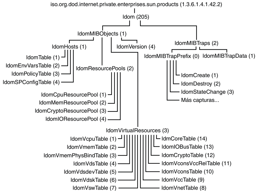
FIGURA 16-2 Árbol de la MIB de Oracle VM Server for SPARC
