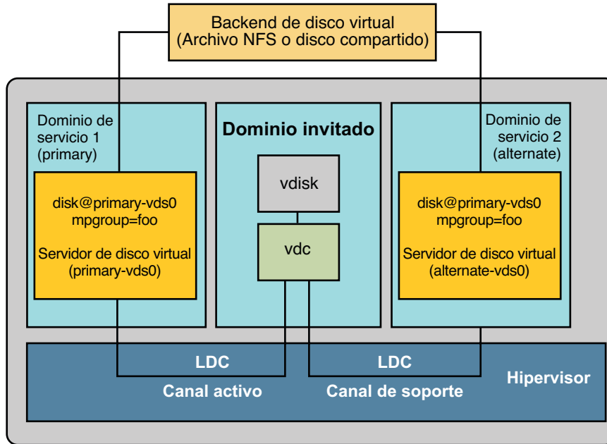
FIGURA 7-2 Configuración de ruta múltiple de disco virtual
