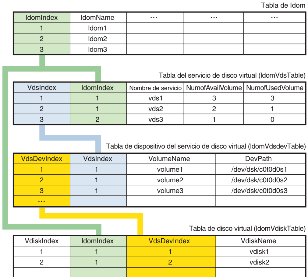
FIGURA 16-3 Relación entre las tablas de discos virtuales y la tabla de dominio
