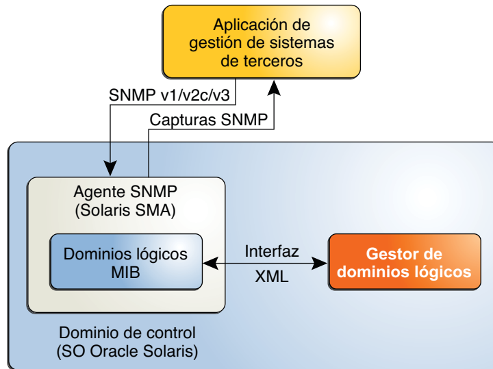
FIGURA 16-1 Interacción de la MIB de Oracle VM Server for SPARC con el agente SNMP de Oracle Solaris, Logical Domains Manager y una aplicación de gestión de sistemas de otro proveedor
