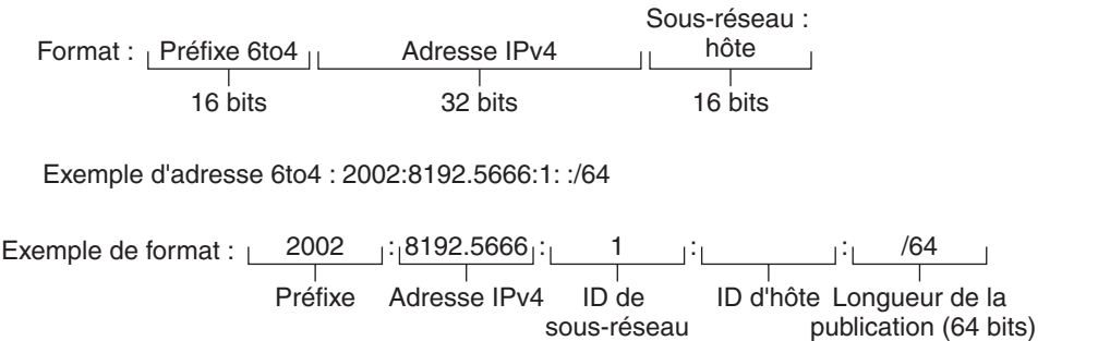
FIGURE 11-2 Eléments d'un préfixe de sous-réseau 6to4
