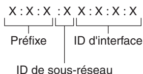
FIGURE 3-2 Format d'adresse IPv6 de base
