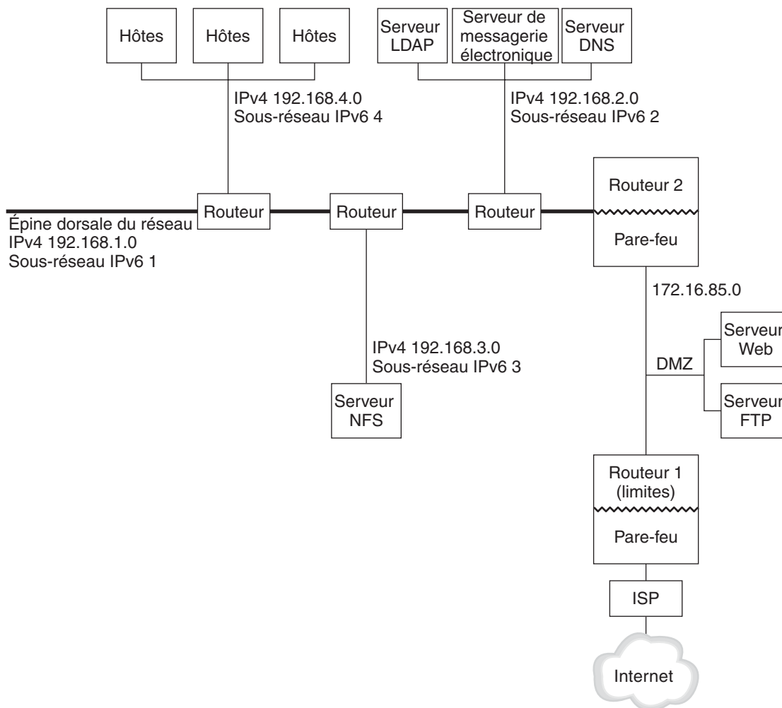
FIGURE 4-1 Scénario de topologie de réseau IPv6
