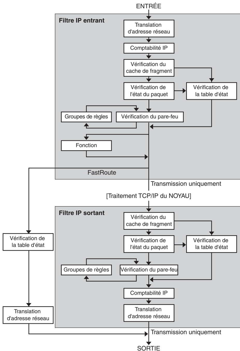
FIGURE 25-1 Séquence de traitement d'un paquet
