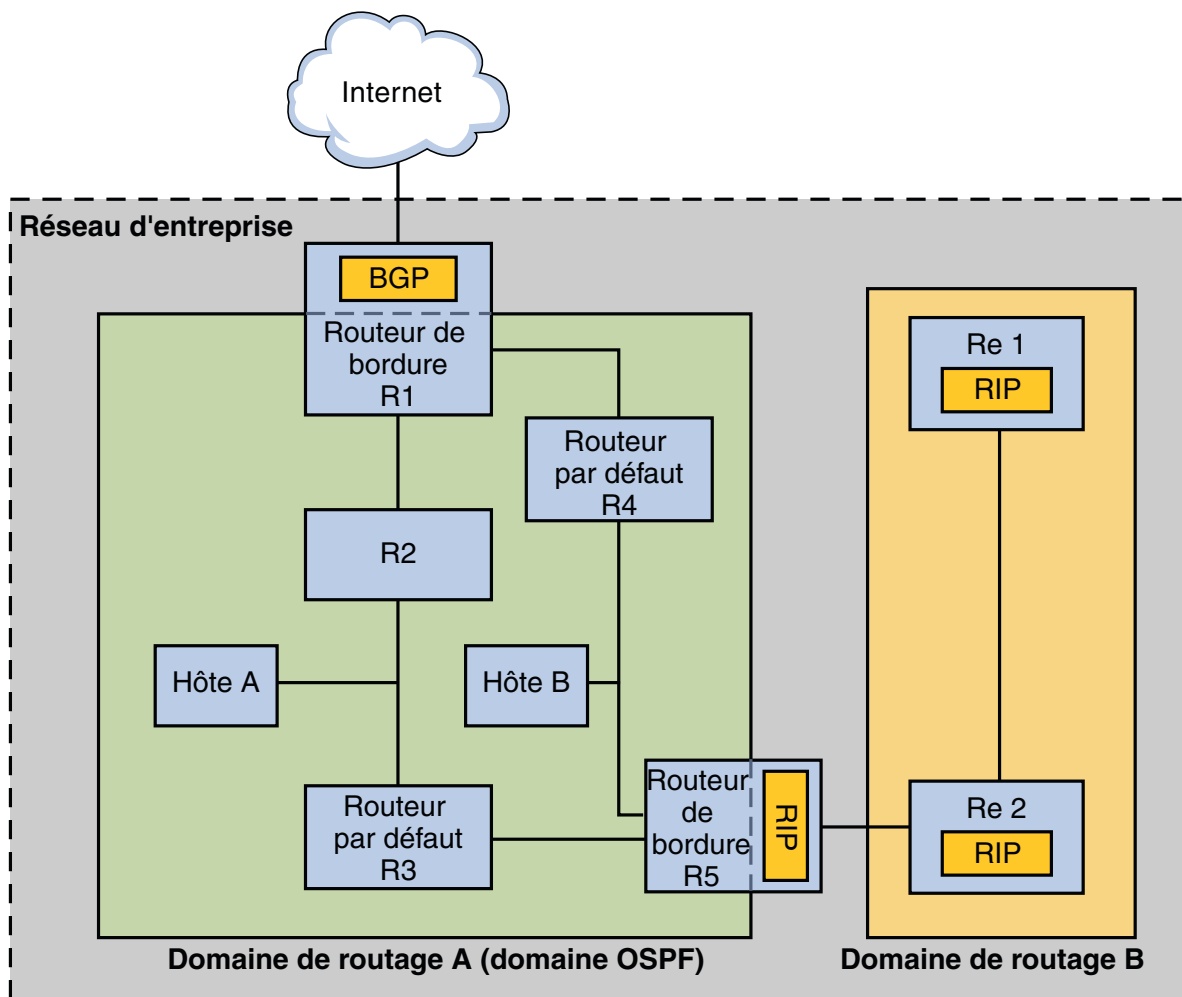
FIGURE 5-2 Réseau d'entreprise exécutant les protocoles Quagga
