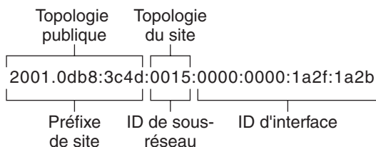
FIGURE 3-3 Parties de l'adresse unicast globale
