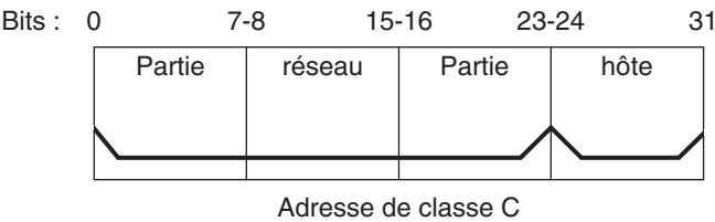
FIGURE 10-5 Allocation des octets dans une adresse de classe C
