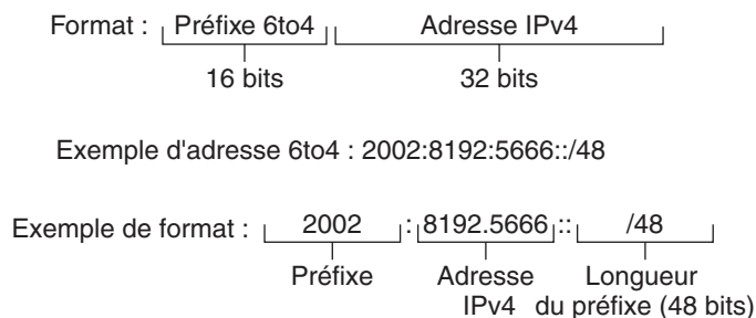
FIGURE 11-1 Eléments d'un préfixe de site 6to4
