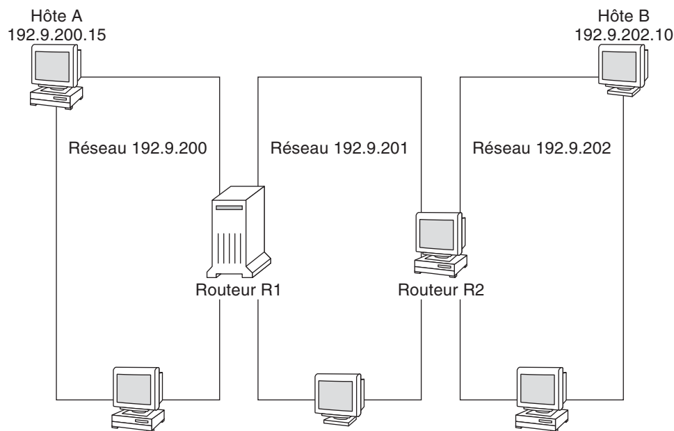
FIGURE 2-5 Topologie réseau correspondant à trois réseaux interconnectés
