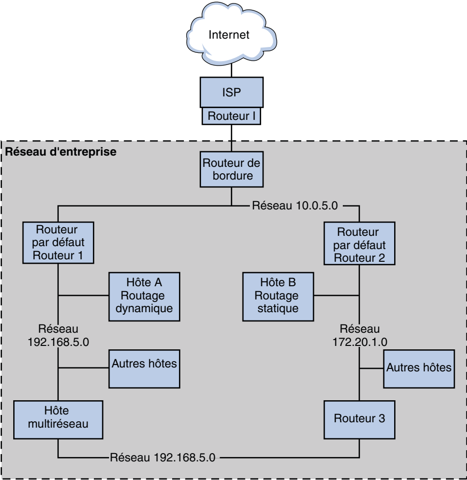
FIGURE 5-3 Système autonome comportant plusieurs routeurs IPv4
