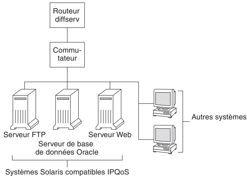
FIGURE 30-1 Systèmes IPQoS sur un segment de réseau
