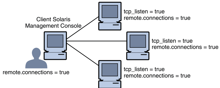
FIGURE 2-6 Client de Solaris Management Console administrant des systèmes distants individuels sur un réseau
