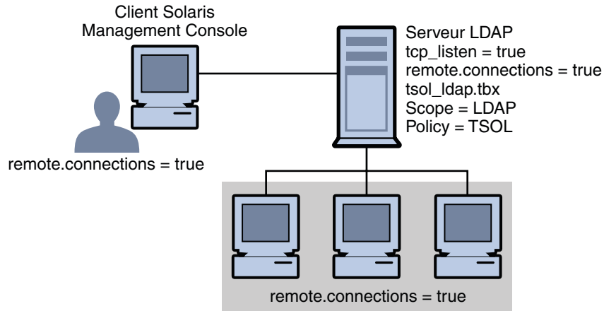
FIGURE 2-5 Client de Solaris Management Console utilisant un serveur LDAP pour administrer le réseau
