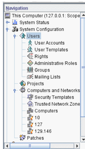
FIGURE 2-4 Ensemble d'outils Computers and Networks (Ordinateurs et réseaux) dans Solaris Management Console
