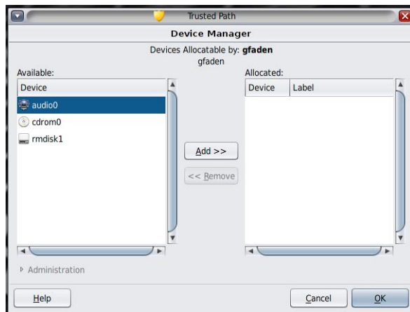
FIGURE 16-1 Gestionnaire d'allocation de périphériques ouvert par un utilisateur
