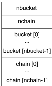
图 12-4 符号散列表
