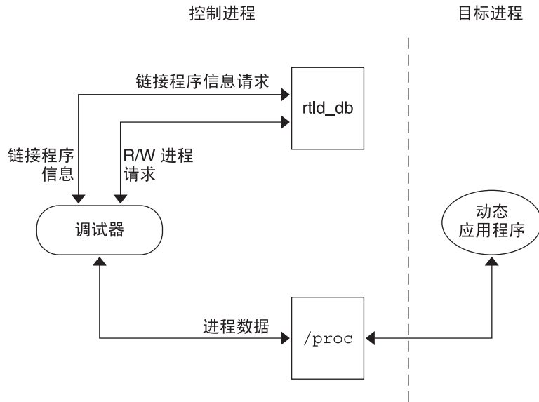
图 11-1 rtdl-debugger 信息流
