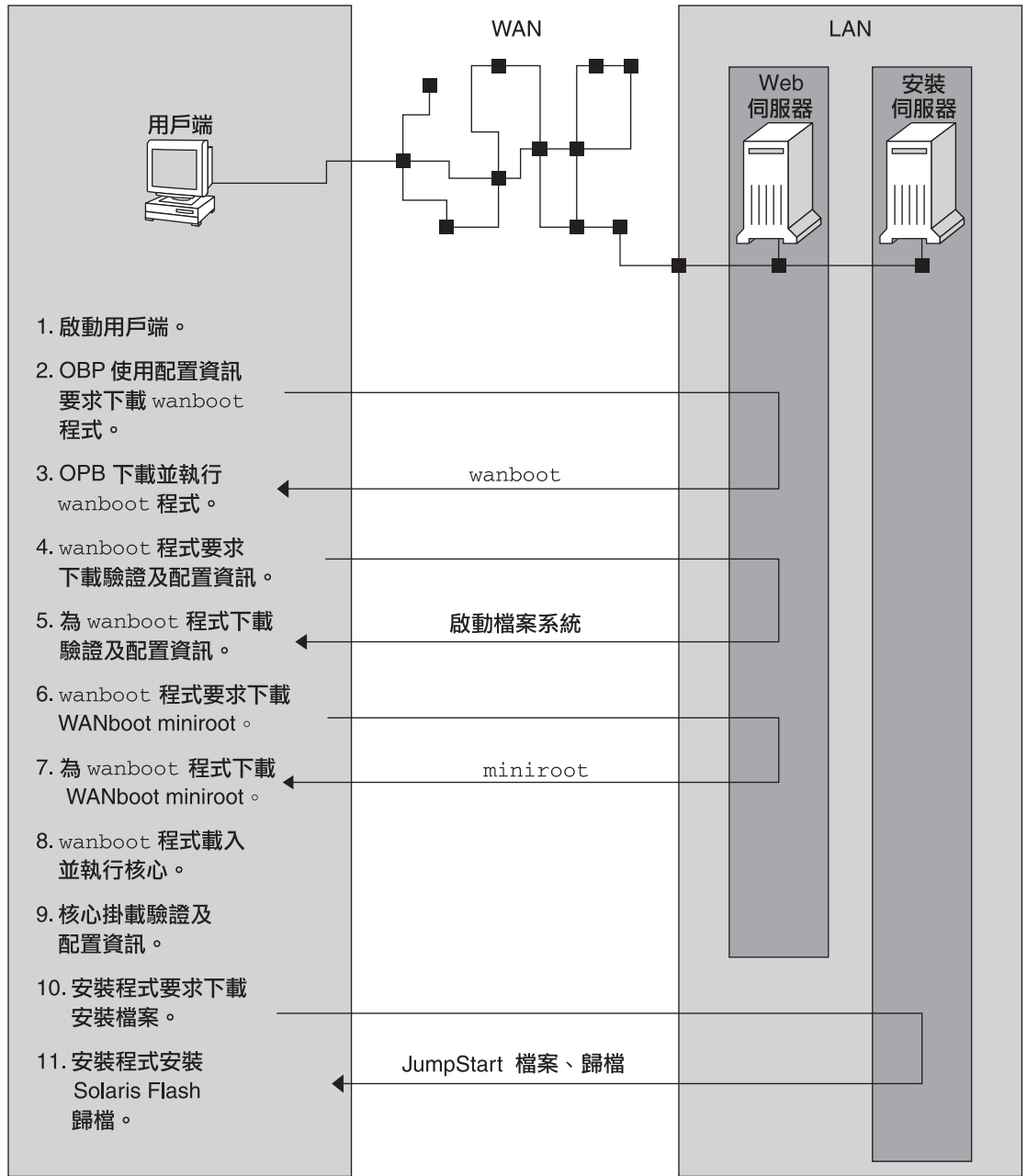
圖 10-1 WAN Boot 安裝中的事件序列
