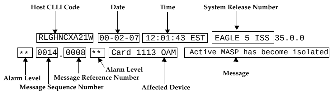
Figure 3-6. Output Message Format
