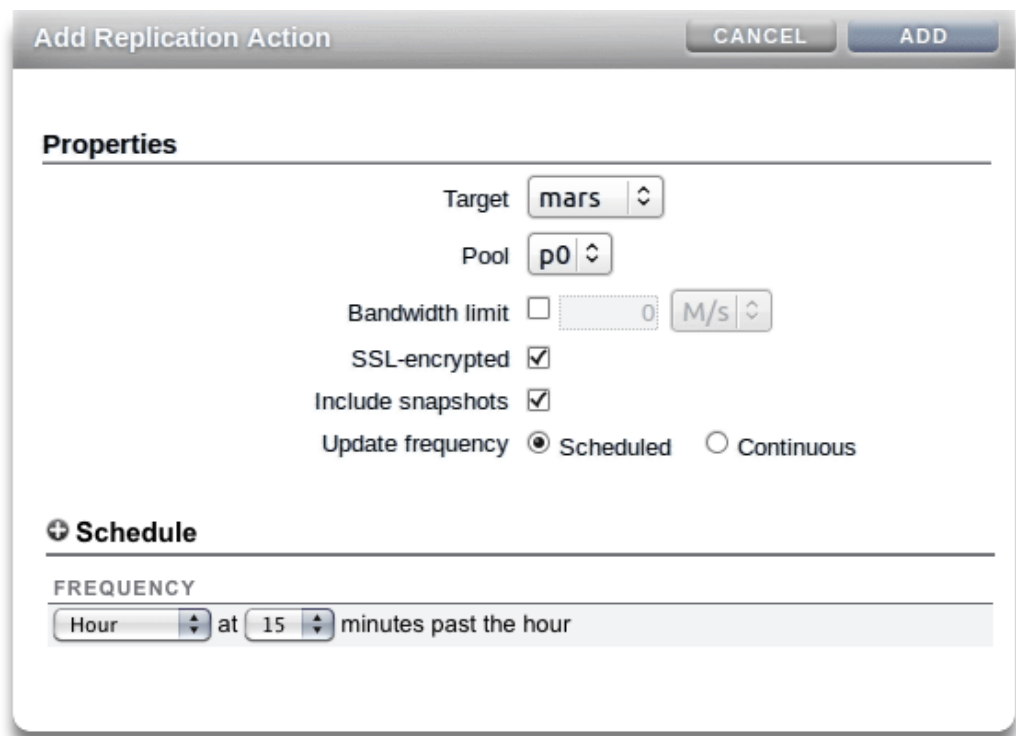
图 44 添加复制操作
