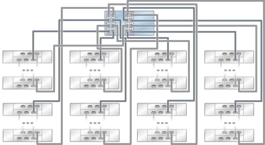
图 28 单个链中的多个磁盘机框
