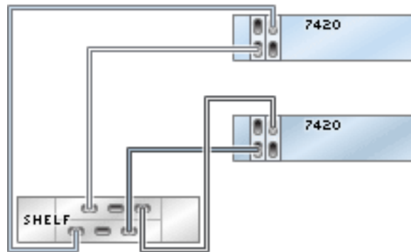
图 167 具有两个 HBA 且通过两个链连接到两个 DE2-24 磁盘机框的群集 7420 控制器
