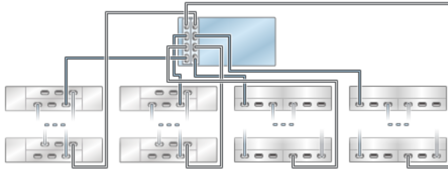
图 351 单个链中的多个 DE2-24 磁盘机框
