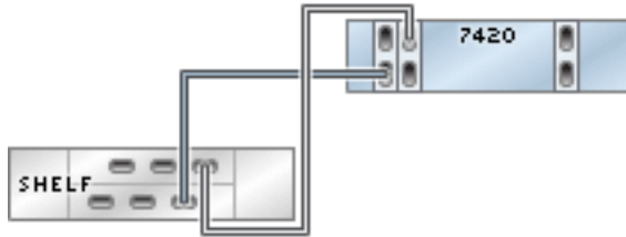
图 137 具有三个 HBA 且通过两个链连接到两个 DE2-24 磁盘机框的单机 7420 控制器
