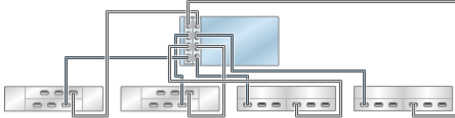
图 350 具有两个 HBA 且通过四个链连接到多个混合磁盘机框的单机 7420 控制器 (DE2-24 显示在左侧)
