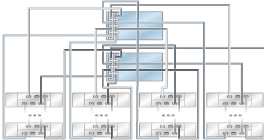
图 34 单个链中的多个磁盘机框
