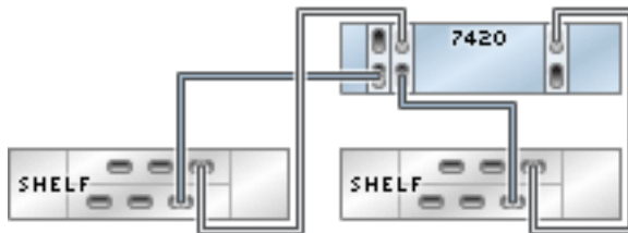
图 138 具有三个 HBA 且通过三个链连接到三个 DE2-24 磁盘机框的单机 7420 控制器
