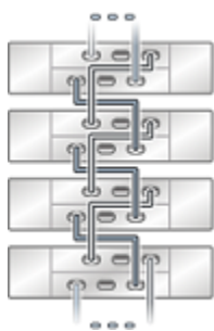
图 10 单个链中的多个磁盘机框
