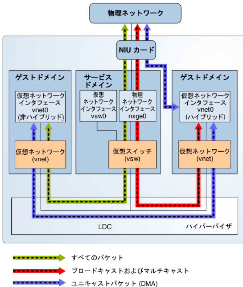
図 12-14 ハイブリッド仮想ネットワーク接続 (Oracle Solaris 10)
