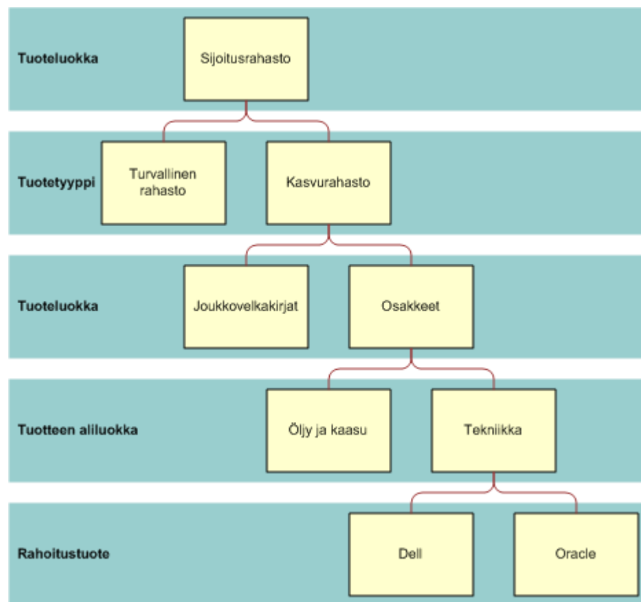
Figure 4: Sijoitusrahaston hierarkiaesimerkki
