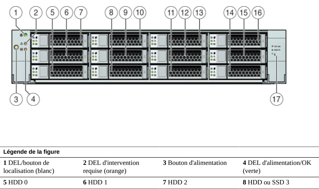
FIGURE 31 Panneau avant du contrôleur 7120
