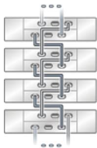
图 370 单个链中的多个 Sun Disk Shelf
