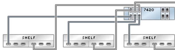
图 229 具有五个 HBA 且通过四个链连接到四个 Sun Disk Shelf 的单机 7420 控制器
