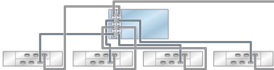
图 9 具有两个 HBA 且通过四个链连接到多个 DE2-24 磁盘机框的单机 ZS4-4/ZS3-4 控制器
