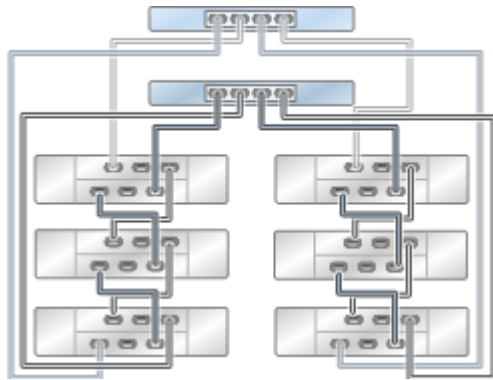
图 67 单个链中的多个磁盘机框
