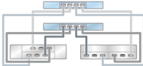
图 338 具有一个 HBA 且通过两个链连接到多个混合磁盘机框的群集 ZS3-2 控制器 (DE2-24 显示在左侧)
