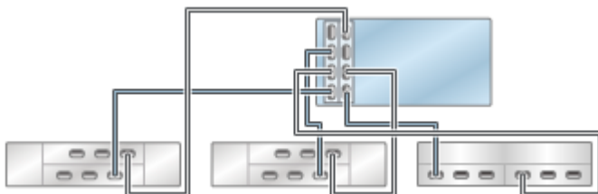
图 281 具有两个 HBA 且通过四个链连接到四个混合磁盘机框的单机 ZS3-4 控制器 (DE2-24 显示在左侧)
