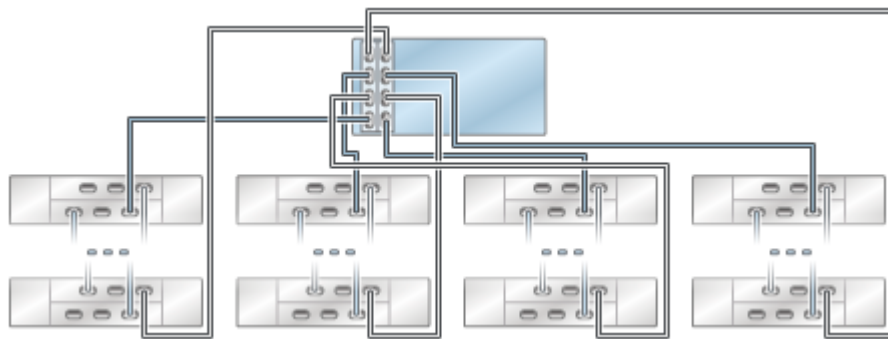
图 10 单个链中的多个磁盘机框
