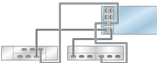
图 280 具有两个 HBA 且通过三个链连接到三个混合磁盘机框的单机 ZS3-4 控制器 (DE2-24 显示在左侧)
