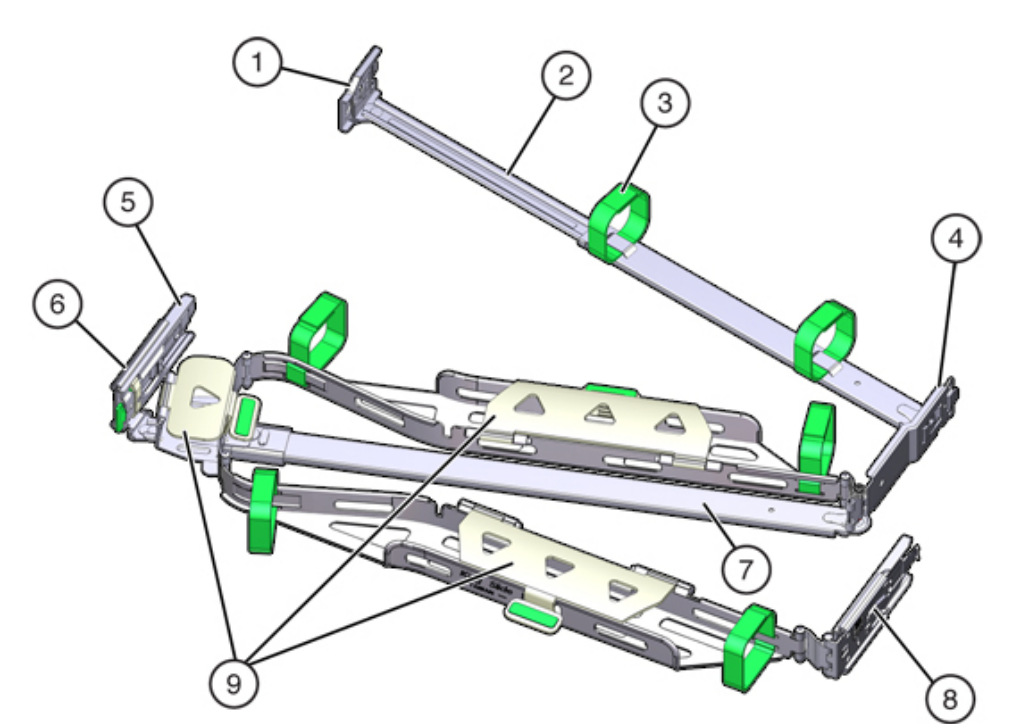
图 35 ZS3-2 控制器的可选理线架
