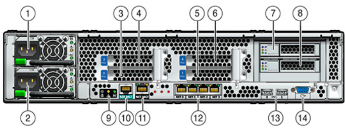
図 66 7120 コントローラの背面パネル
