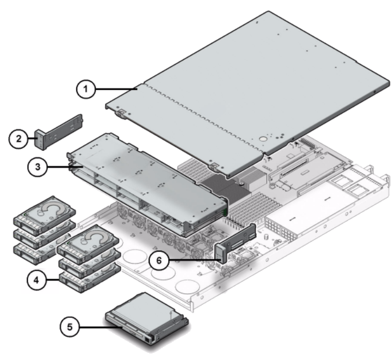
図 64 7320 コントローラの I/O コンポーネント
