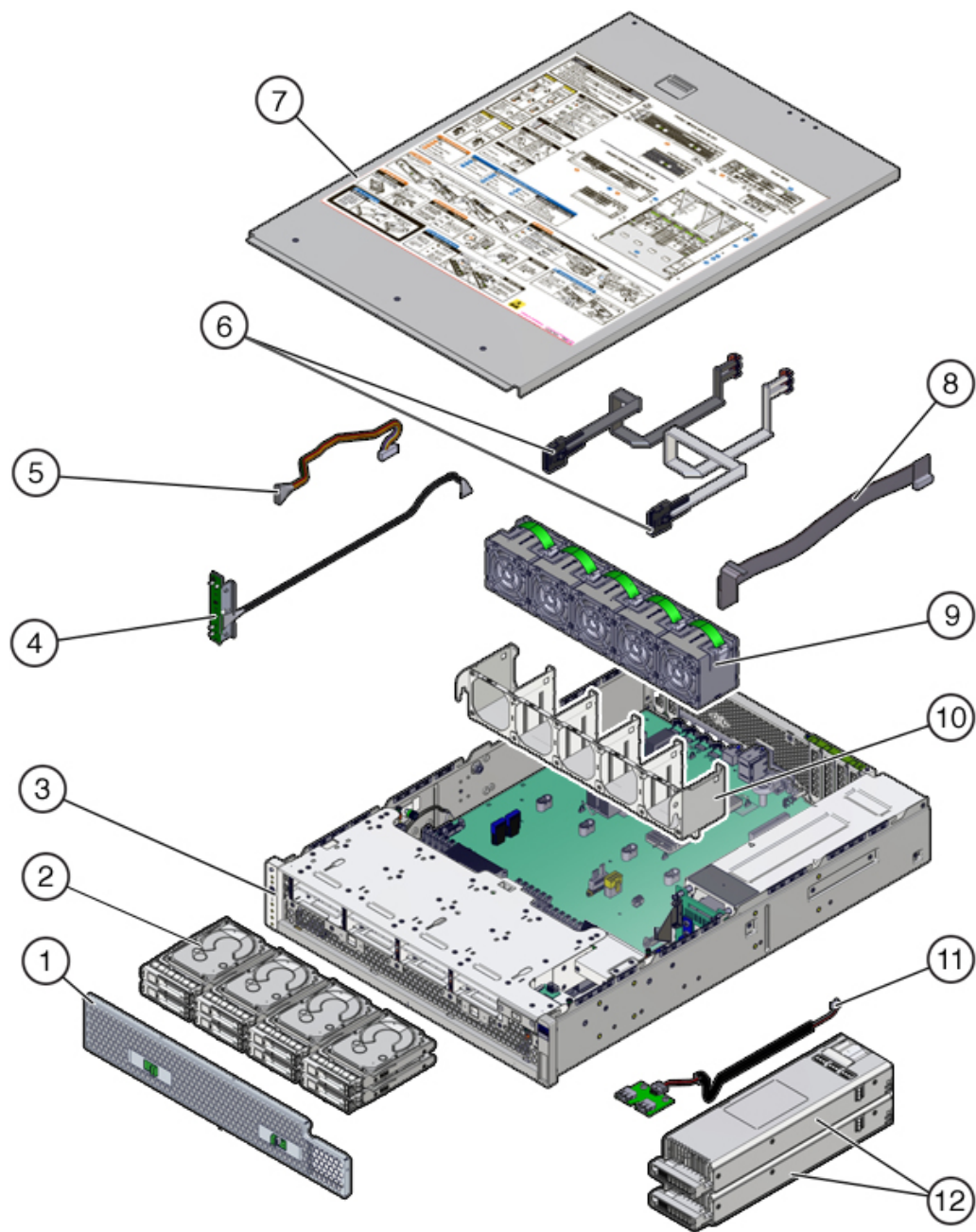
図 9 ZS5-2 のストレージ、電源、およびファンモジュール
