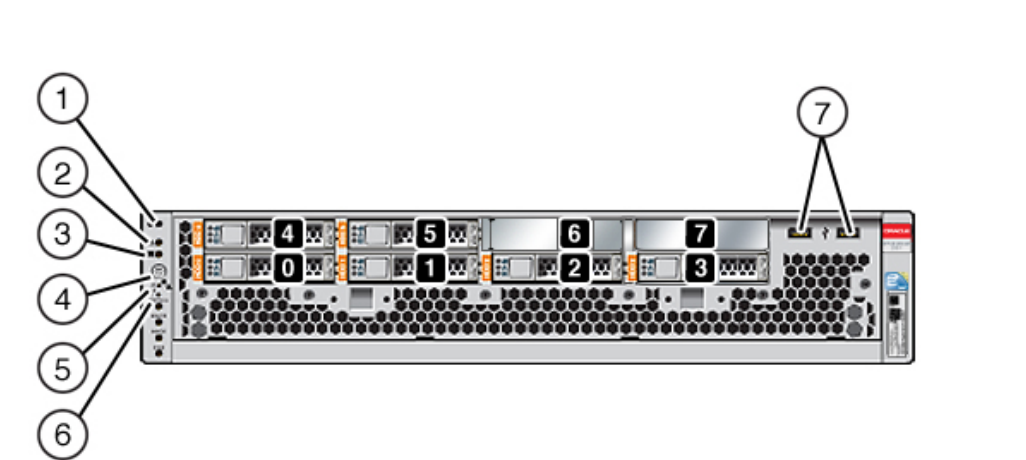
図 35 ZS3-2 コントローラのフロントパネル
